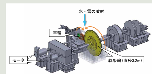
【ブレーキ総合試験装置】
