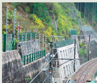
【落石止擁壁と落石警報装置】
