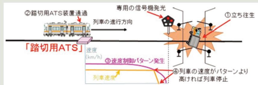
【踏切用ATS装置】
