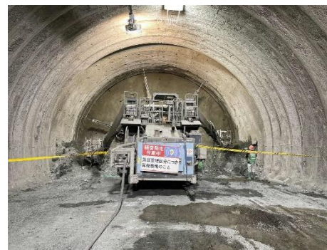
伊那山地トンネル (青木川工区) 本坑掘削工
