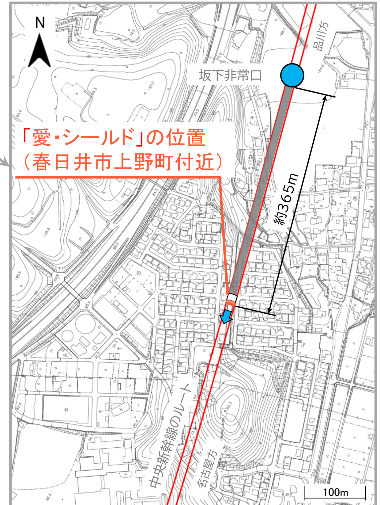
掘進位置周辺の拡大図
