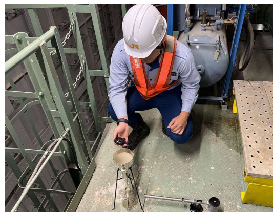
泥水品質の確認状況
