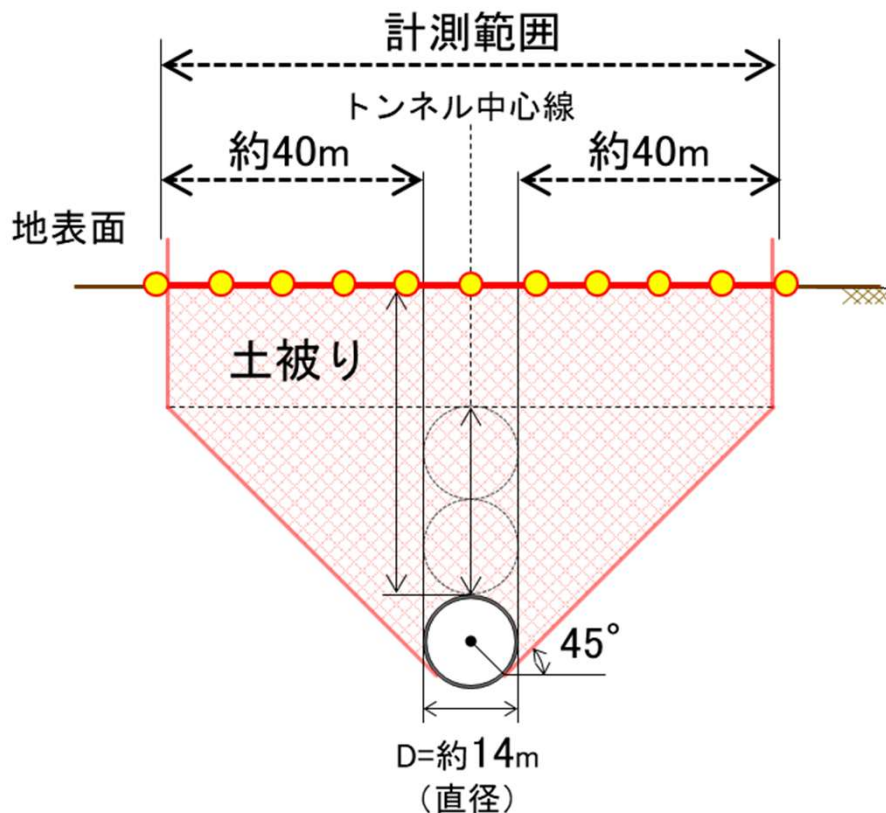
【横断図】
