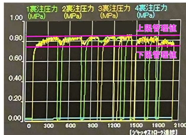
管理モニター（裏込め注入圧）の確認状況
