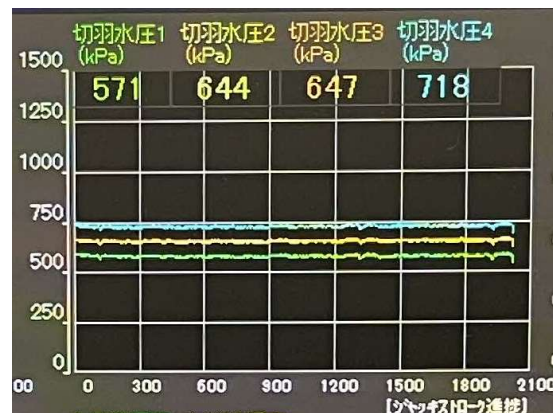
管理モニター（泥水圧）の表示状況
