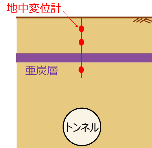
「地中変位計」の設置イメージ
