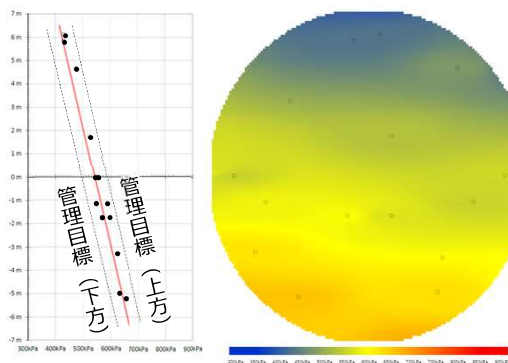
チャンバー内の泥土の圧力勾配
