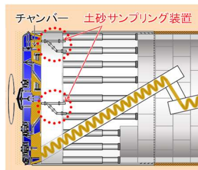
土砂サンプリング装置の設置位置
