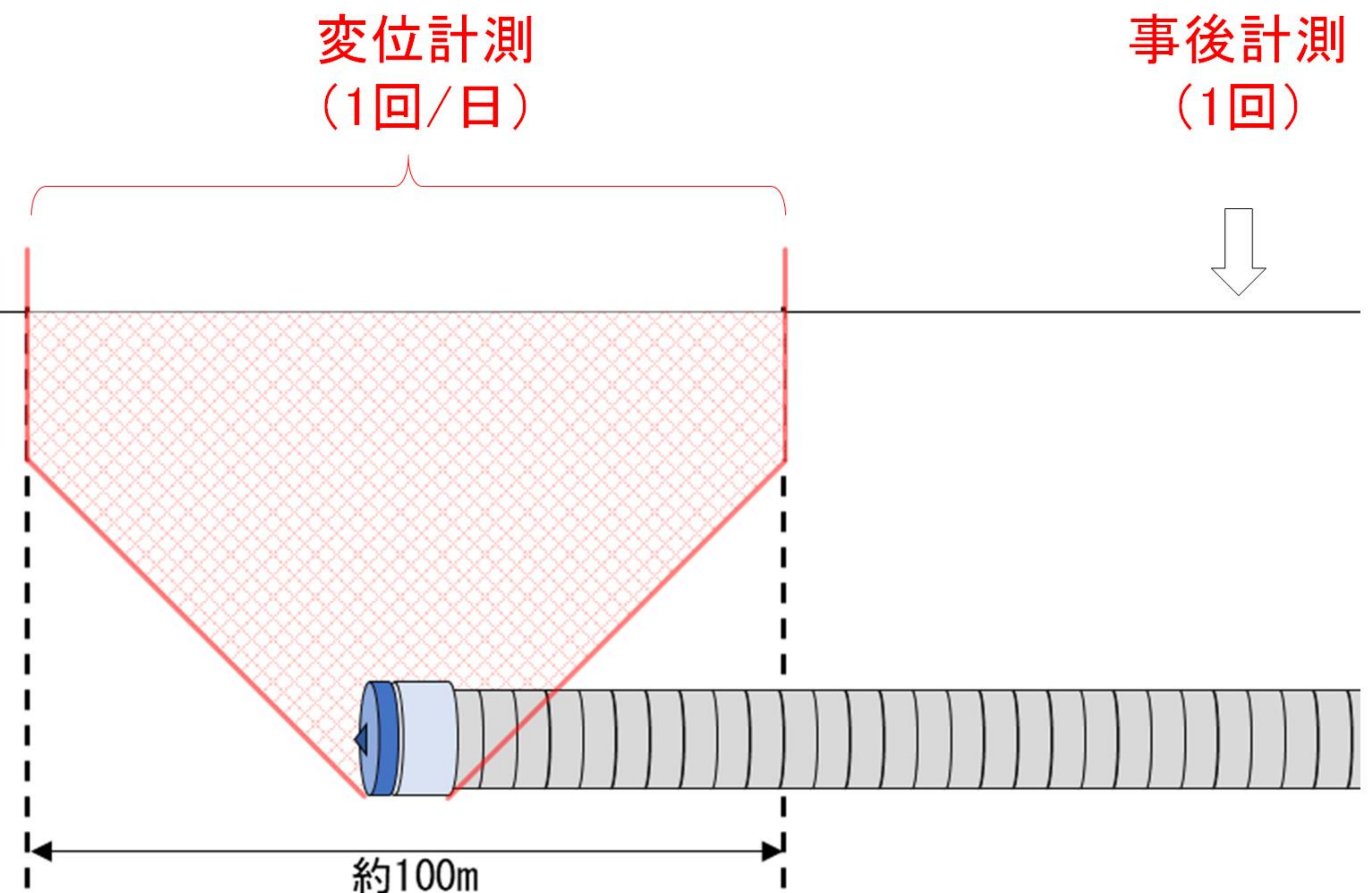
【縦断面図】
