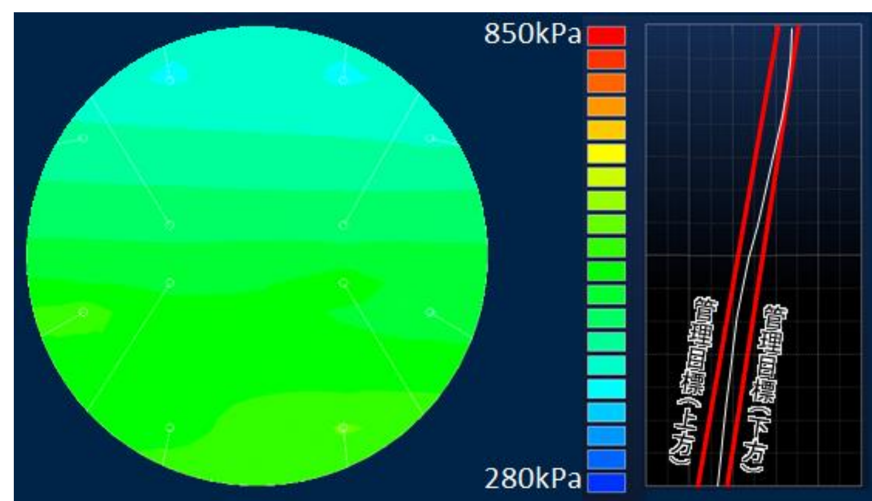
チャンバー内の泥土の圧力勾配
