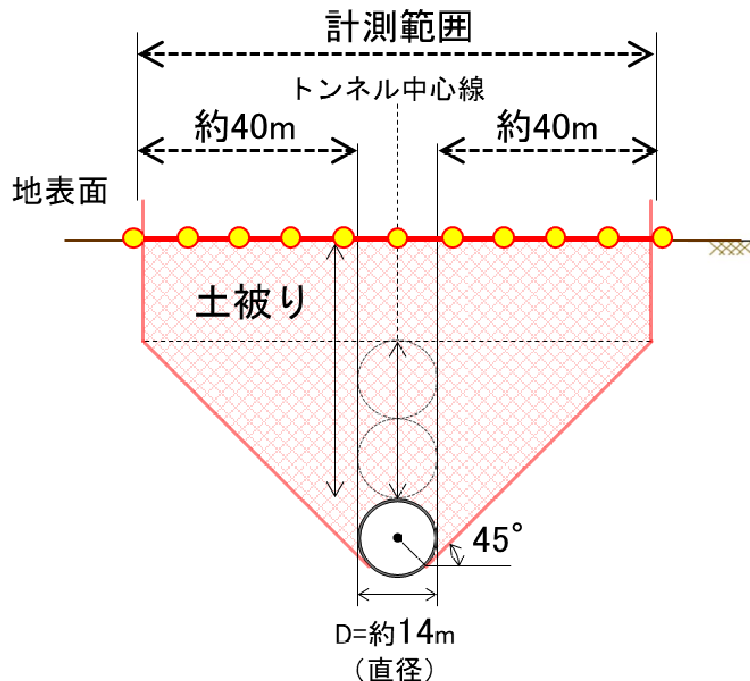
【横断面図】
