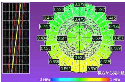
チャンバー内泥土の圧力勾配
