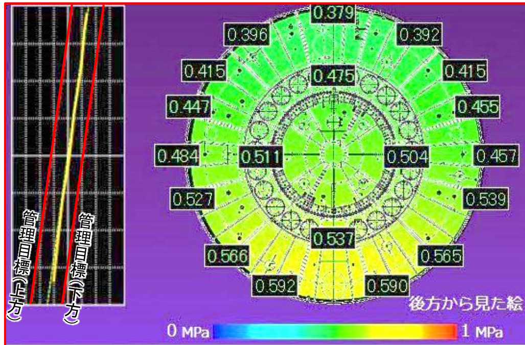
管理モニターの表示状況(掘進距離約100m付近)
