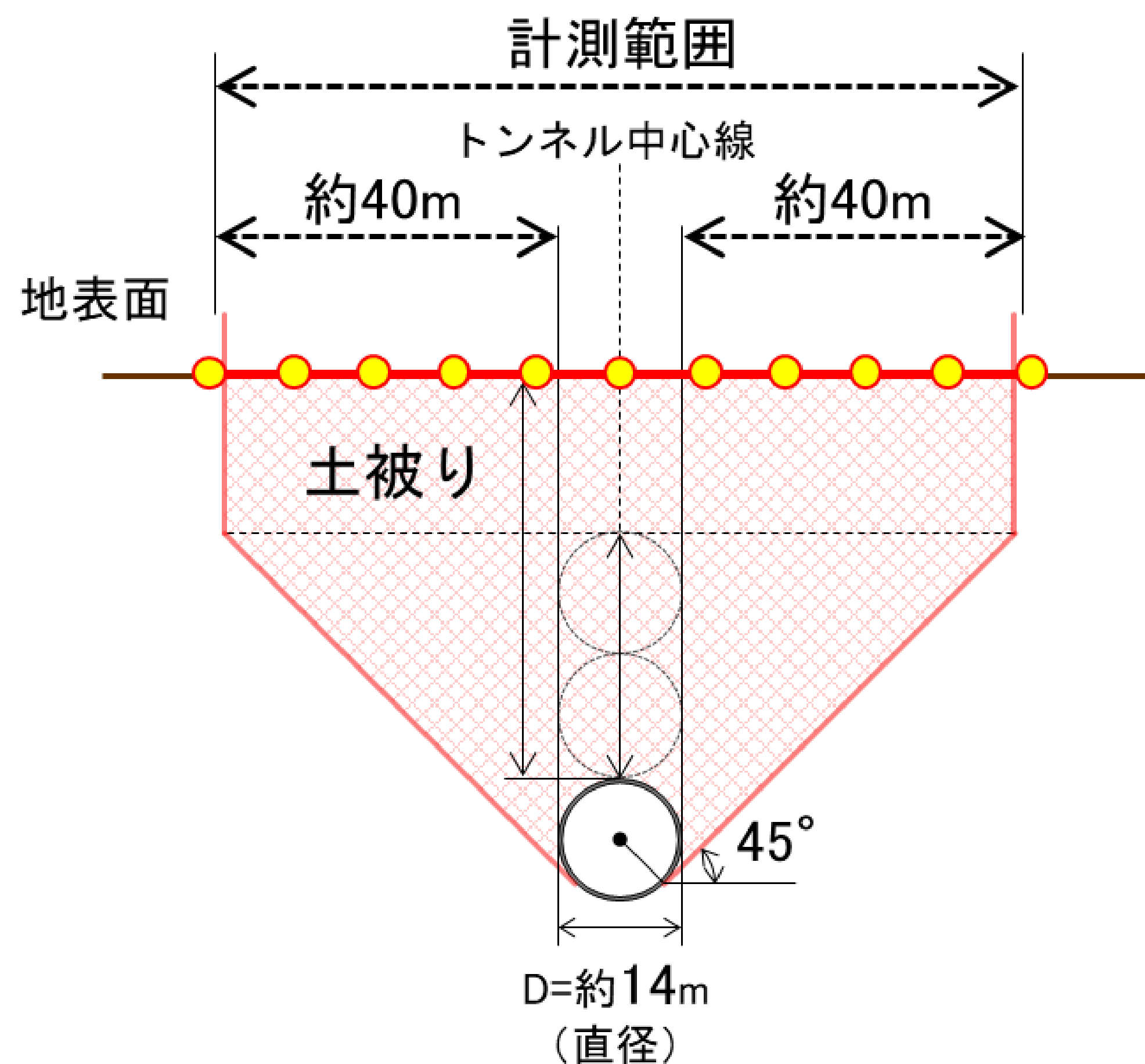
【横断図】
