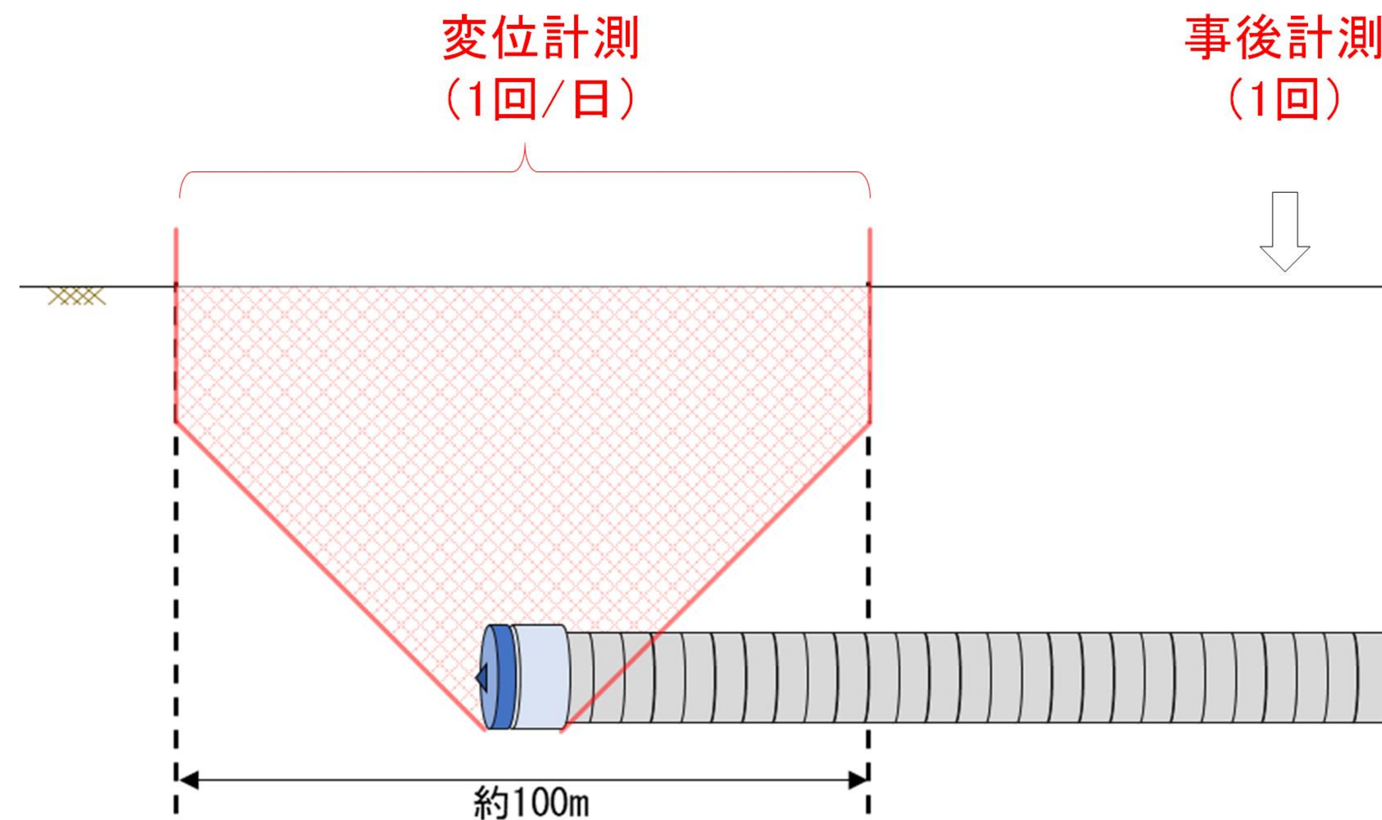
水準測量
