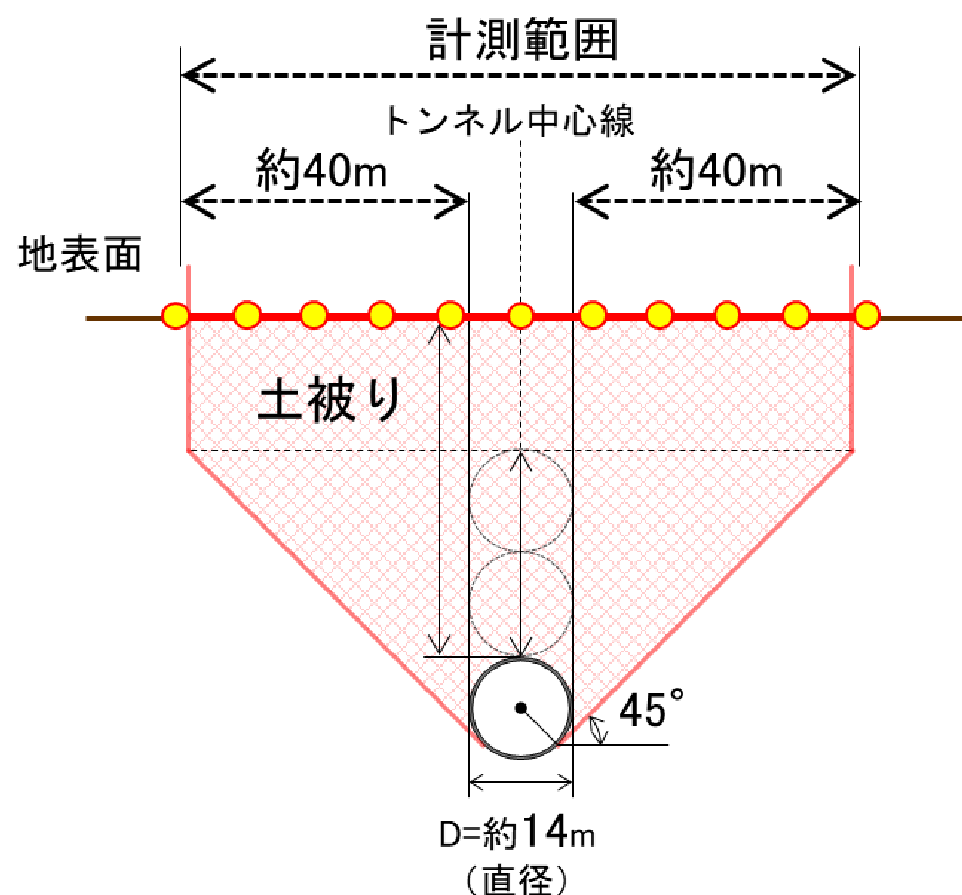
【横断図】
