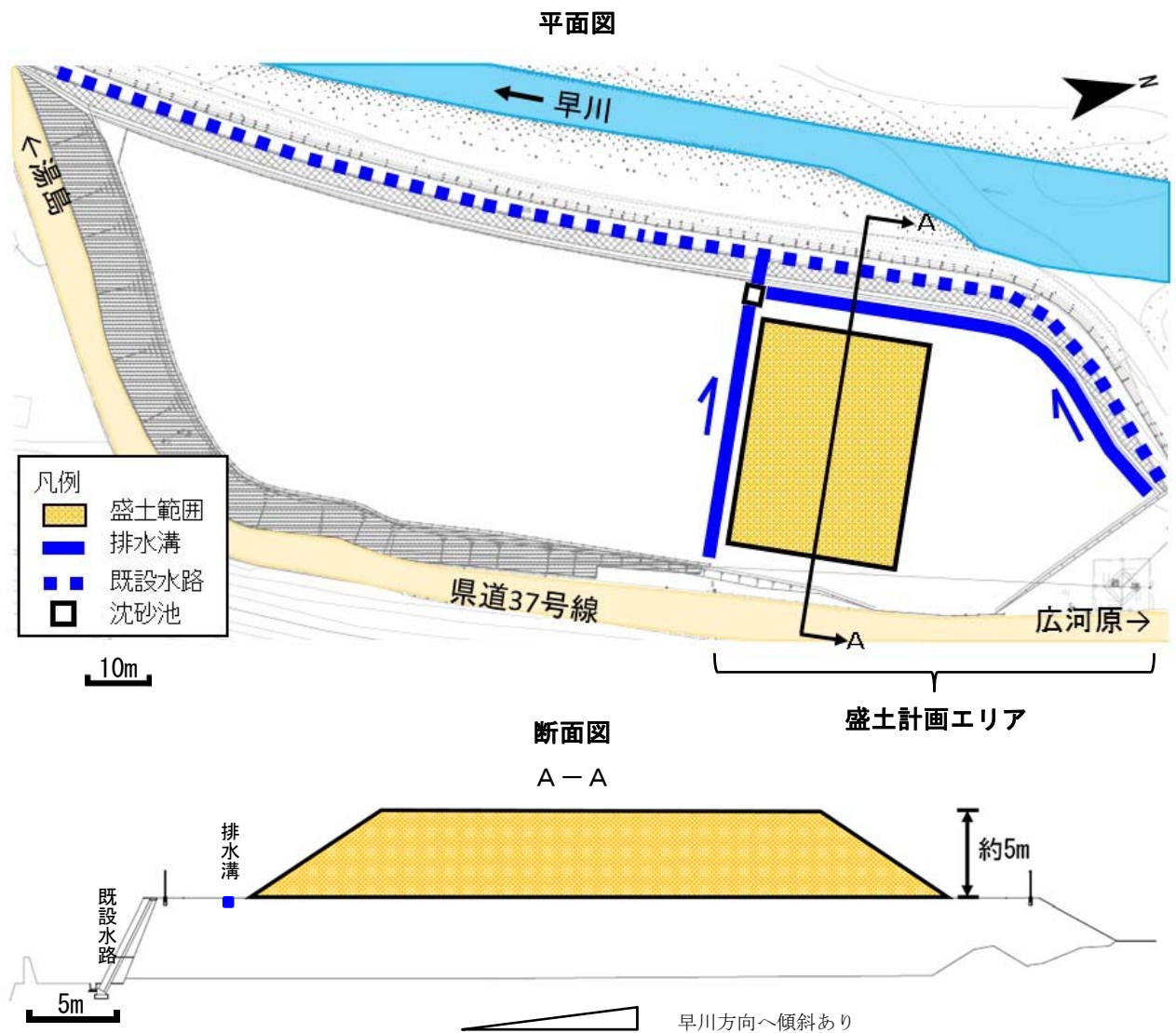
図 2-3 (1) 奈良田地区発生土仮置き場における盛土計画（冬季閉鎖期間）
