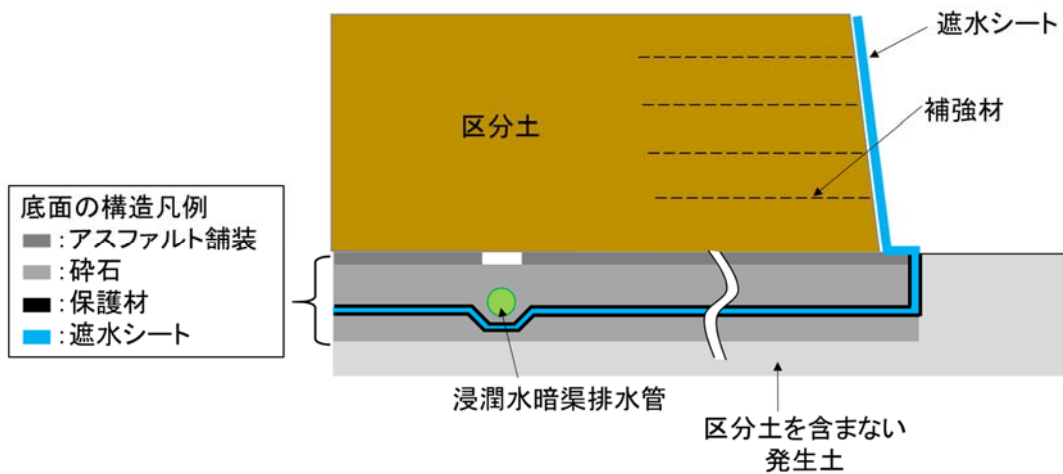
図 2-3(3) 中洲地区（その2）発生土仮置き場計画地における盛土計画
