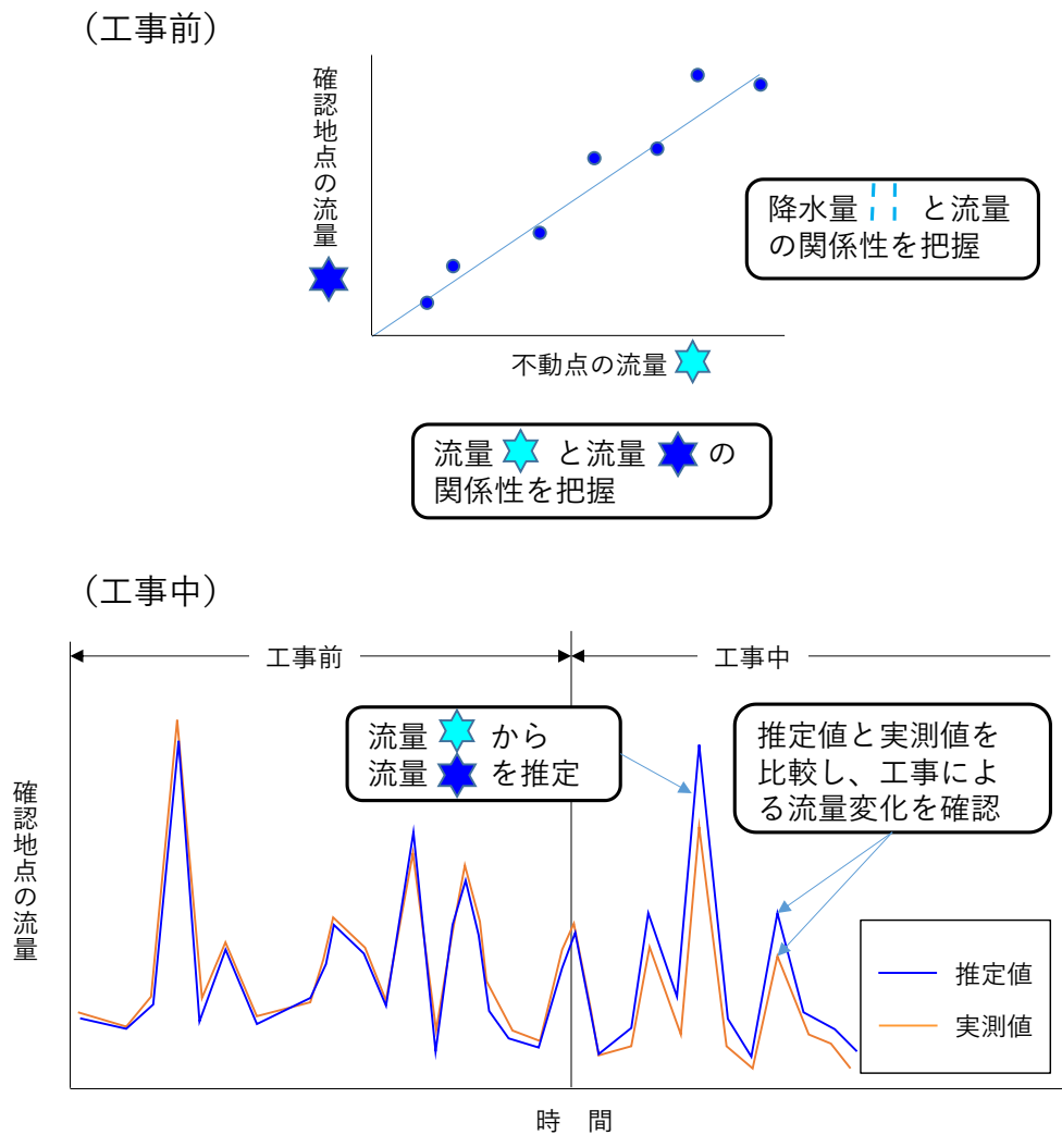
図 5 さわらじま 椹島における流量変化の確認方法 (イメージ)
