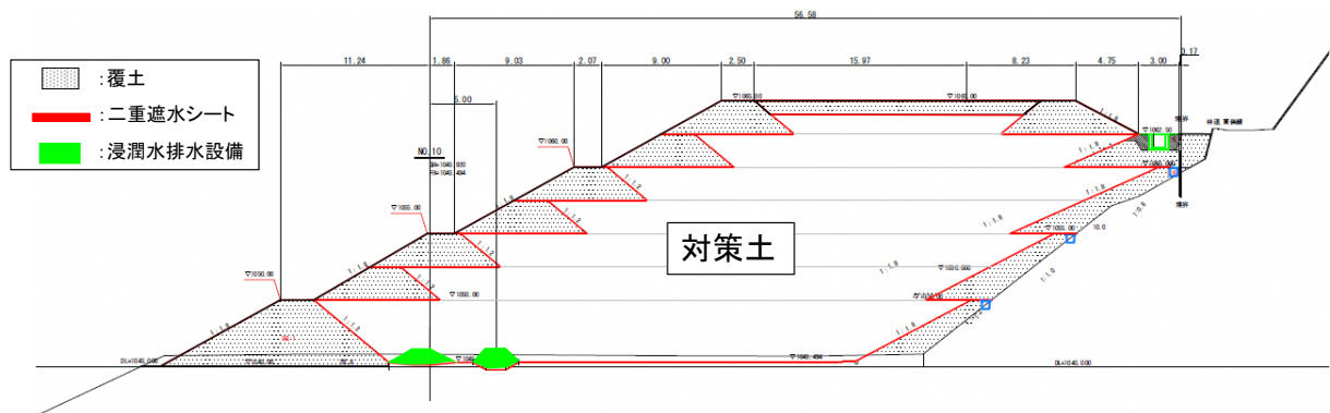
図 12 計画横断図（A－A'断面のうち盛土部）
