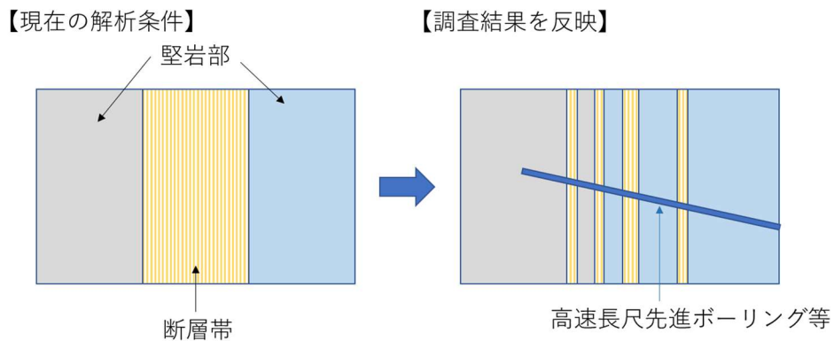
図 17 調査による地盤区分の把握のイメージ
