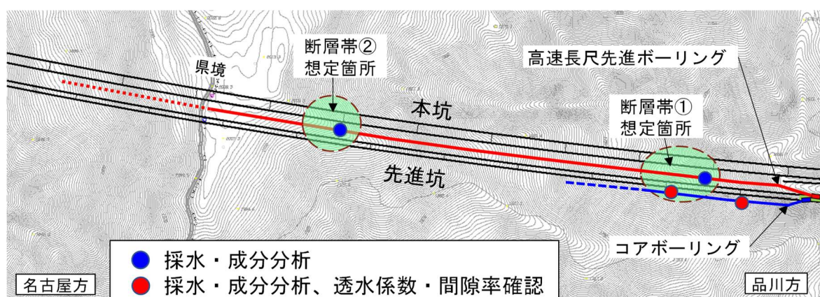
図 5 6 測定地点
