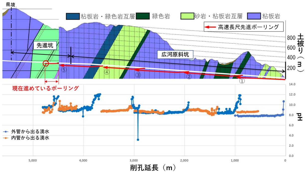
図 59 山梨県内の高速長尺先進ボーリング（広河原斜坑・先進坑）湧水の pH
