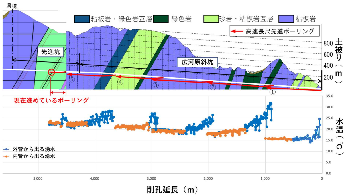
図 5 7 山梨県内の高速長尺先進ボーリング（広河原斜坑・先進坑）湧水の水温
