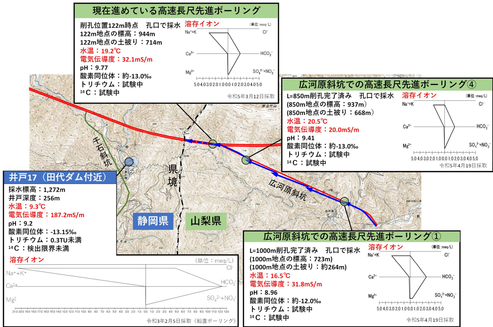
図 6 1 山梨県内の地下水、静岡県内の地下水に関わる水質の測定結果①
