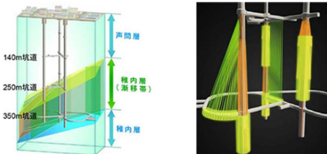
図 1 1-6 幌延深地層研究施設（左図）および薬液注入位置（右図）の概要図
