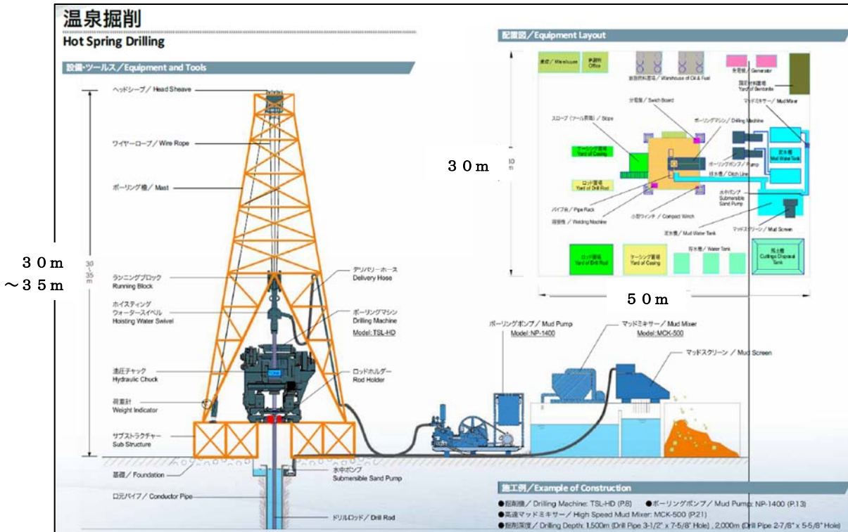
図 8-8 深井戸掘削設備のイメージ
