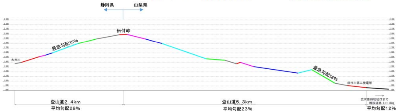
図 8-2 計画縦断面図
