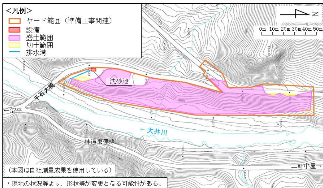
図 1-4(3) 造成・整地（千石Bヤード）
