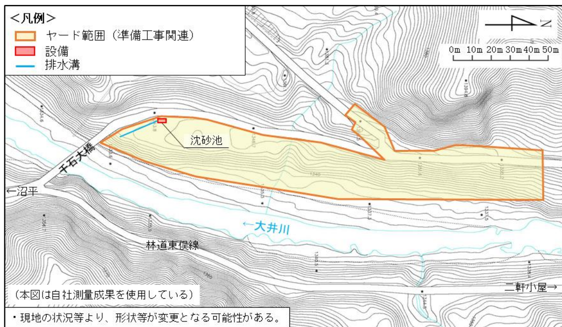
図 1-2(2) ヤード範囲、配置（千石Bヤード）
