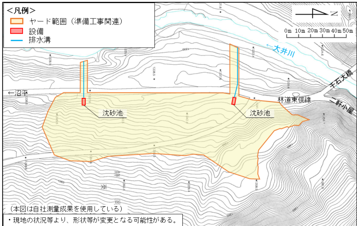
図 1-2(1) ヤード範囲、配置（千石Aヤード）
