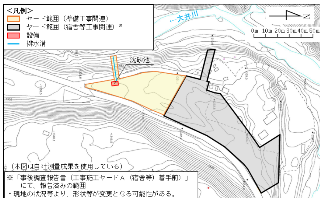
図 1-2(3) ヤード範囲、配置（千石沢ヤード）
