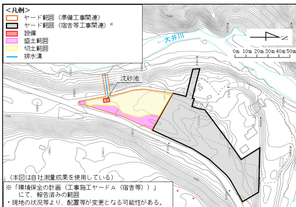
図 1-4(4) 造成・整地（千石沢ヤード）
