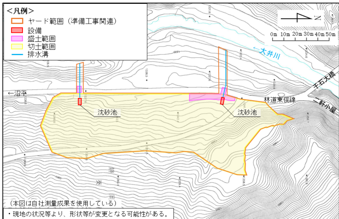
図 1-4(2) 造成・整地（千石Aヤード）
