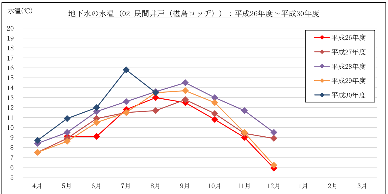
図 3-1-3(2) 地下水の水温計測結果 : 02 民間井戸 (榎島ロッヂ)
