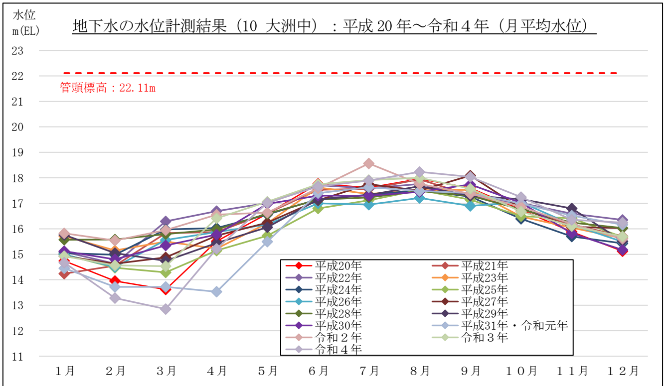
図 3-2-2(19) 地下水の水位計測結果 (月平均水位) : 10 大洲中 (藤枝市弥左工門)
