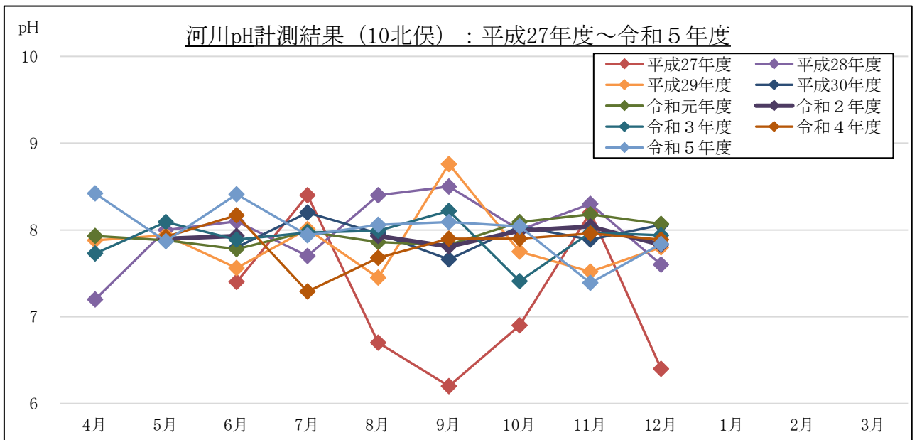
図 2-1-8(6) pH計測結果 (流量 (月1回計測箇所)) : 10 北俣
