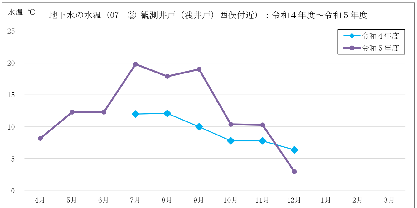
図 3-1-3(10) 地下水の水温計測結果 : 07-② 観測井戸 (浅井戸) 西俣付近
