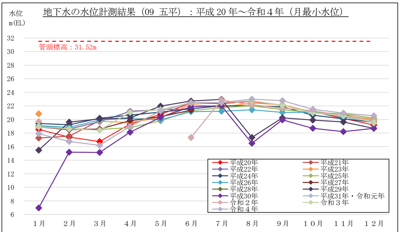
図 3-2-2(18) 地下水の水位計測結果 (月最小水位) : 09 五平 (藤枝市大西町)
