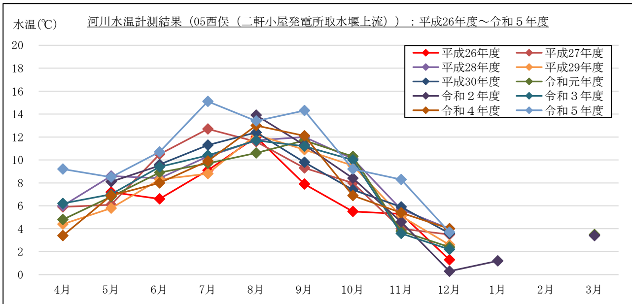
図 2-1-7(1) 水温計測結果 (流量 (月1回計測箇所)) : 05 西俣 (二軒小屋発電所取水堰上流)
