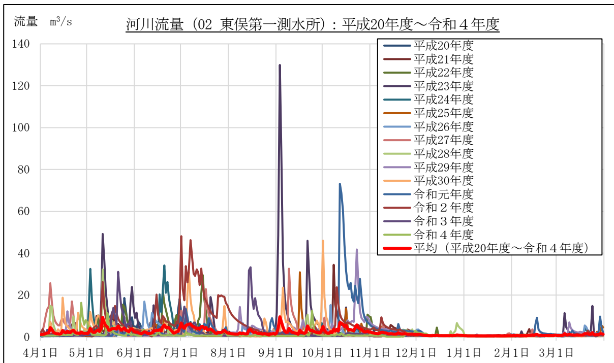
図 2-1-2(2) 流量計測結果 (流量 (常時計測箇所)) : 02 東俣第一測水所
