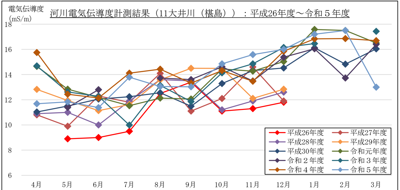
図 2-1-9(7) 電気伝導度計測結果 (流量 (月1回計測箇所)) : 11 大井川 (榎島)
