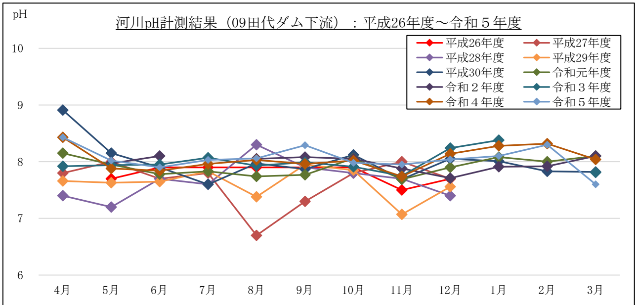
図 2-1-8(5) pH計測結果 (流量 (月1回計測箇所)) : 09 大井川 (田代ダム下流)
