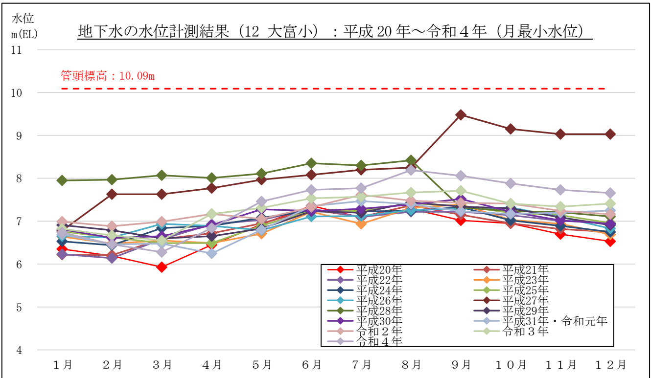
図 3-2-2(24) 地下水の水位計測結果 (月最小水位) : 12 大富小 (烧津市中根新田)
