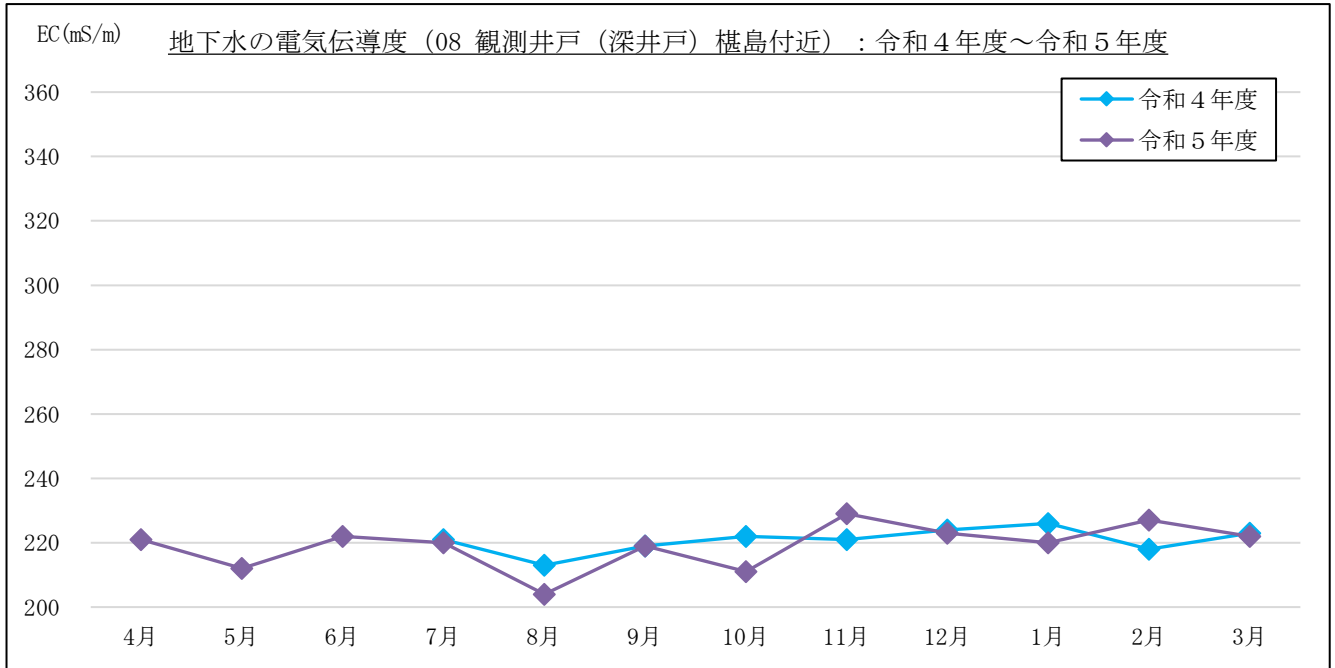
図 3-1-5 (11) 地下水の電気伝導度計測結果 : 08 観測井戸 (深井戸) 樫島付近
