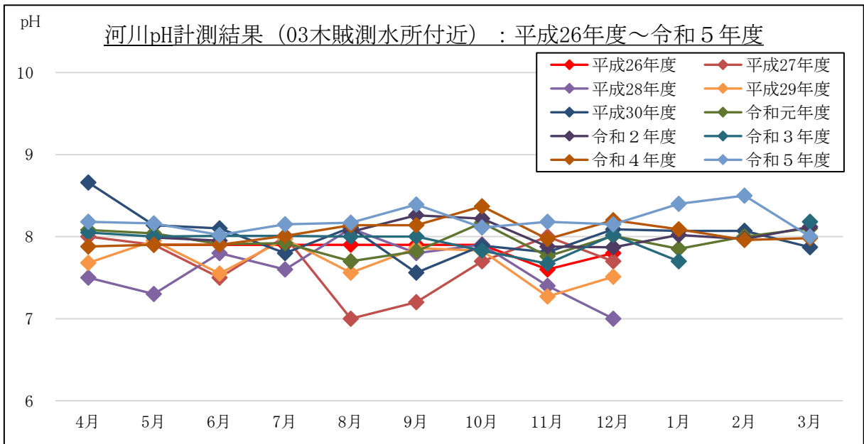
図 2-1-4(3) pH計測結果（流量（常時計測箇所））：03 木賊測水所付近
