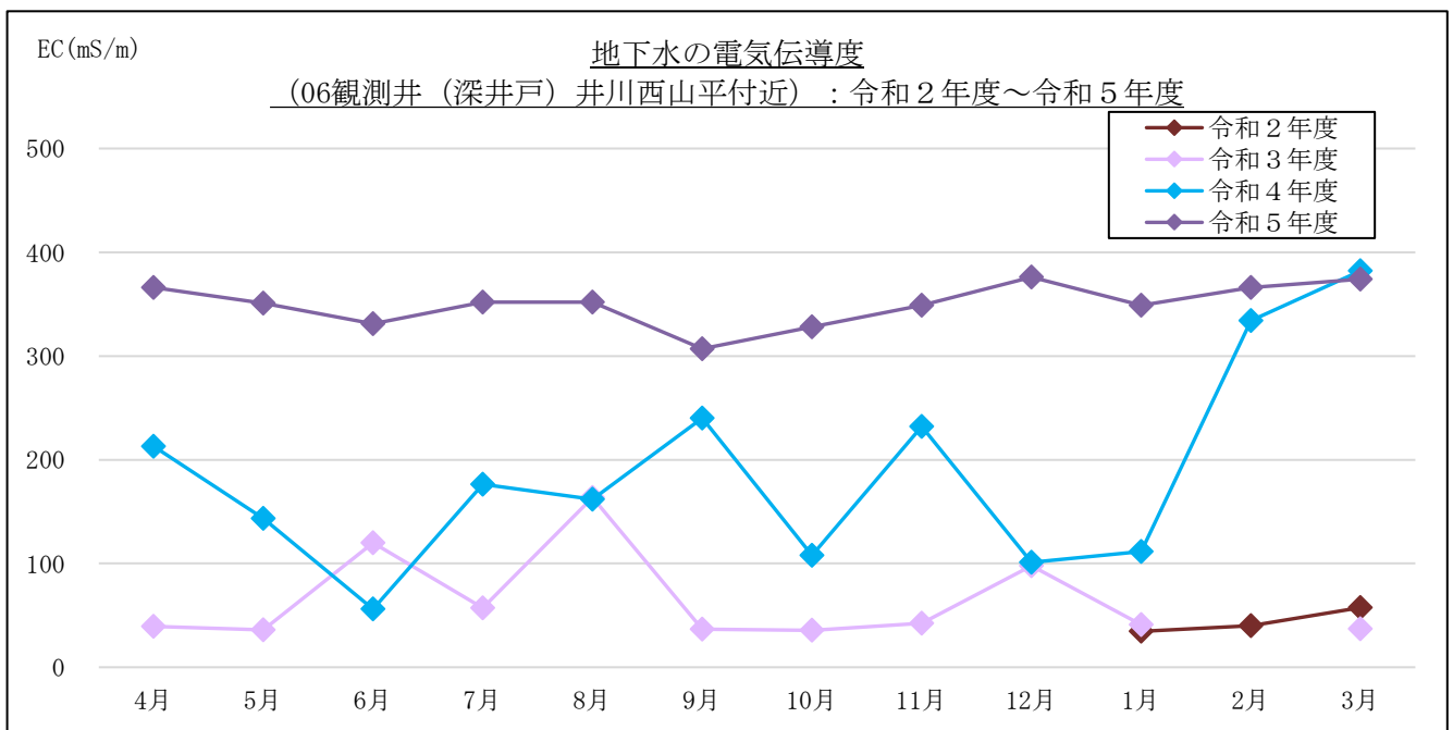
図 3-1-5 図 3-1-2(8) 地下水の電気伝導度計測結果 : 06 観測井戸 (深井戸) 井川西山平付近
