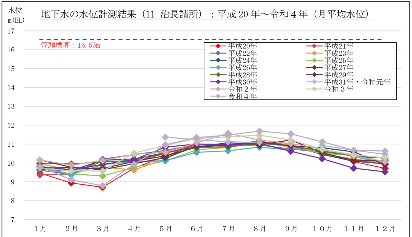
図 3-2-2(21) 地下水の水位計測結果 (月平均水位) : 11 治長請所 (焼津市治長請所)
