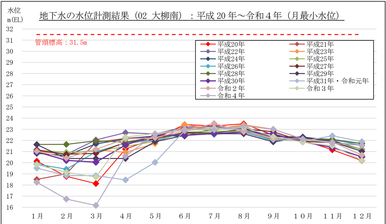
図 3-2-2(4) 地下水の水位計測結果 (月最小水位) : 02 大柳南 (島田市大柳)
