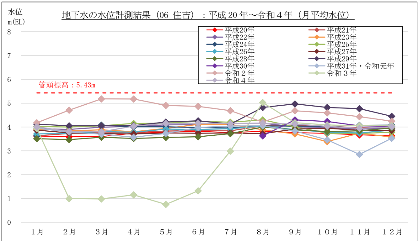
図 3-2-2(11) 地下水の水位計測結果 (月平均水位) : 06 住吉 (吉田町住吉)
