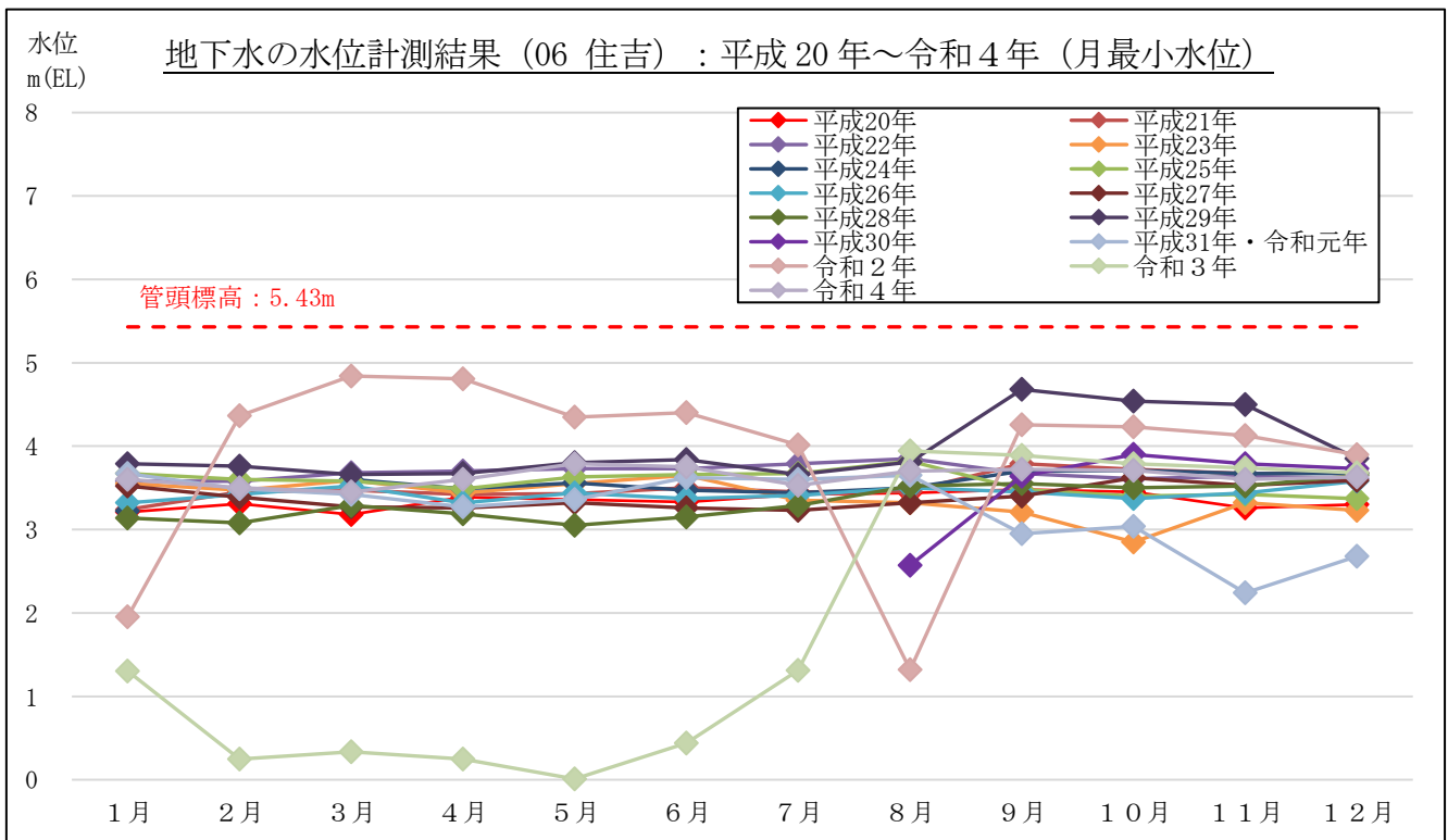
図 3-2-2(12) 地下水の水位計測結果 (月最小水位) : 06 住吉 (吉田町住吉)
