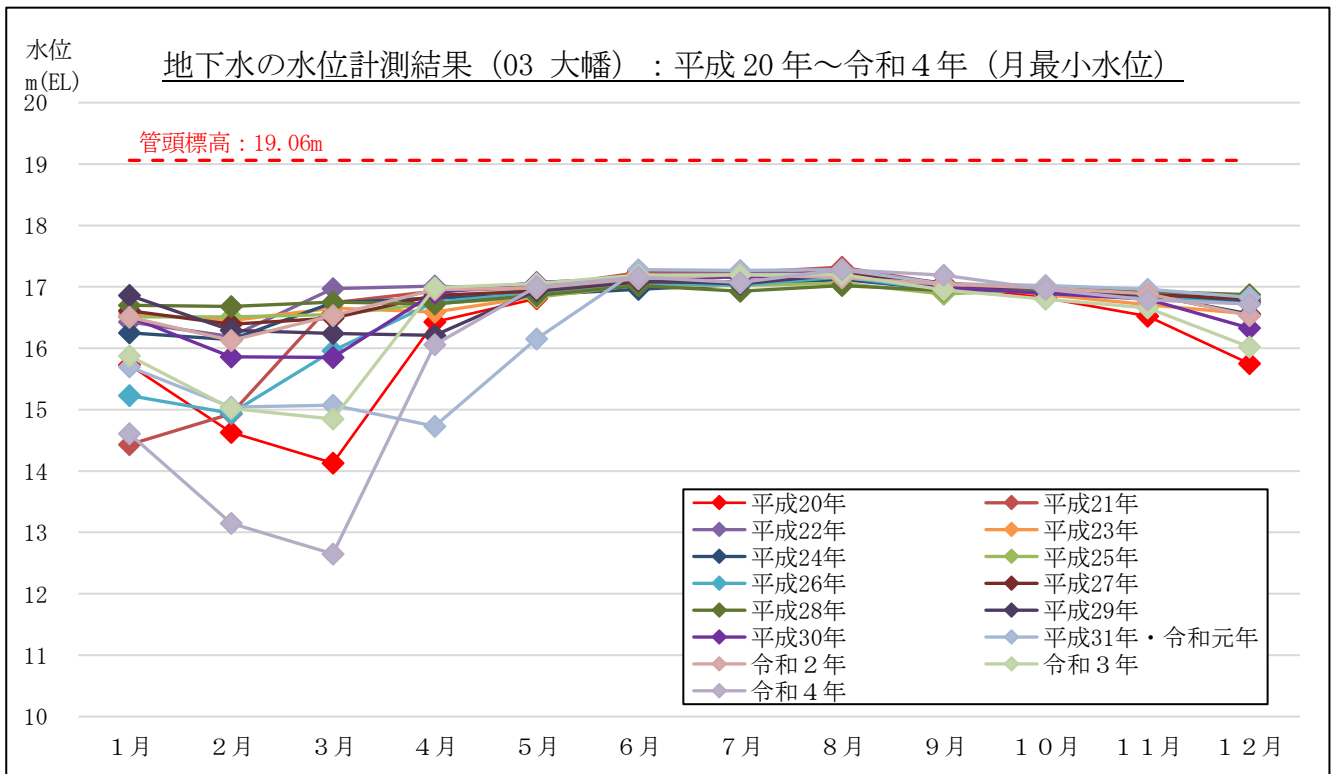
図 3-2-2(6) 地下水の水位計測結果 (月最小水位) : 03 大幡 (吉田町大幡)
