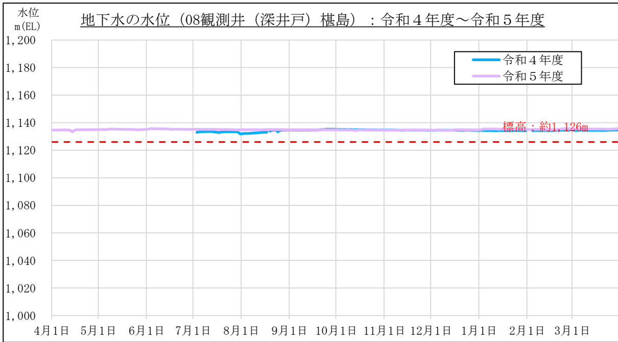
図 3-1-2(11) 地下水の水位計測結果 (常時計測) : 08 観測井戸 (深井戸) 榎島付近
