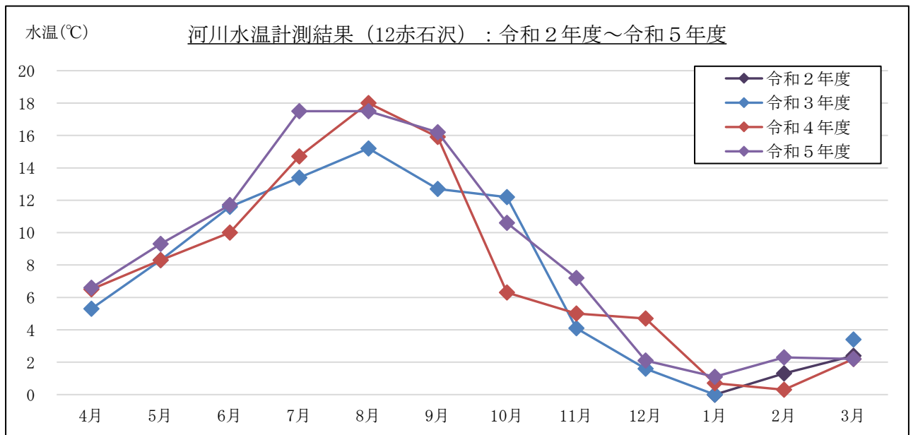
図 2-1-7(8) 水温計測結果 (流量 (月1回計測箇所)) : 12 赤石沢
