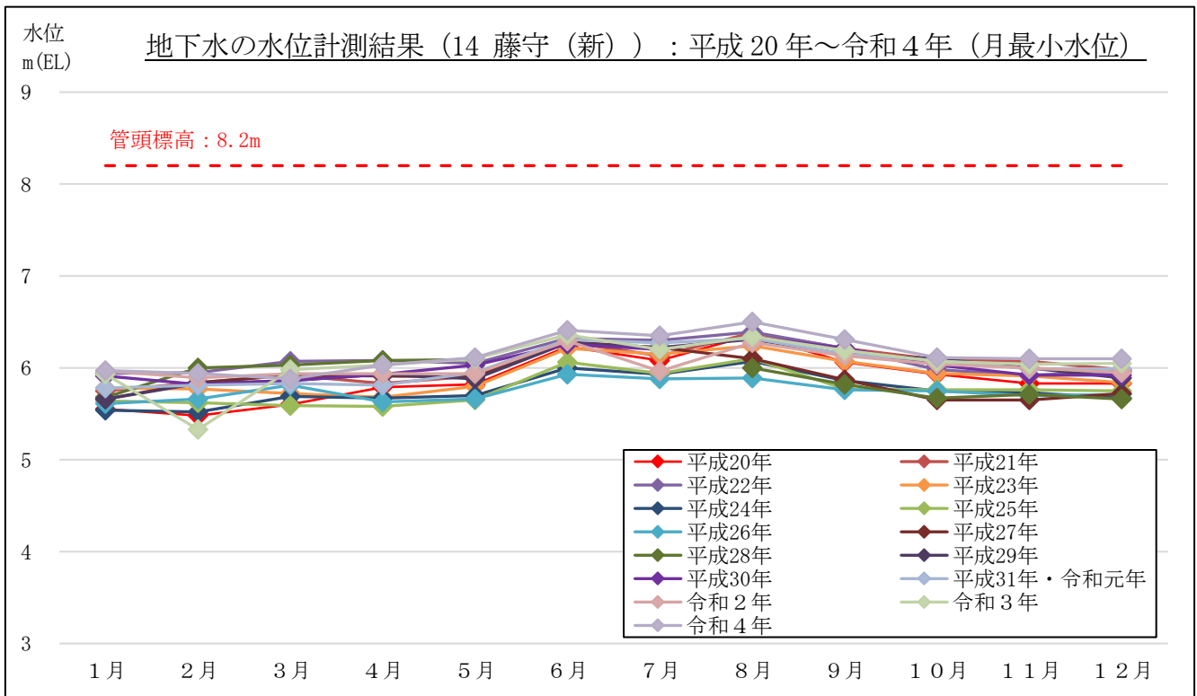
図 3-2-2(28) 地下水の水位計測結果 (月最小水位) : 14 藤守 (新) (烧津市藤守)
