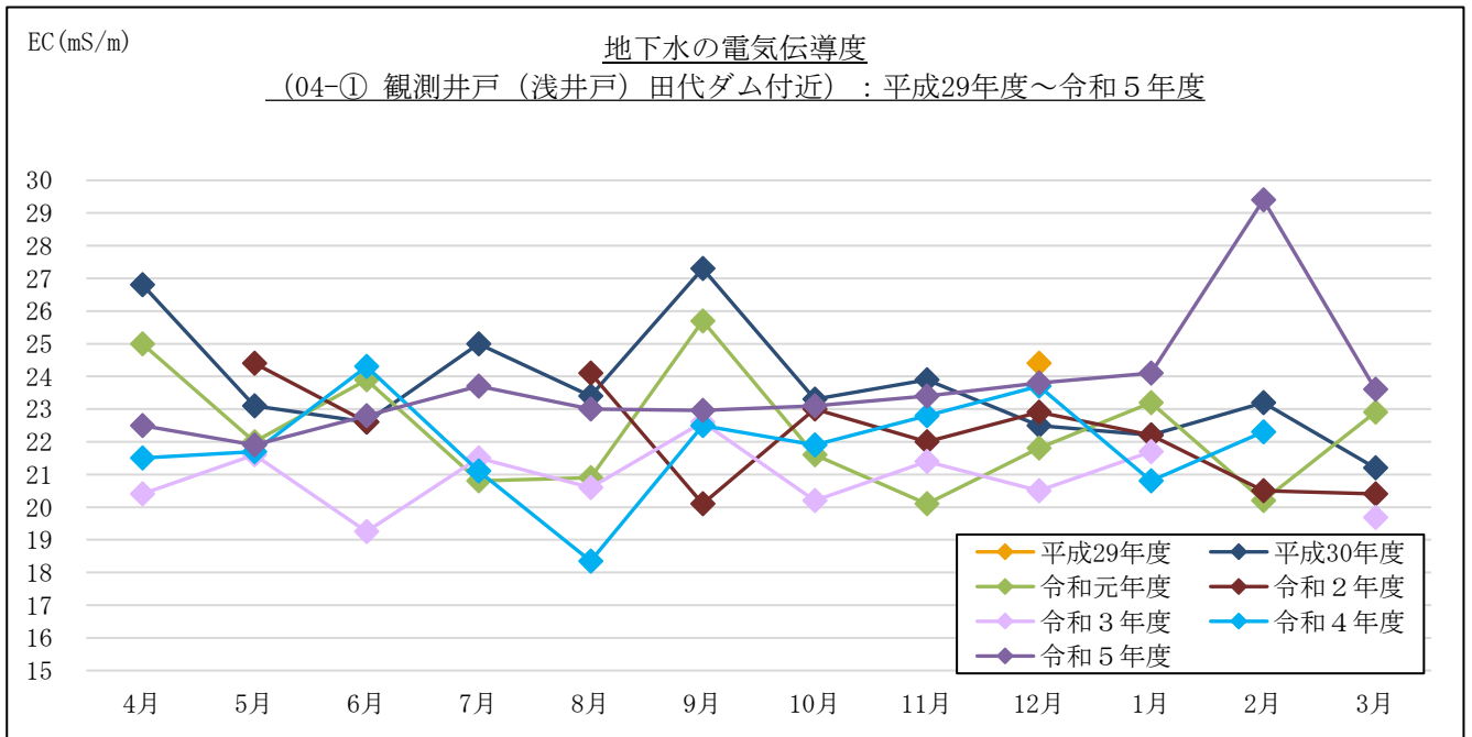
図 3-1-5(5) 地下水の電気伝導度計測結果 : 04-① 観測井戸 (浅井戸) 田代ダム付近
