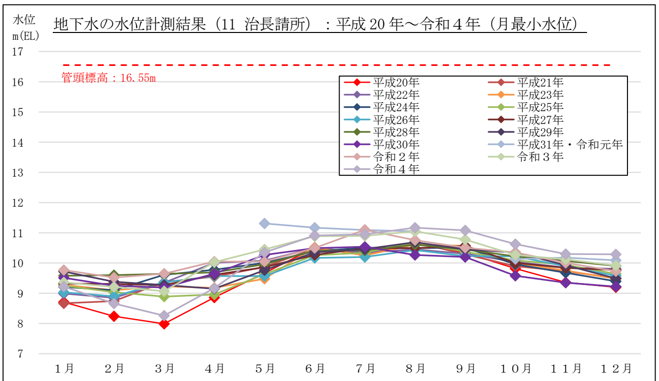
図 3-2-2(22) 地下水の水位計測結果 (月最小水位) : 11 治長請所 (焼津市治長請所)
