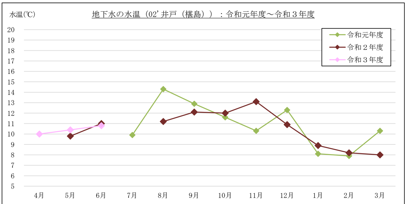
図 3-1-3(3) 地下水の水温計測結果 : 02' 井戸 (樺島宿舎)
