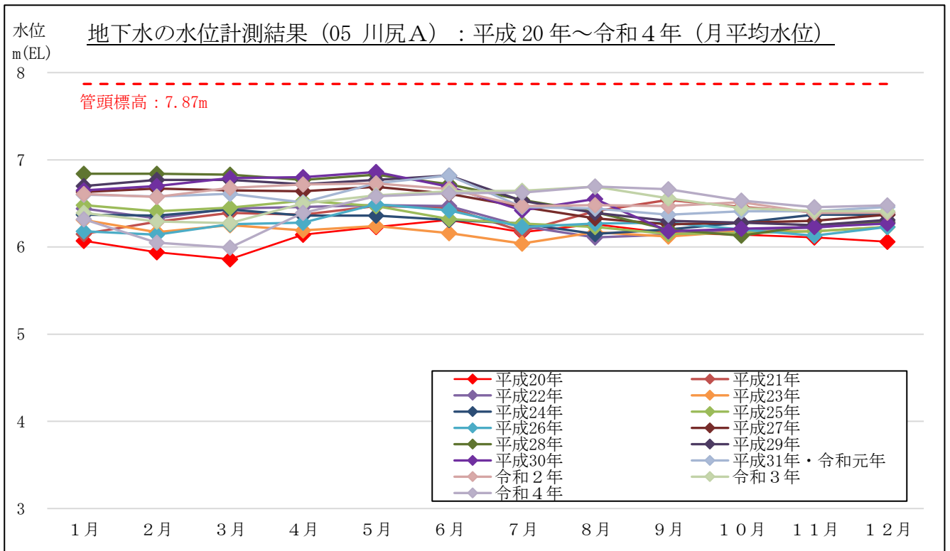
図 3-2-2(9) 地下水の水位計測結果 (月平均水位) : 05 川尻A (吉田町川尻)
