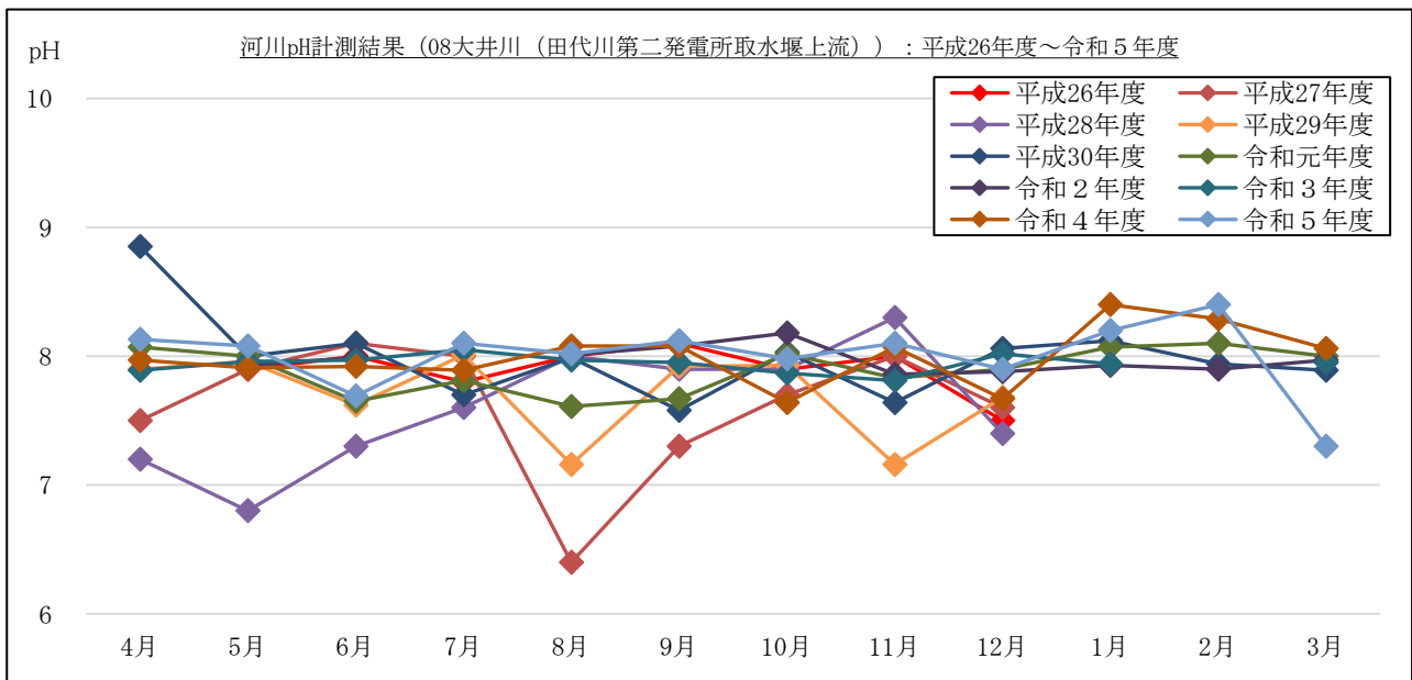
図 2-1-8(4) pH計測結果（流量（月1回計測箇所））：08 大井川（田代ダム上流）
