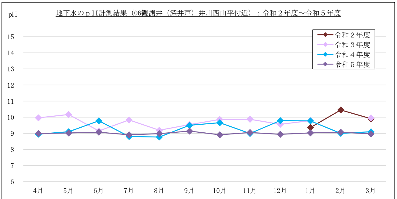
図 3-1-4(8) 地下水のpH計測結果 : 06 観測井戸 (深井戸) 井川西山平付近
