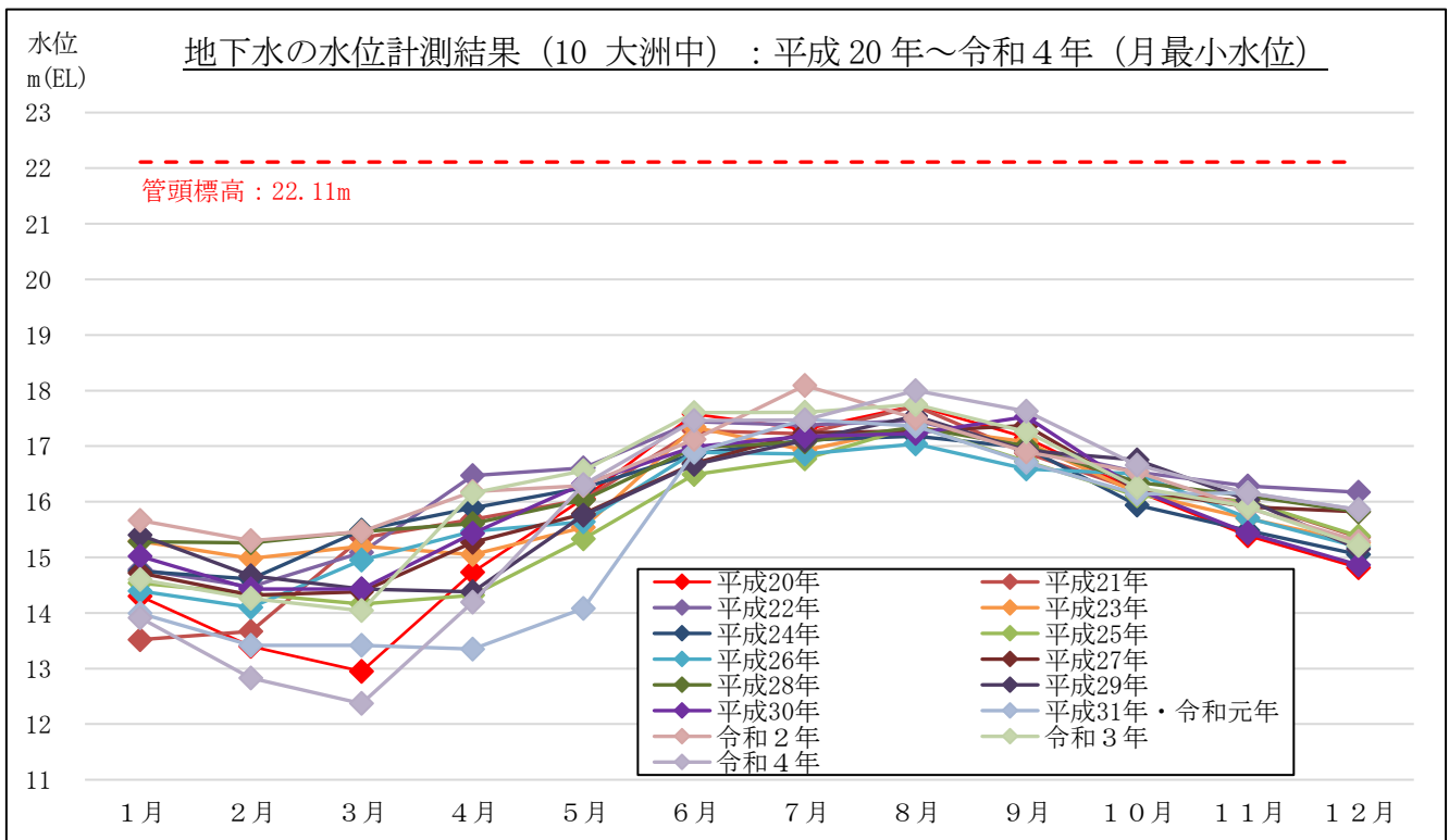
図 3-2-2(20) 地下水の水位計測結果 (月最小水位) : 10 大洲中 (藤枝市弥左工門)
