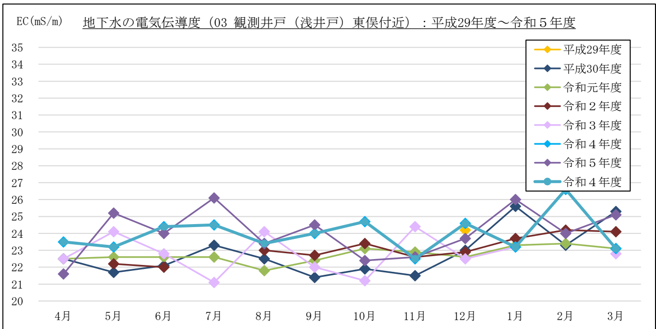
図 3-1-5(4) 地下水の電気伝導度計測結果:03観測井戸(浅井戸)東俣付近
