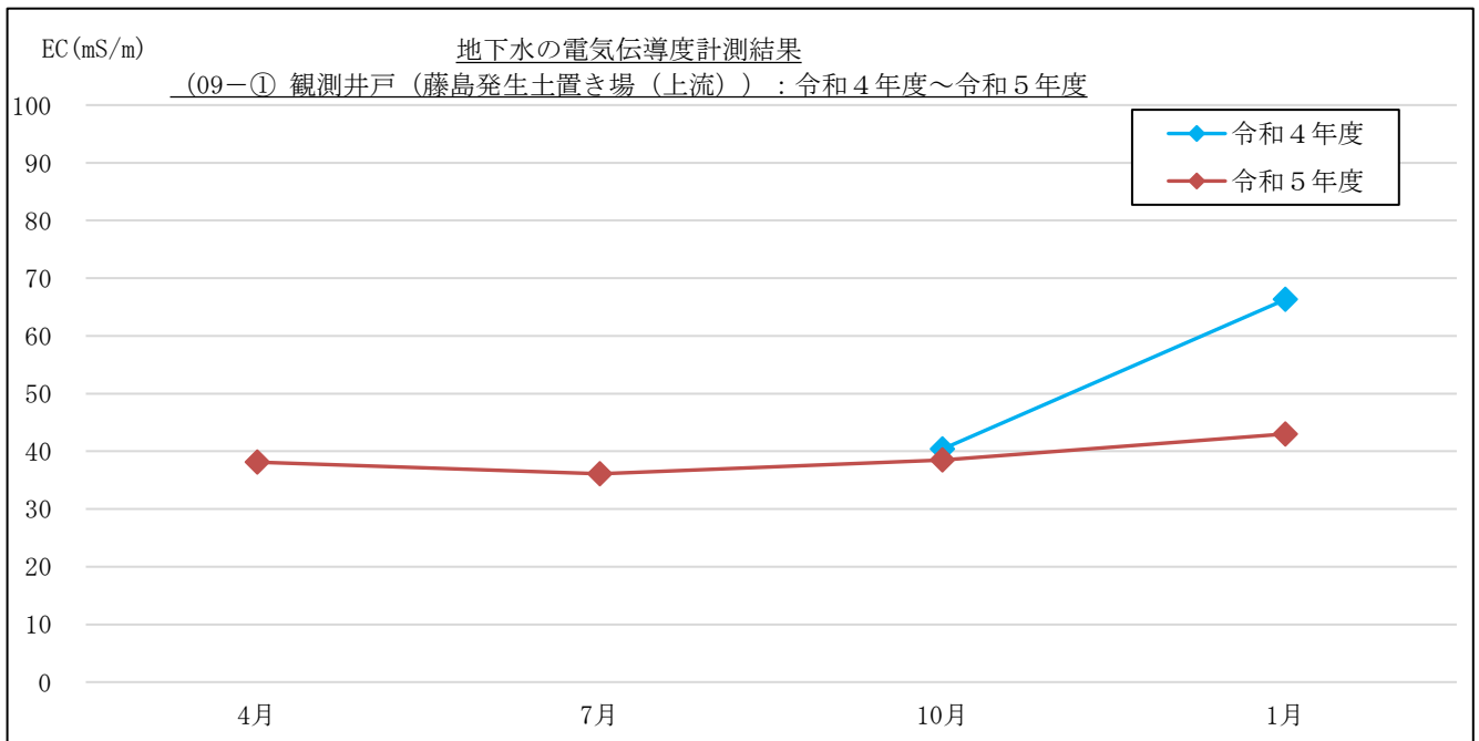
図 3-1-5 (12) 地下水の電気伝導度計測結果 : 09-① 観測井戸 (上流側) 藤島発生土置き場付近
