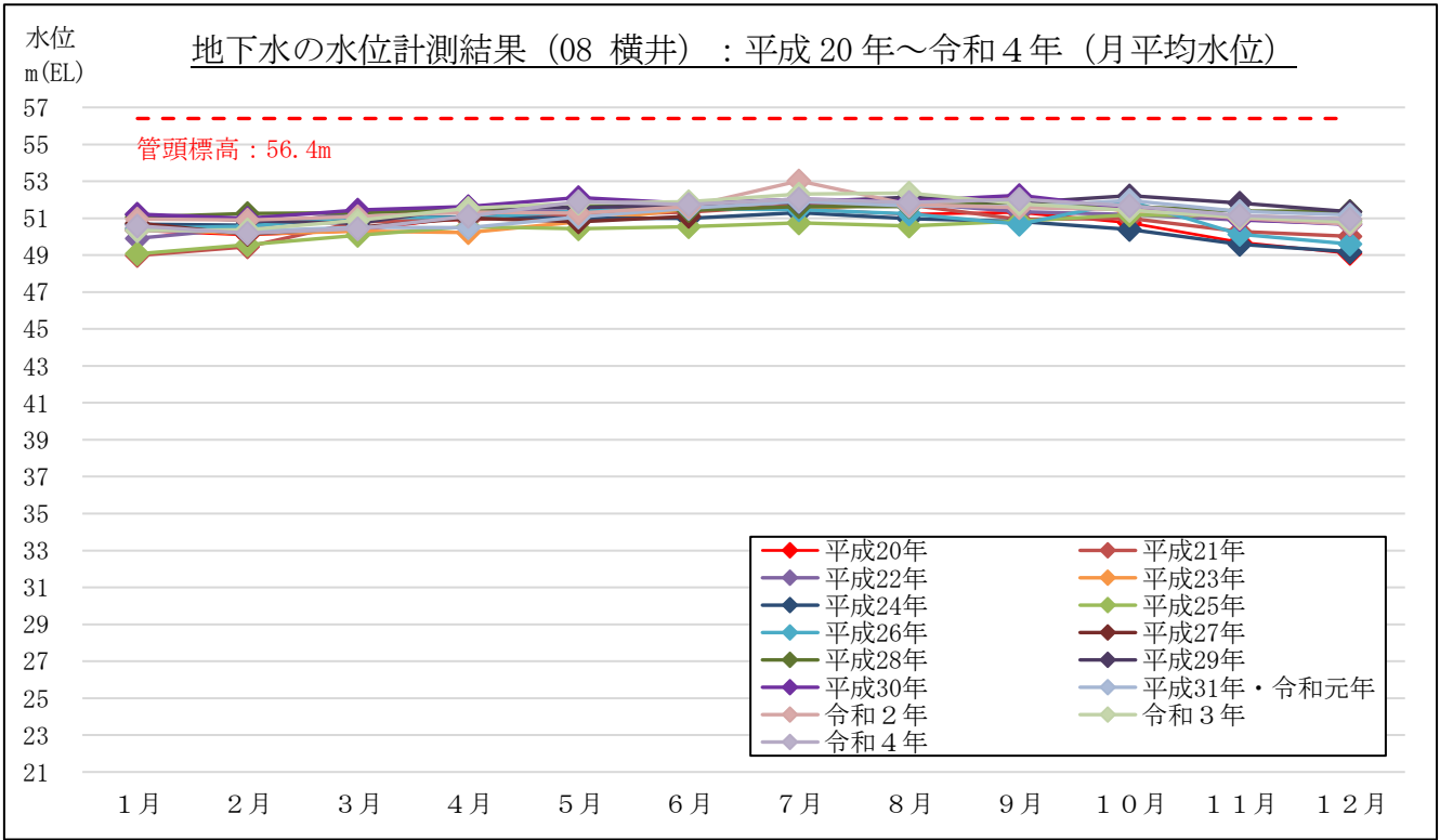
図 3-2-2(15) 地下水の水位計測結果 (月平均水位) : 08 横井 (島田市横井)
