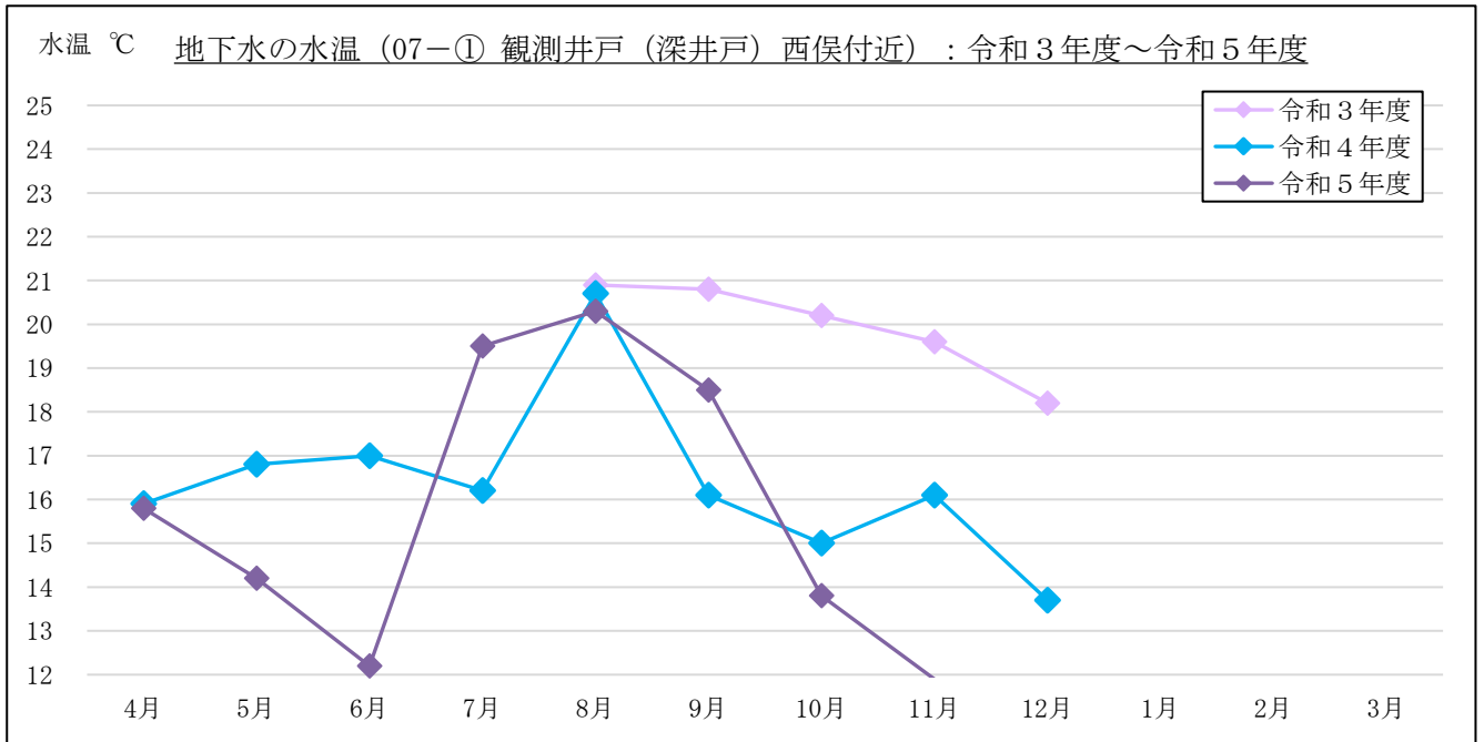
図 3-1-3(9) 地下水の水温計測結果 : 07-① 観測井戸 (深井戸) 西俣付近
