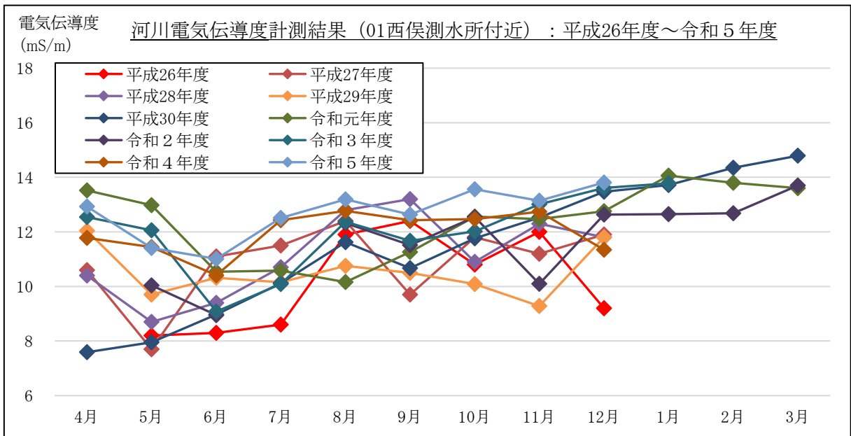
図 2-1-5(1) 電気伝導度計測結果（流量（常時計測箇所））：01 西俣測水所付近
