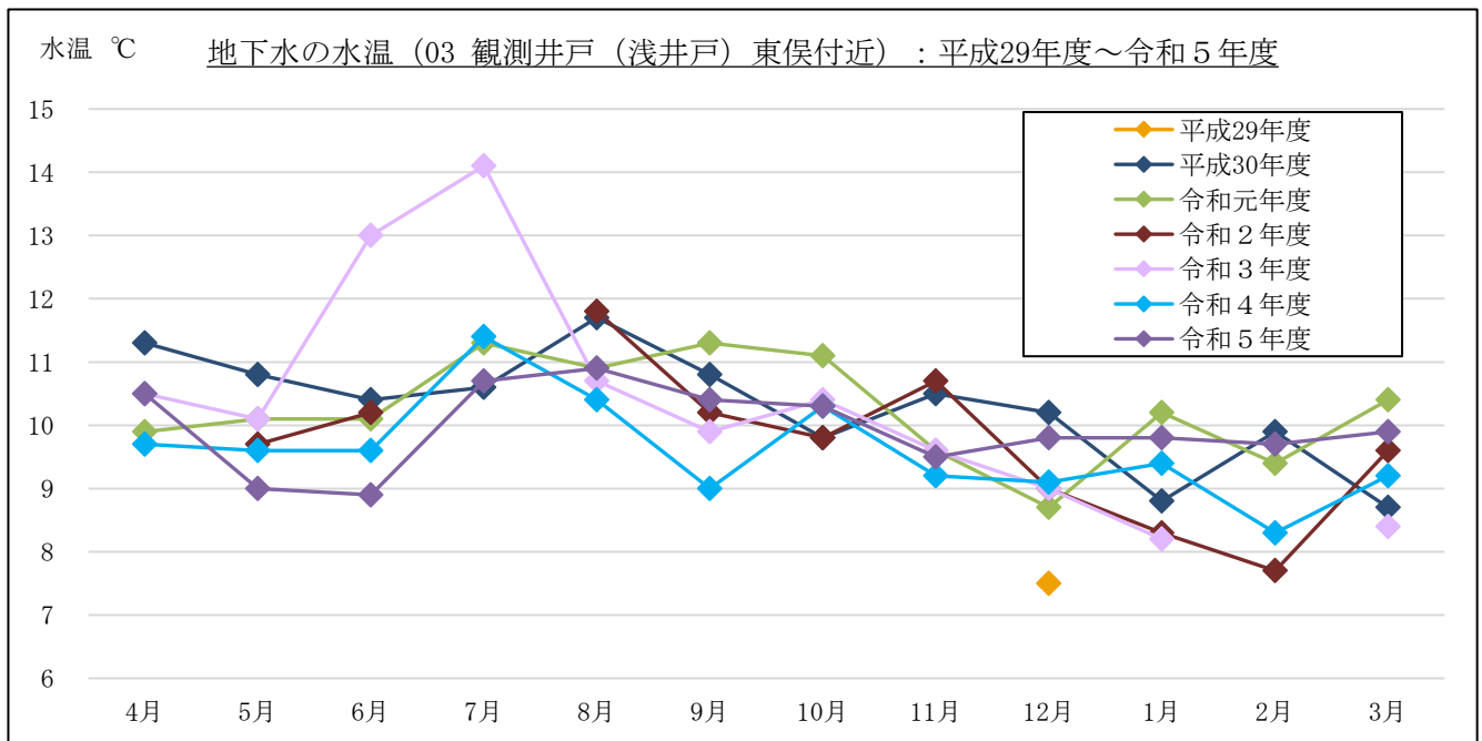
図 3-1-3(4) 地下水の水温計測結果 : 03 観測井戸 (浅井戸) 東俣付近
