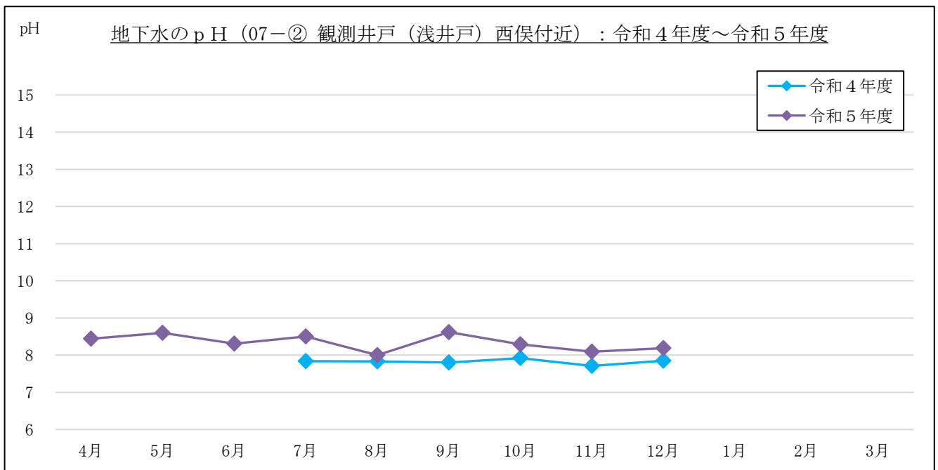
図 3-1-4(10) 地下水のpH計測結果 : 07-② 観測井戸 (浅井戸) 西俣付近
