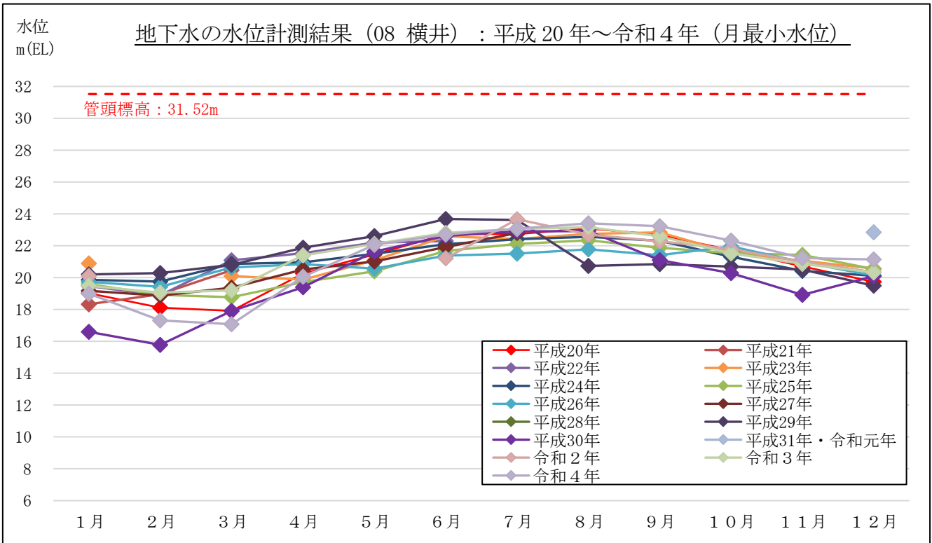
図 3-2-2(16) 地下水の水位計測結果 (月最小水位) : 08 横井 (島田市横井)
