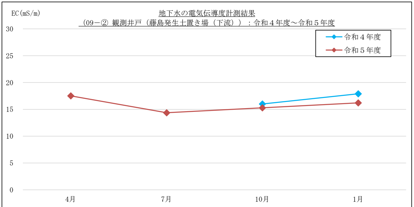
図 3-1-5 (13) 地下水の電気伝導度計測結果 : 09-② 観測井戸 (下流側) 藤島発生土置き場付近
