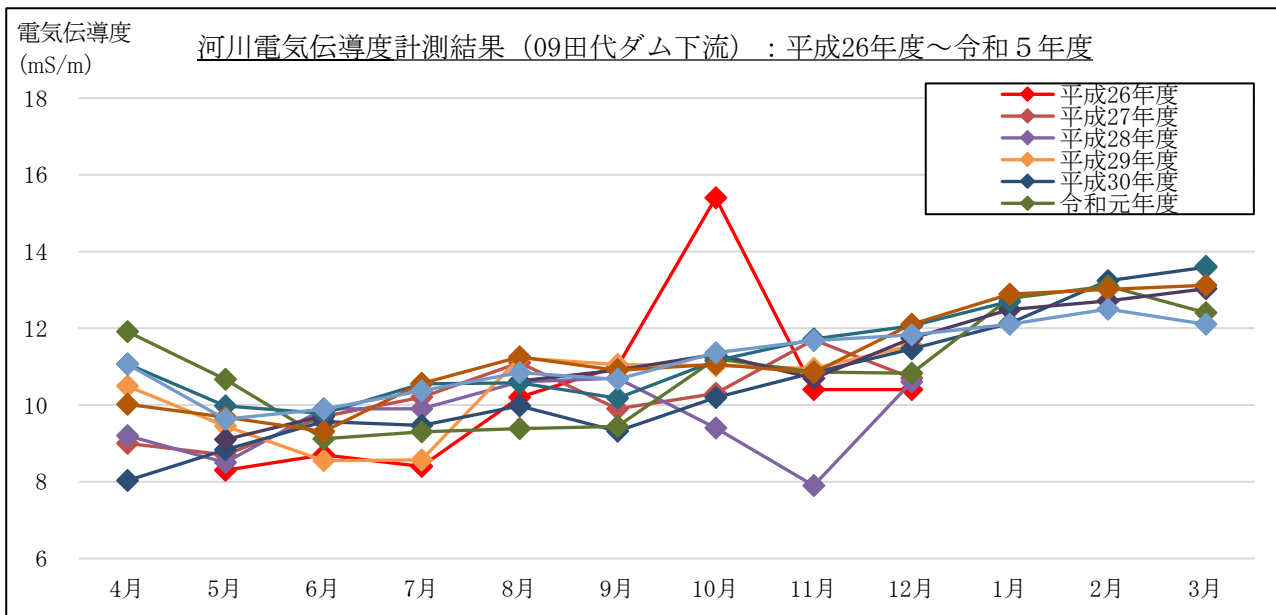
図 2-1-9(5) 電気伝導度計測結果 (流量 (月1回計測箇所)) : 09 大井川 (田代ダム下流)
