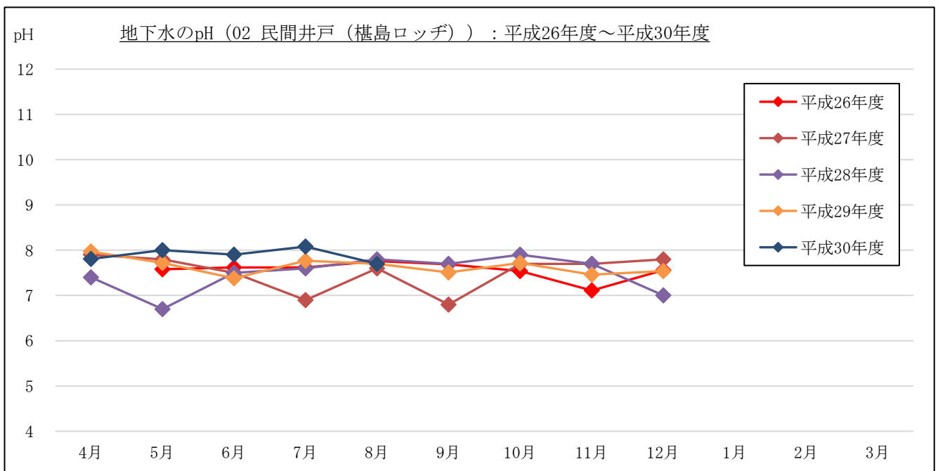
図 3-1-4(2) 地下水の pH 計測結果 : 02 民間井戸 (榎島ロッヂ)
