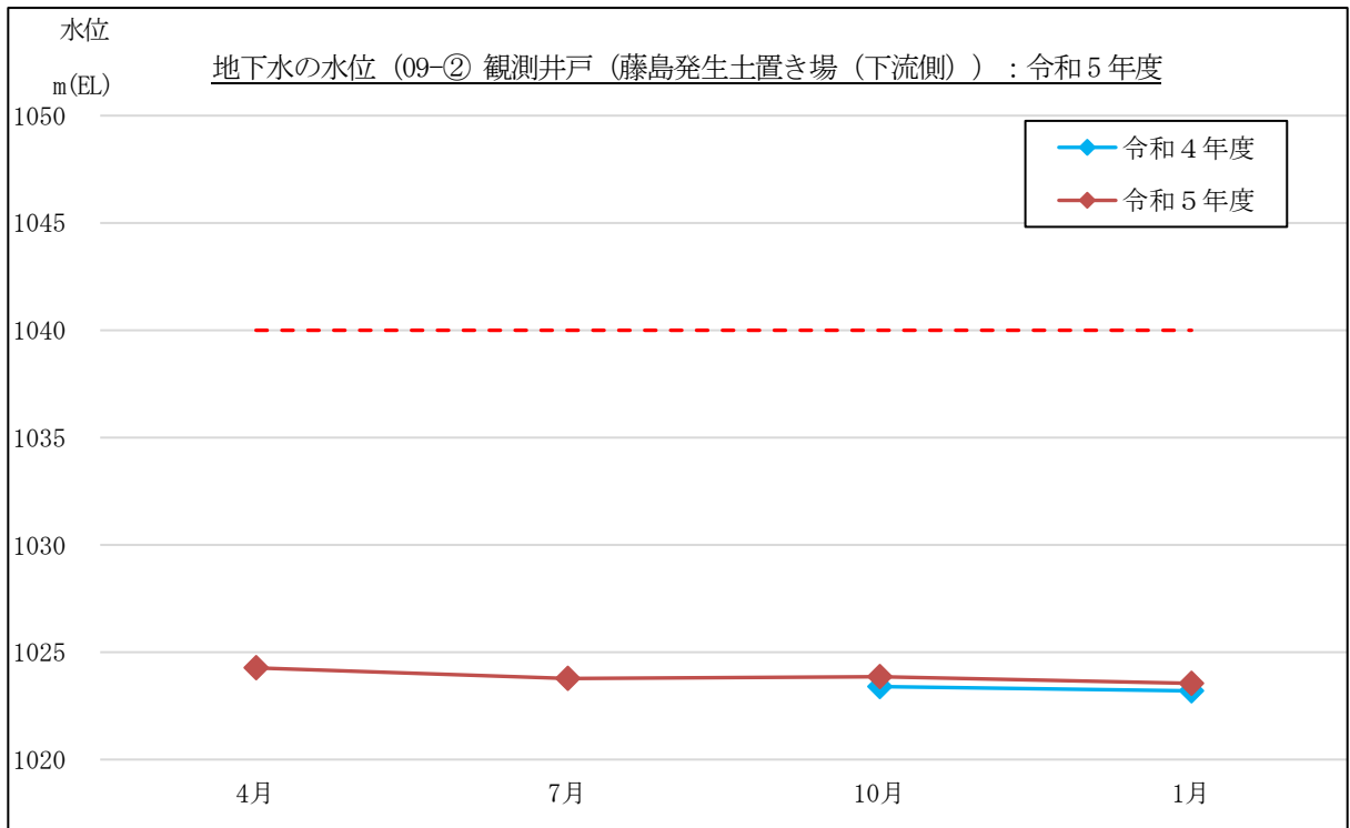
図 3-1-2(13) 地下水の水位計測結果 (常時計測) : 09-② 観測井戸 (下流側) 藤島発生土置き場付近
