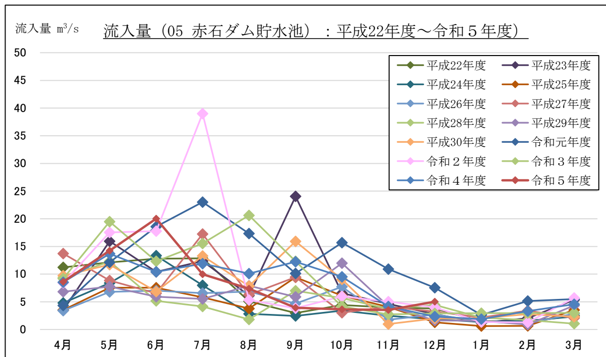
図 2-1-2(5) 流量計測結果 (流量 (常時計測箇所)) : 13 赤石ダム貯水池
