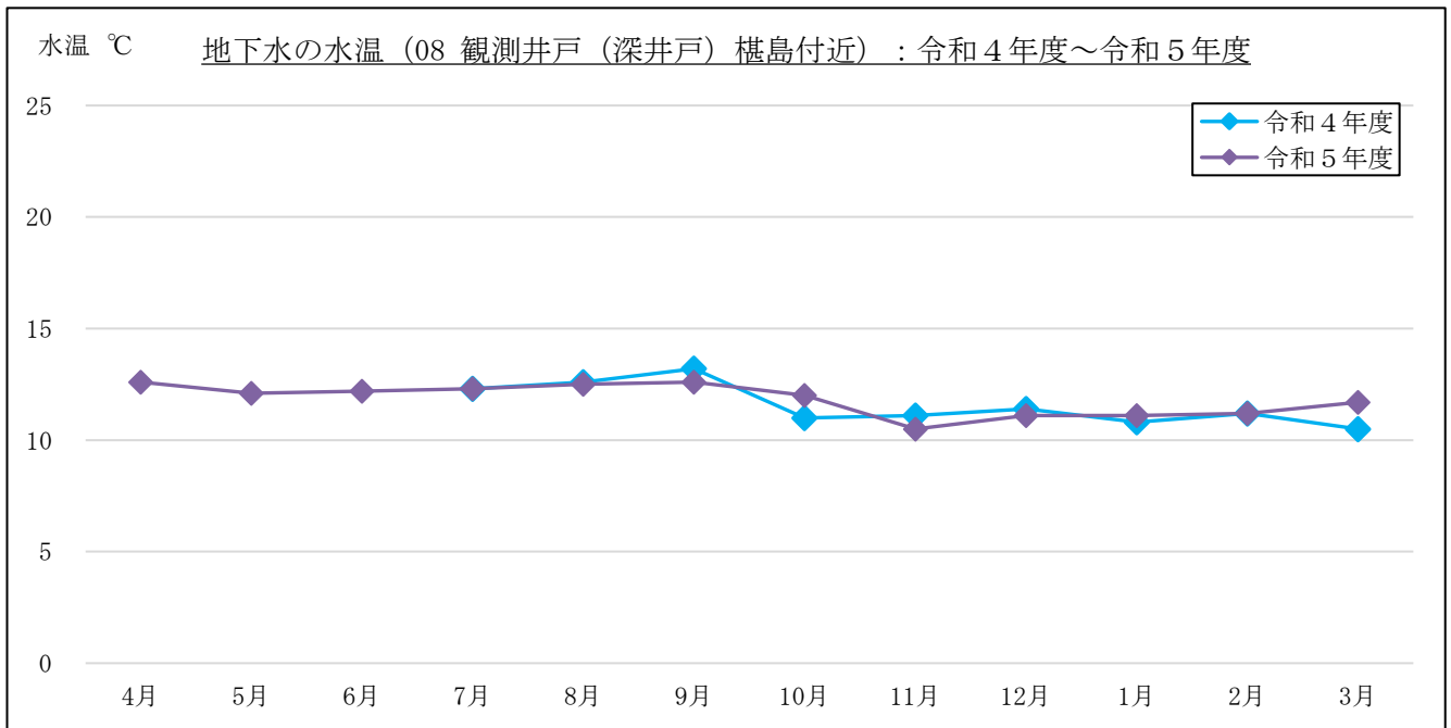
図 3-1-3(11) 地下水の水温計測結果 : 08 観測井戸 (深井戸) 榎島付近
