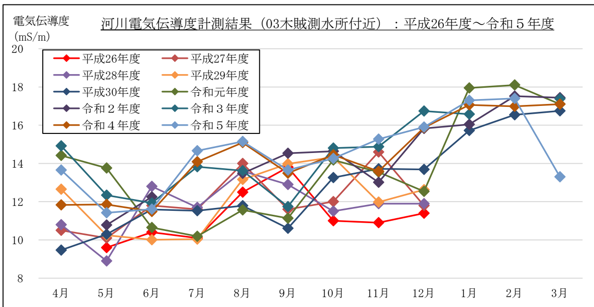
図 2-1-5(3) 電気伝導度計測結果 (流量 (常時計測箇所)) : 03 木賊測水所付近
