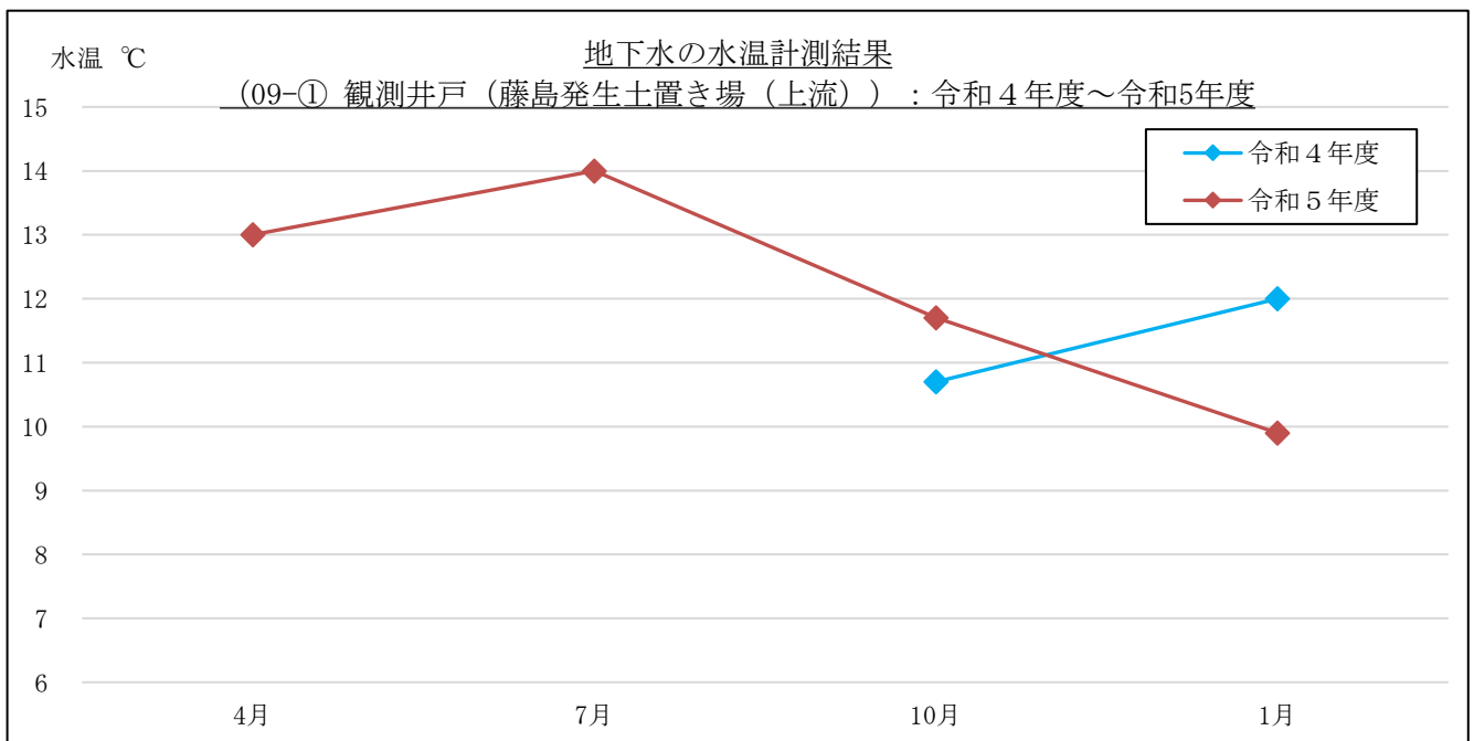
図 3-1-3(12) 地下水の水温計測結果 : 09-① 観測井戸 (上流側) 藤島発生土置き場付近
