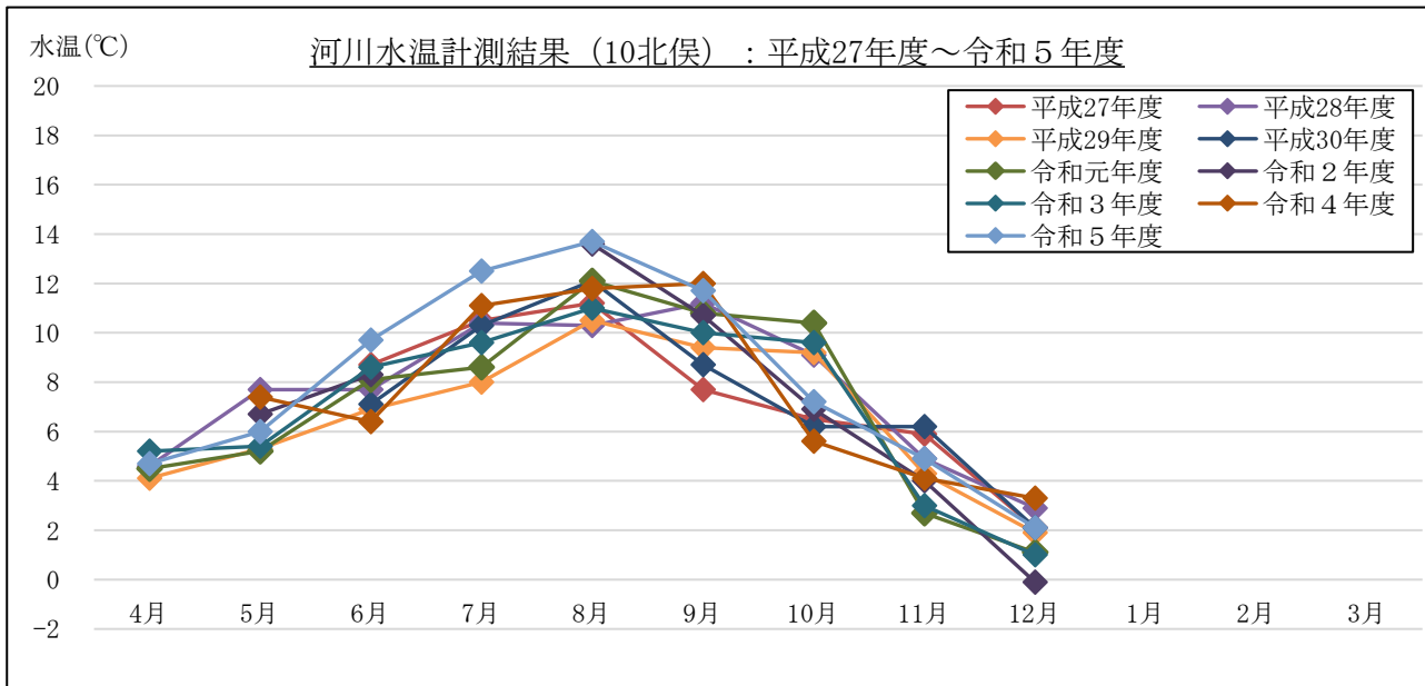
図 2-1-7(6) 水温計測結果 (流量 (月1回計測箇所)) : 10 北俣
