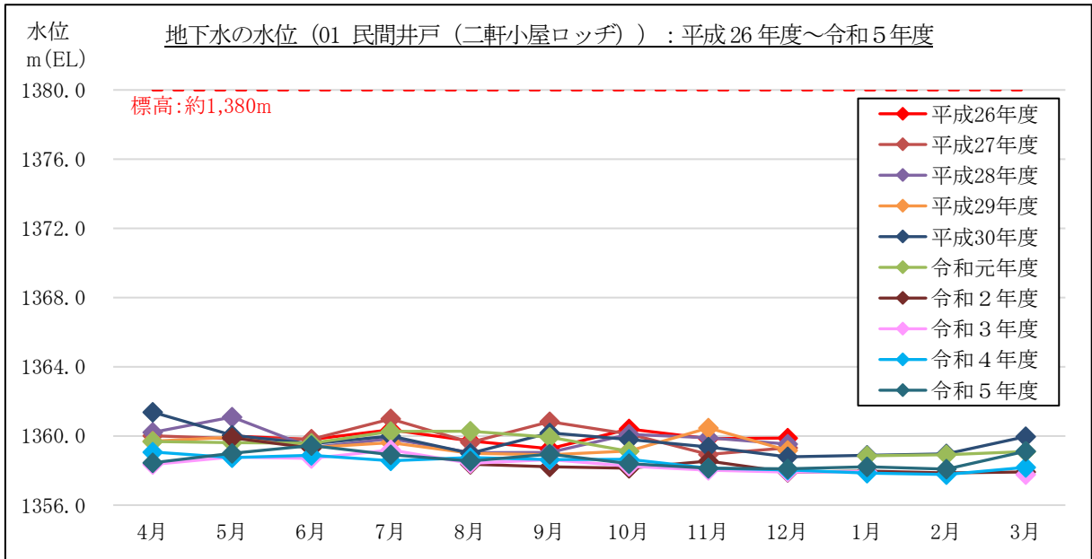
図 3-1-2(1) 地下水の水位計測結果 (月1回計測) : 01 民間井戸 (二軒小屋ロッヂ)
