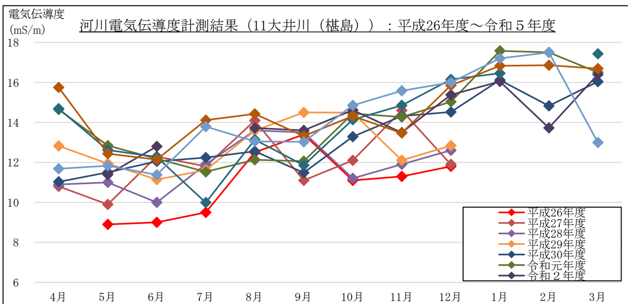
図 2-1-9(6) 電気伝導度計測結果 (流量 (月1回計測箇所)) : 10 北俣
