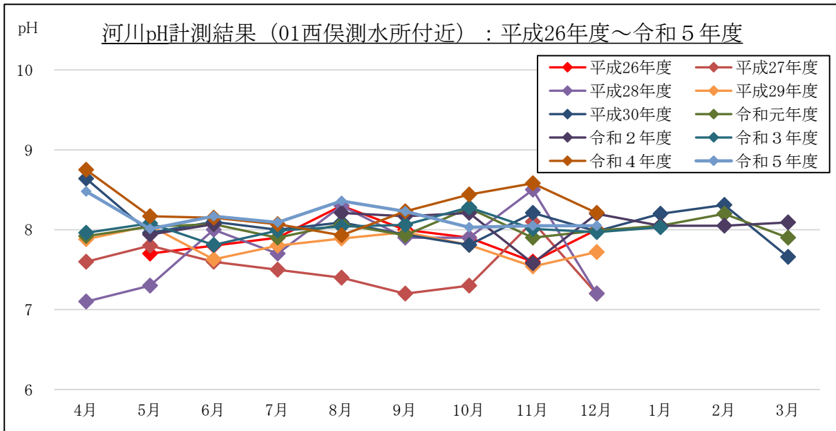
图 2-1-4(1) pH 計測結果 (流量 (常時計測箇所)) : 01 西俣測水所付近
