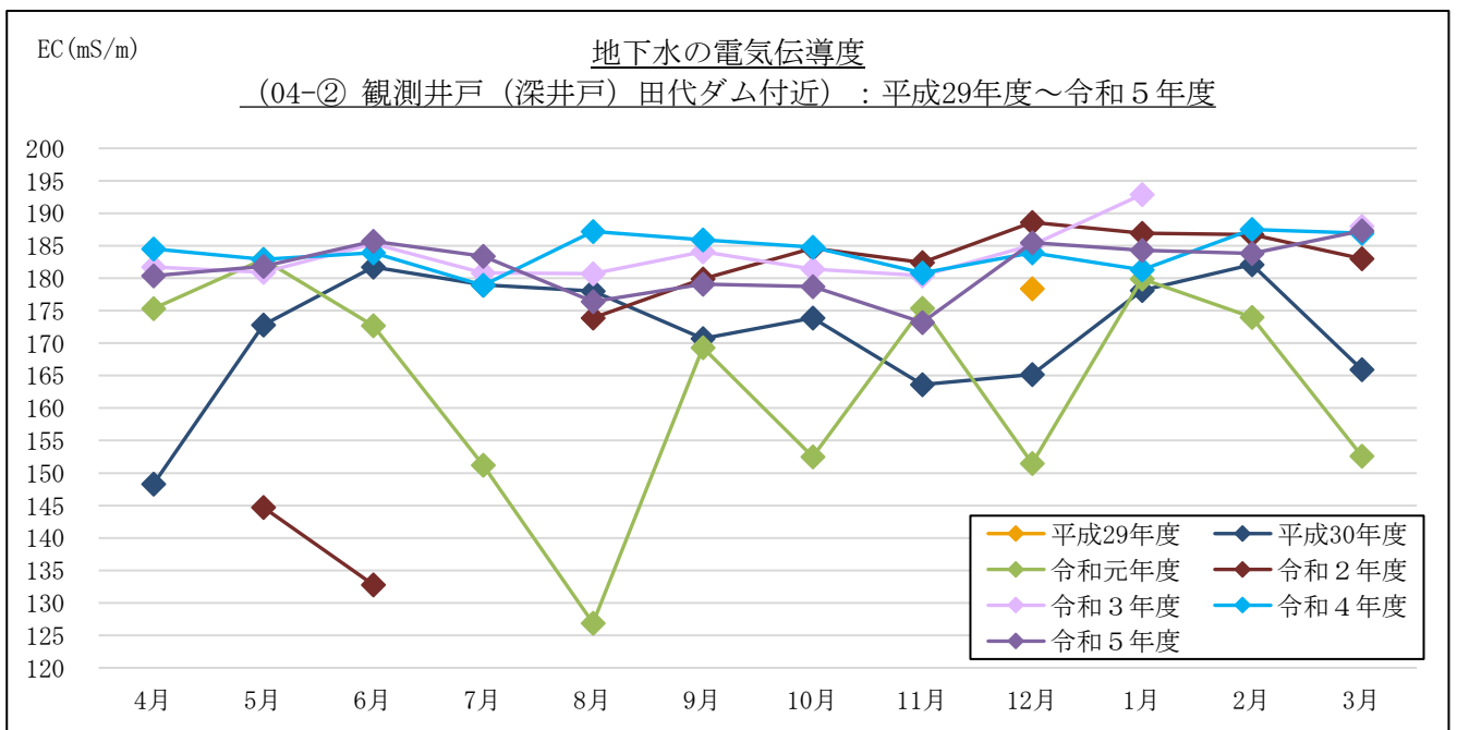
図 3-1-5(6) 地下水の電気伝導度計測結果 : 04-② 観測井戸 (深井戸) 田代ダム付近
