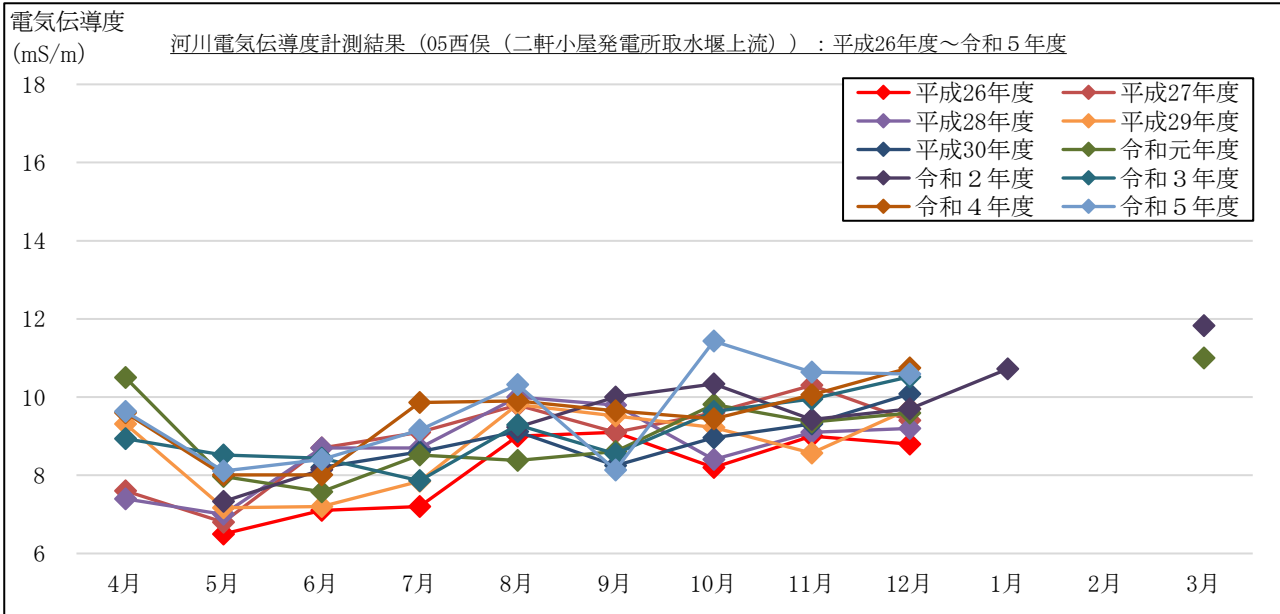
図 2-1-9(1) 電気伝導度計測結果 (流量 (月1回計測箇所)) : 05 西俣 (二軒小屋発電所取水堰上流)
