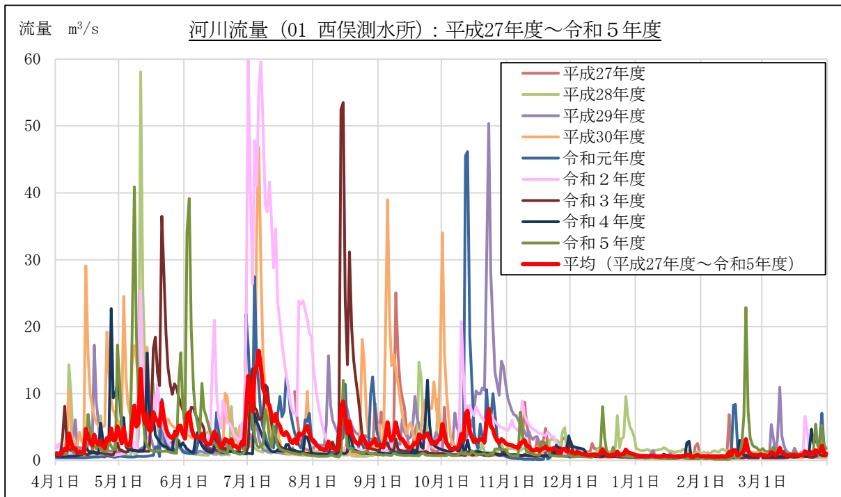
図 2-1-2(1) 流量計測結果 (流量 (常時計測箇所)) : 01 西俣測水所
