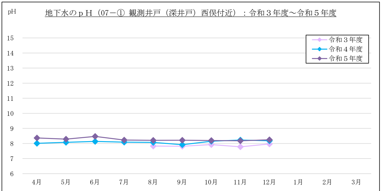
図 3-1-4(9) 地下水のpH計測結果 : 07-① 観測井戸 (深井戸) 西俣付近
