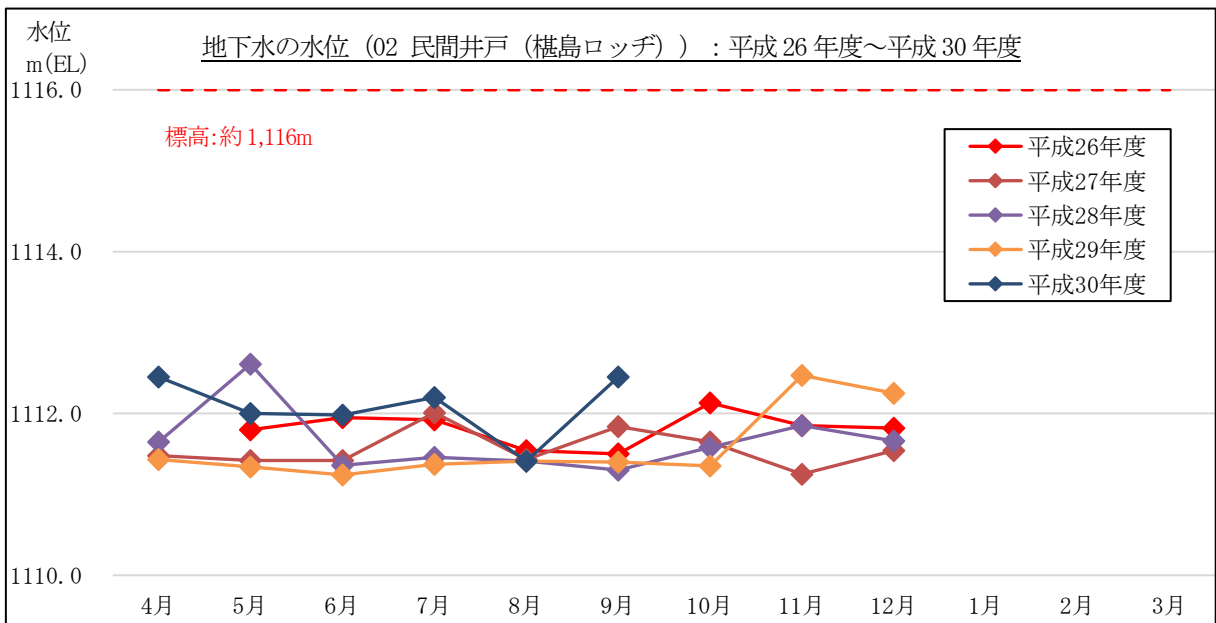
図 3-1-2(2) 地下水の水位計測結果 (月1回計測) : 02 民間井戸 (樫島ロッヂ)
