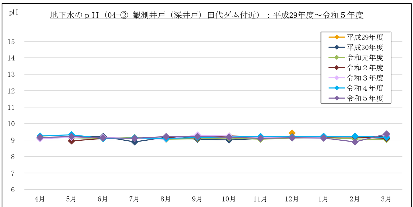
図 3-1-4(6) 地下水のpH計測結果 : 04-② 観測井戸 (深井戸) 田代ダム付近
