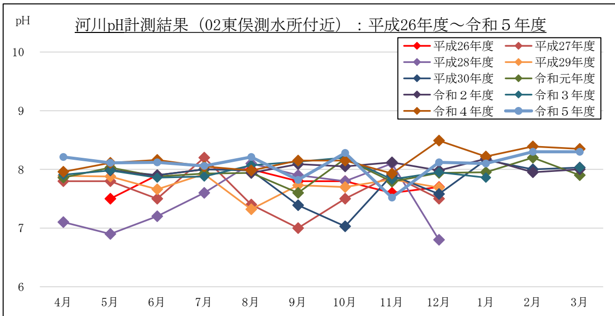
图 2-1-4(2) pH 計測結果 (流量 (常時計測箇所)) : 02 東俣第一測水所付近
