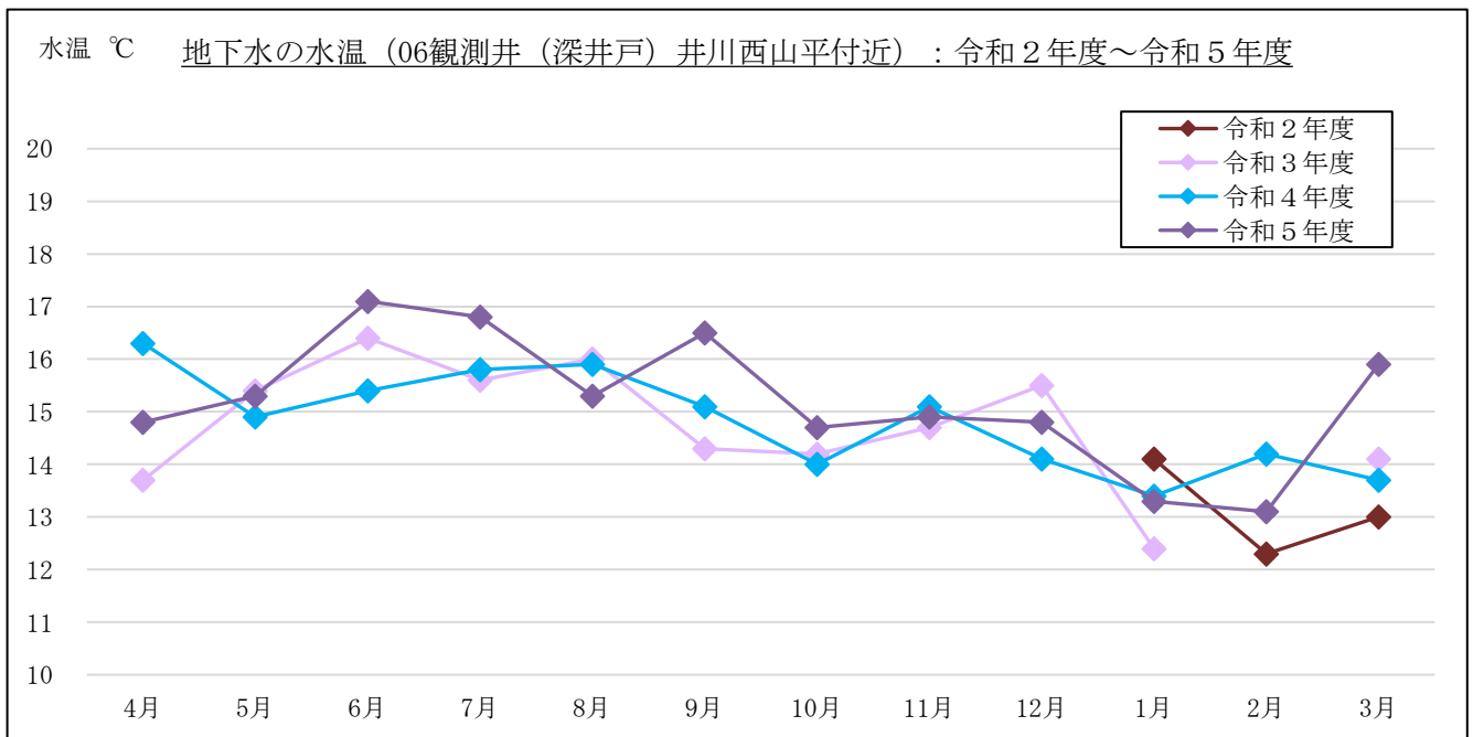
図 3-1-3(8) 地下水の水温計測結果 : 06 観測井戸 (深井戸) 井川西山平付近
