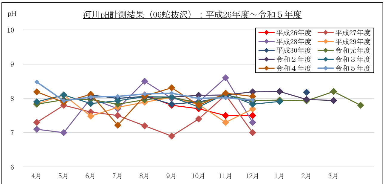
図 2-1-8(2) pH 計測結果 (流量 (月 1 回計測箇所)) : 06 蛇抜沢
