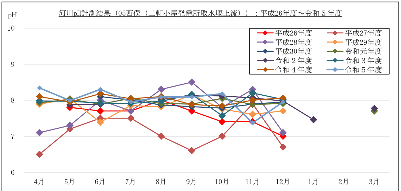
図 2-1-8(1) pH 計測結果 (流量 (月 1 回計測箇所)) : 05 西俣 (二軒小屋発電所取水堰上流)
