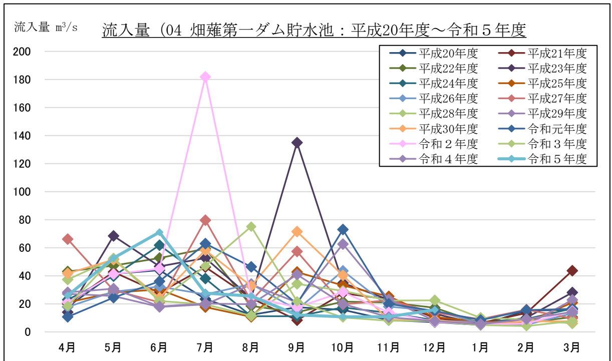
図 2-1-2(4) 流量計測結果 (流量 (常時計測箇所)) : 04 畑薙第一ダム貯水池
