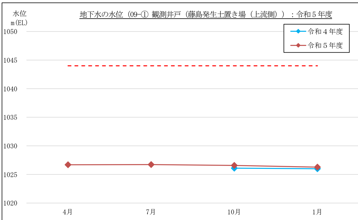
図 3-1-2(12) 地下水の水位計測結果 (常時計測) : 09-① 観測井戸 (上流側) 藤島発生土置き場付近
