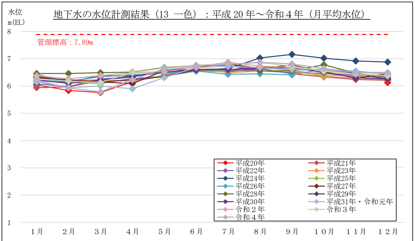
図 3-2-2(25) 地下水の水位計測結果 (月平均水位) : 13 一色 (焼津市一色)
