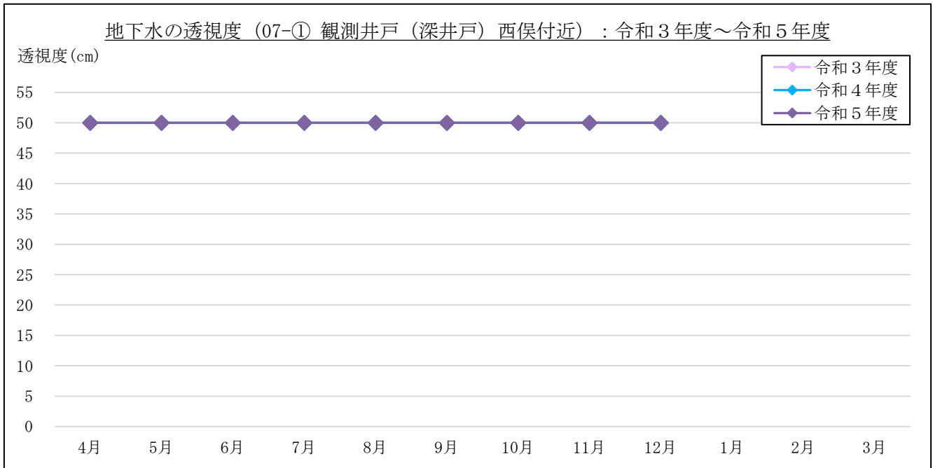
図 3-1-6(9) 地下水の透視度計測結果 : 07-① 観測井戸 (深井戸) 西俣付近
