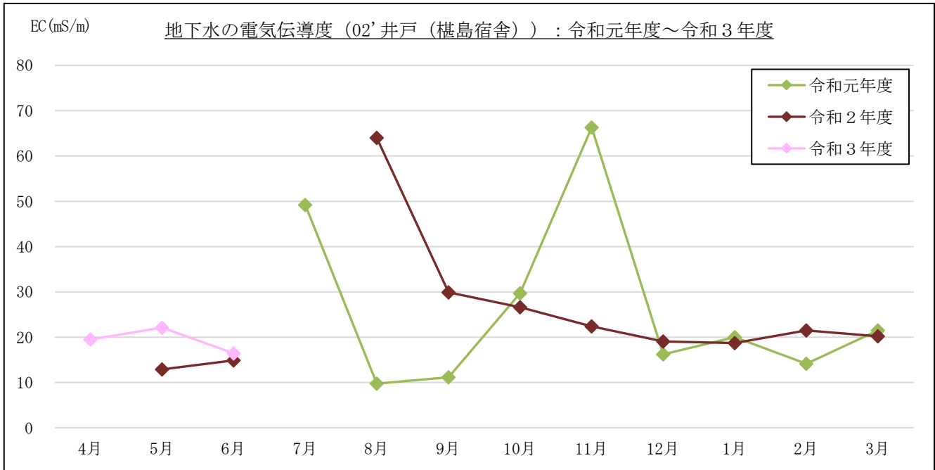
図 3-1-5(3) 地下水の電気伝導度計測結果:02' 井戸(榎島宿舎)
