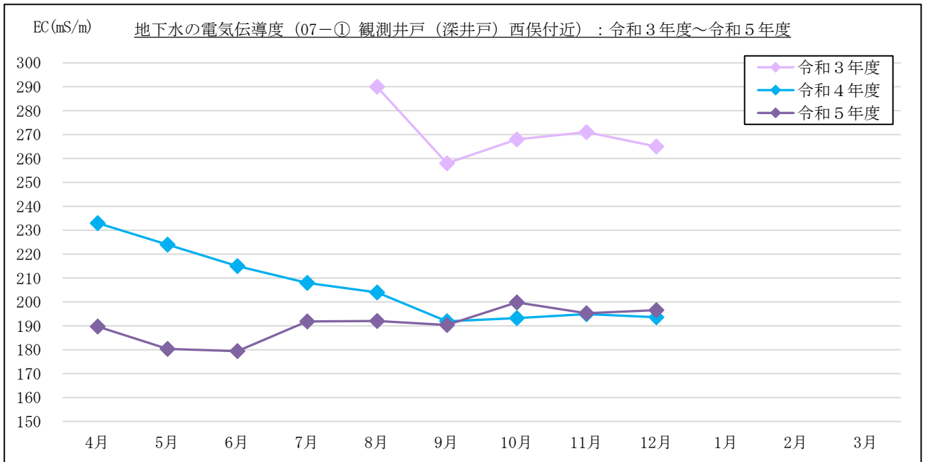
図 3-1-5(9) 地下水の電気伝導度計測結果 : 07-① 観測井戸 (深井戸) 西俣付近
