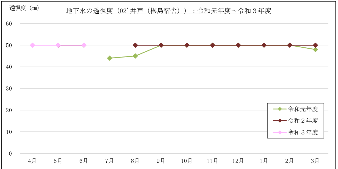
図 3-1-6(3) 地下水の透視度計測結果 : 02' 井戸 (榎島宿舎)
