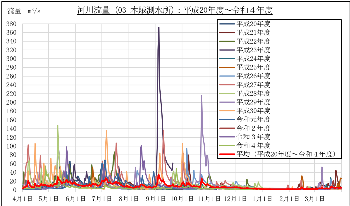
図 2-1-2(3) 流量計測結果 (流量 (常時計測箇所)) : 03 木賊測水所
