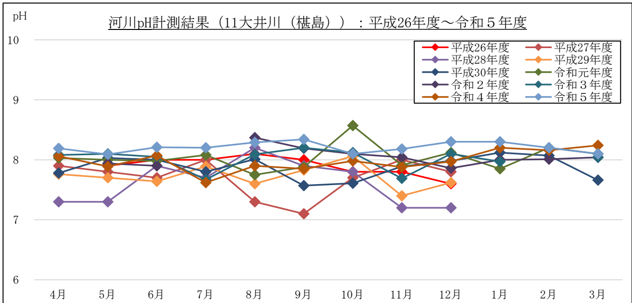
図 2-1-8(7) pH計測結果（流量（月1回計測箇所））：11 大井川（樫島）
