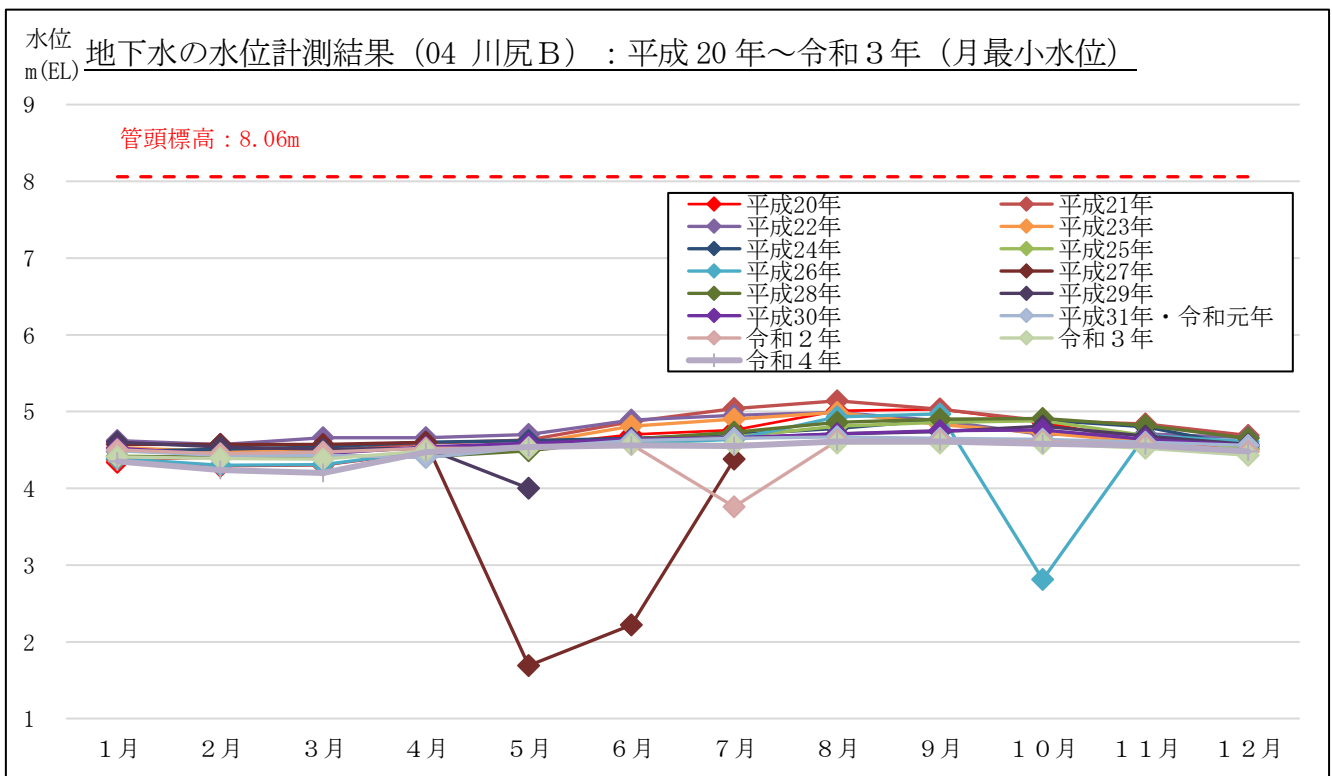
図 3-2-2(8) 地下水の水位計測結果 (月最小水位) : 04 川尻B (吉田町川尻)
