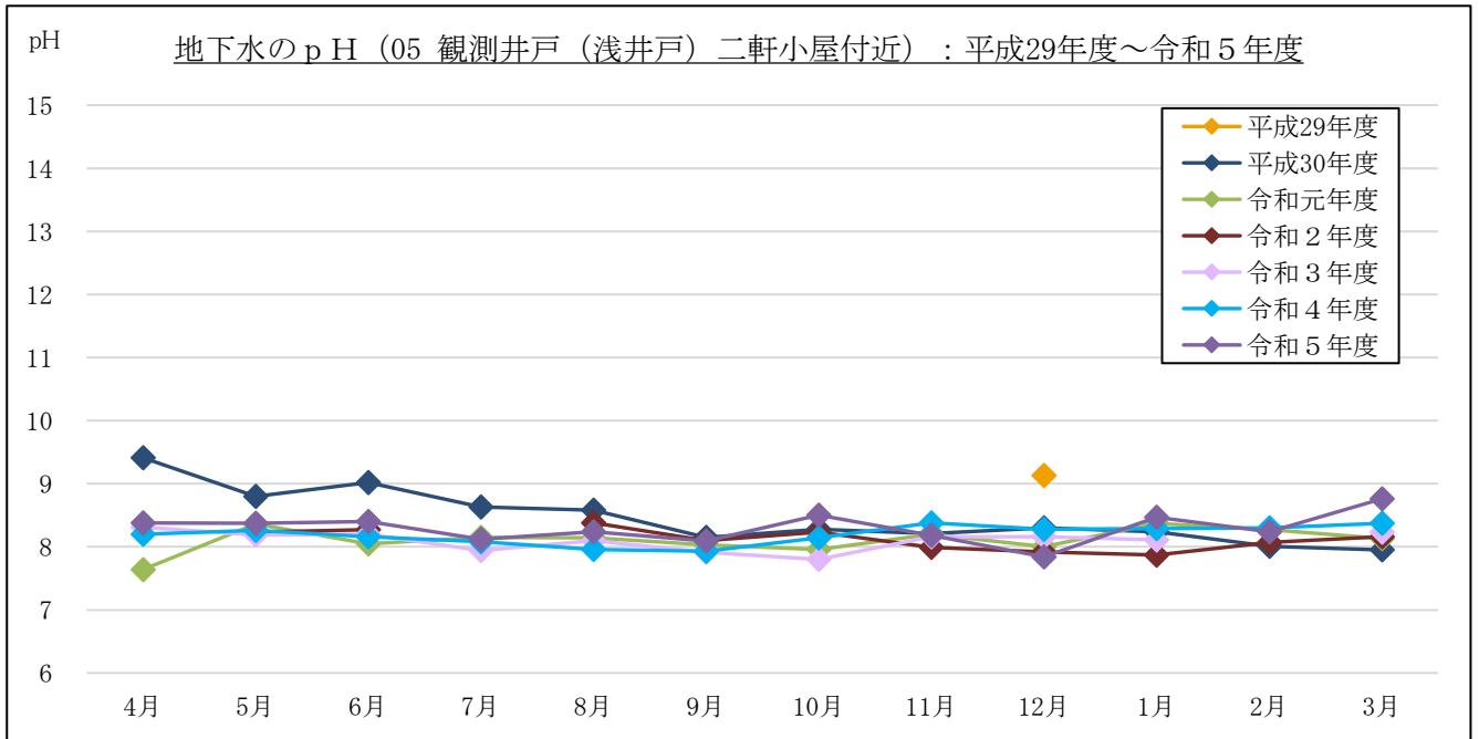
図 3-1-4(7) 地下水のpH計測結果 : 05 観測井戸 (浅井戸) 二軒小屋付近
