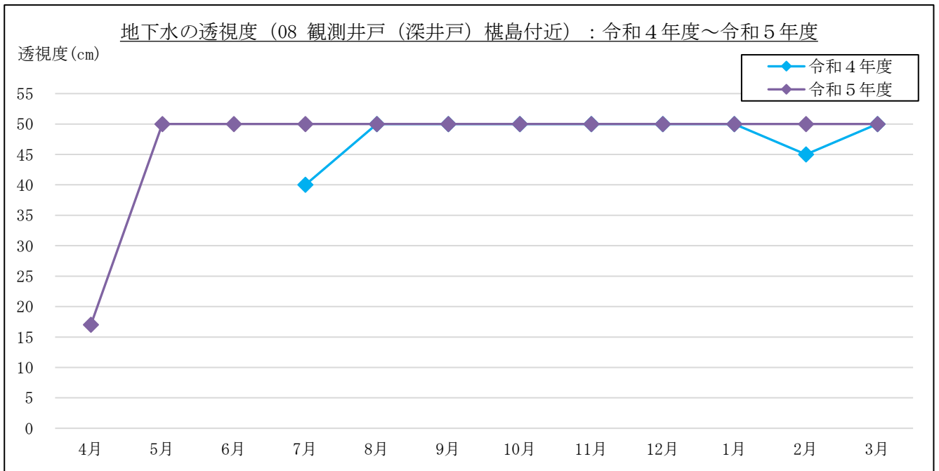
図 3-1-6(11) 地下水の透視度計測結果：08 観測井戸（深井戸）榎島付近
