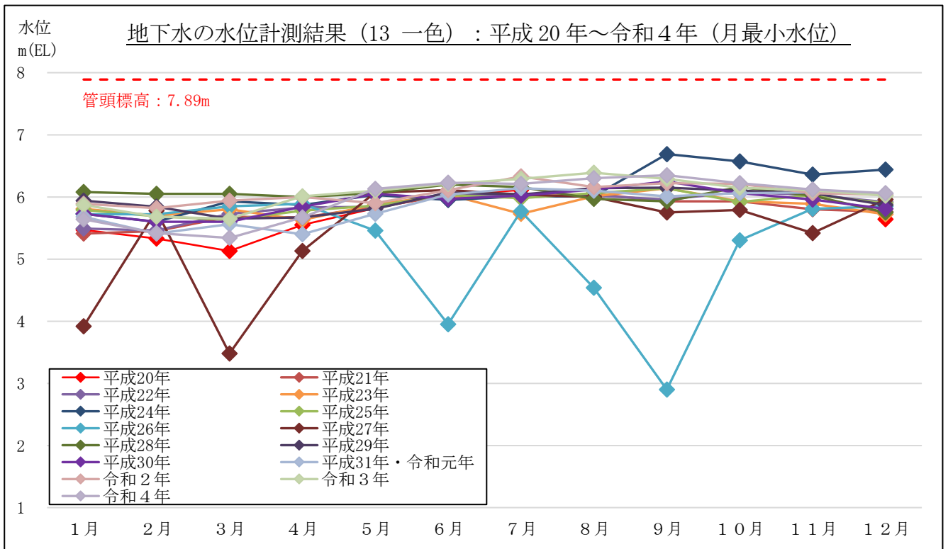
図 3-2-2(26) 地下水の水位計測結果 (月最小水位) : 13 一色 (焼津市一色)
