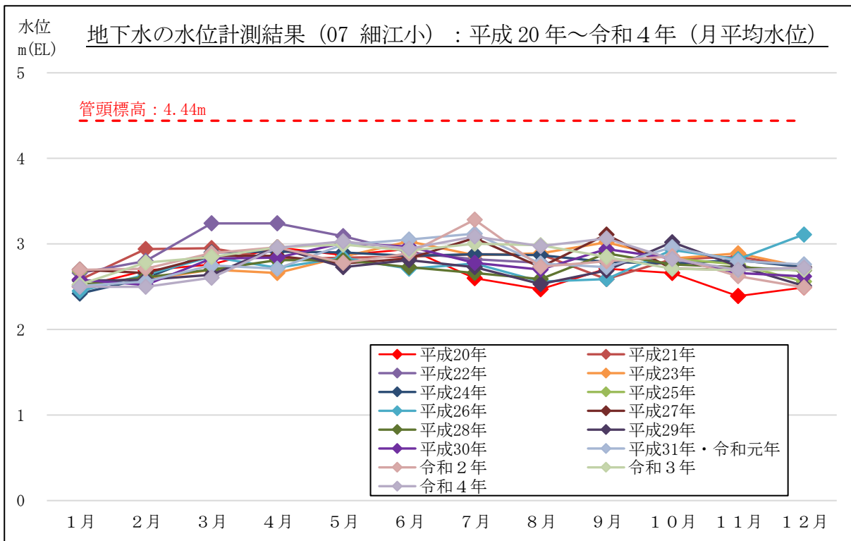
図 3-2-2(13) 地下水の水位計測結果 (月平均水位) : 07 細江小 (牧之原市細江)
