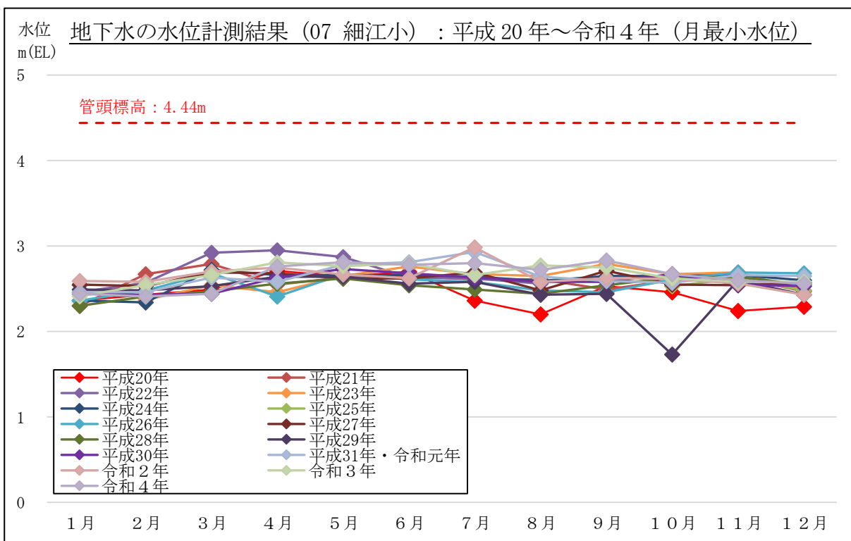
図 3-2-2(14) 地下水の水位計測結果 (月最小水位) : 07 細江小 (牧之原市細江)
