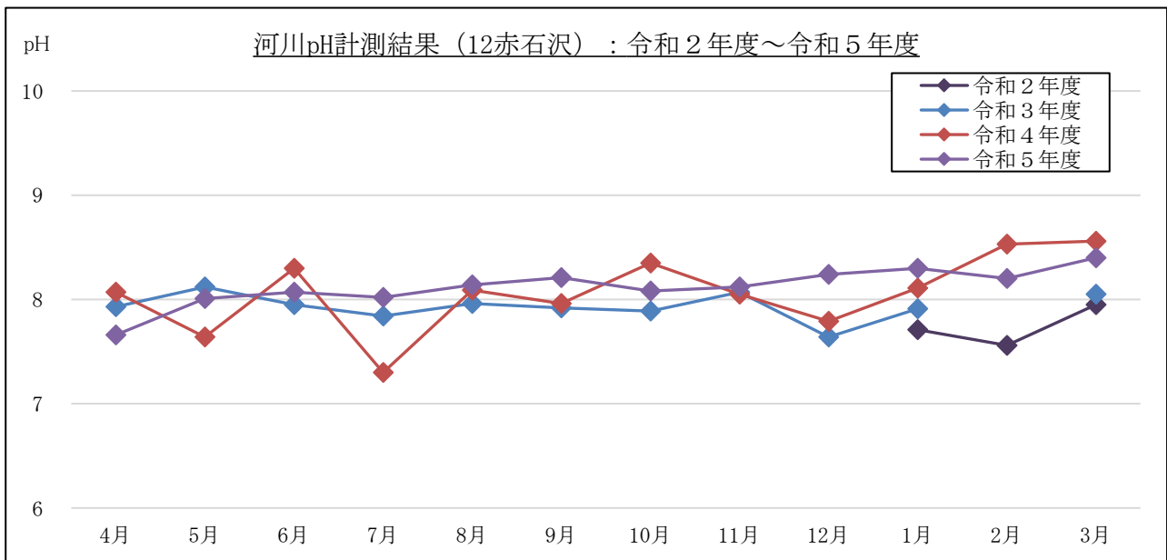
図 2-1-8(8) pH計測結果（流量（月1回計測箇所））：12 赤石沢
