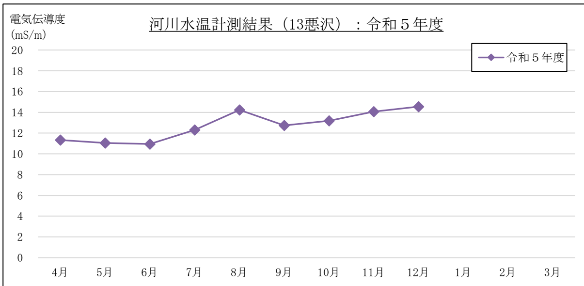
図 2-1-9(9) 電気伝導度計測結果 (流量 (月1回計測箇所)) : 13 悪沢
