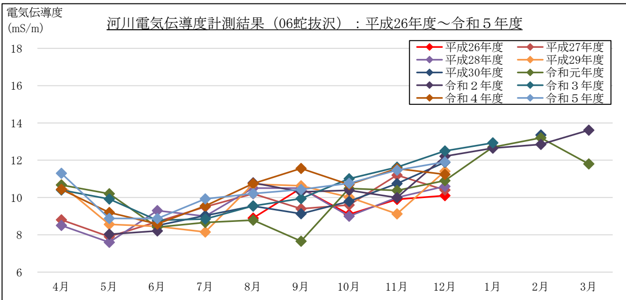
図 2-1-9(2) 電気伝導度計測結果 (流量 (月1回計測箇所)) : 06 蛇抜沢
