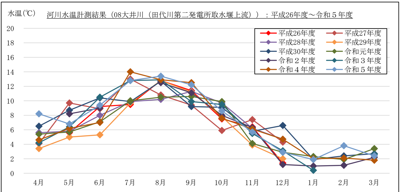
図 2-1-7(4) 水温計測結果 (流量 (月1回計測箇所)) : 08 大井川 (田代川第二発電所上流)
