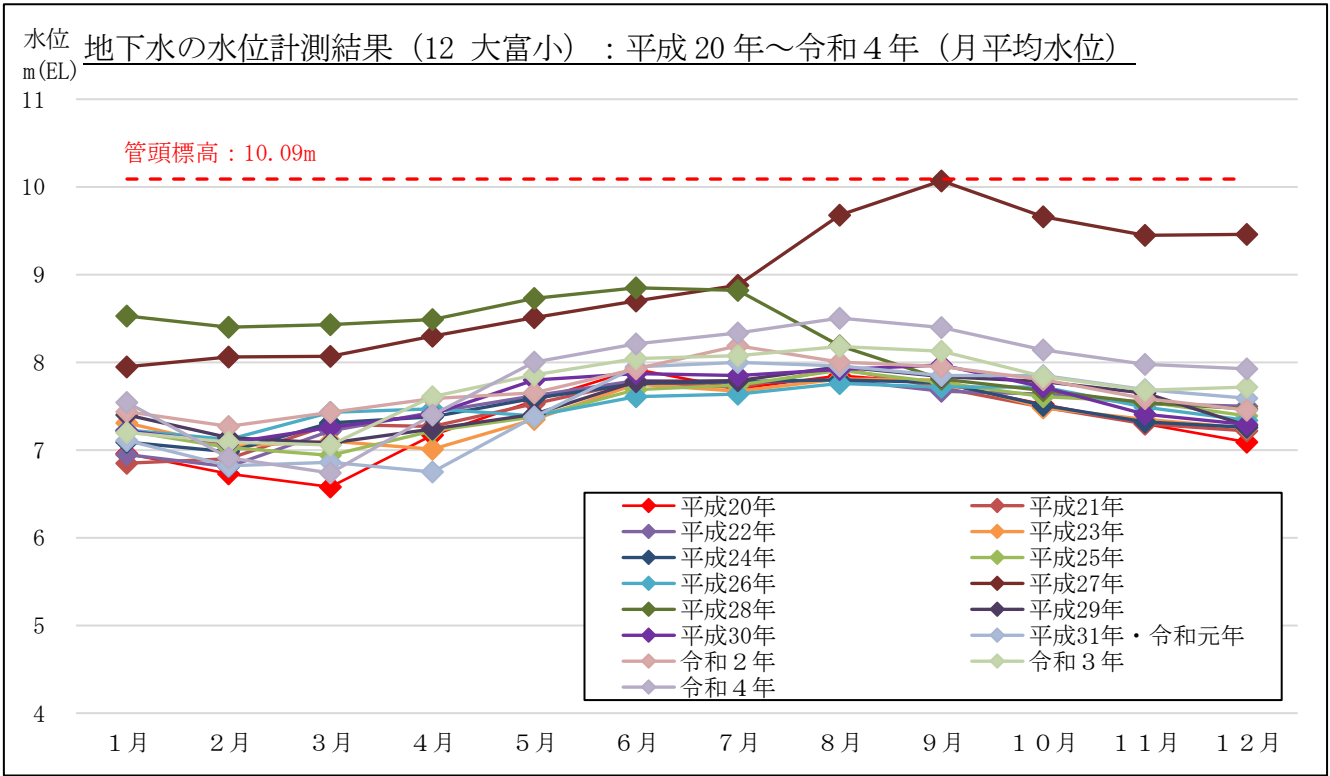
図 3-2-2(23) 地下水の水位計測結果 (月平均水位) : 12 大富小 (烧津市中根新田)
