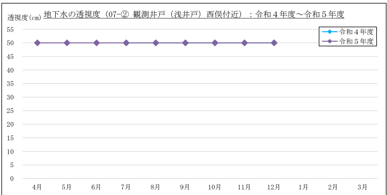
図 3-1-6(10) 地下水の透視度計測結果 : 07-② 観測井戸 (浅井戸) 西俣付近
