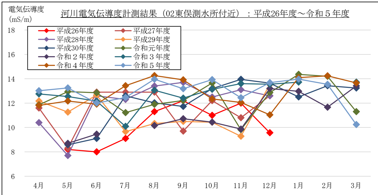
図 2-1-5(2) 電気伝導度計測結果 (流量 (常時計測箇所)) : 02 東俣第一測水所付近
