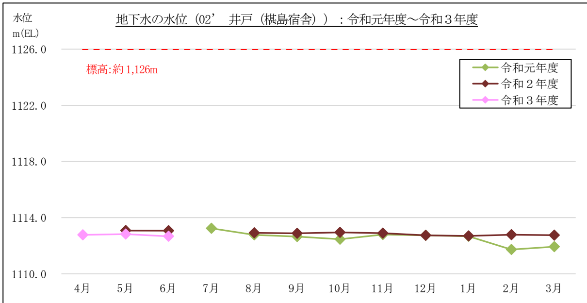
図 3-1-2(3) 地下水の水位計測結果 (月1回計測) : 02' 井戸 (榎島宿舎)
