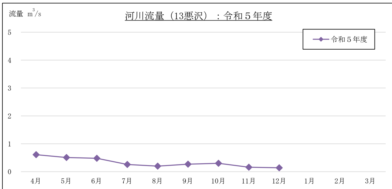
図 2-1-6(9) 流量計測結果 (流量 (月1回計測箇所)) : 13 悪沢
