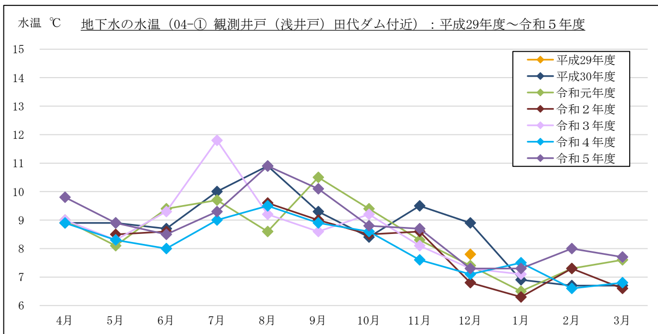
図 3-1-3(5) 地下水の水温計測結果 : 04-① 観測井戸 (浅井戸) 田代ダム付近
