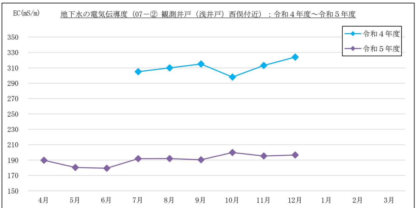
図 3-1-5 (10) 地下水の電気伝導度計測結果 : 07-② 観測井戸 (浅井戸) 西俣付近
