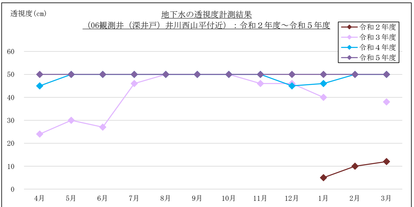
図 3-1-6(8) 地下水の透視度計測結果 : 06 観測井戸 (深井戸) 井川西山平付近
