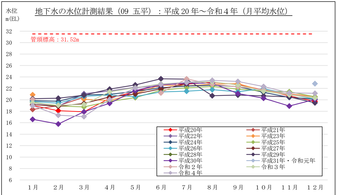
図 3-2-2(17) 地下水の水位計測結果 (月平均水位) : 09 五平 (藤枝市大西町)
