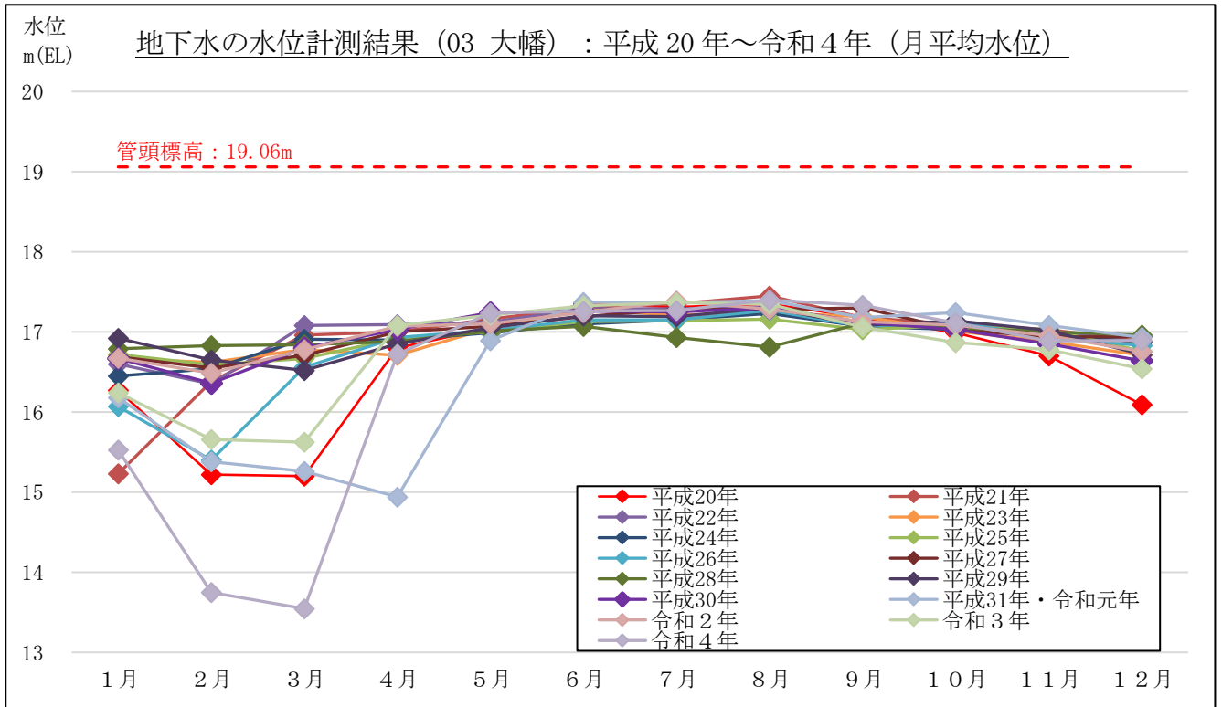
図 3-2-2(5) 地下水の水位計測結果 (月平均水位) : 03 大幡 (吉田町大幡)
