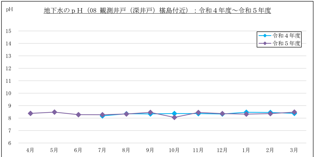
図 3-1-4(11) 地下水のpH計測結果：08 観測井戸（深井戸）榎島付近
