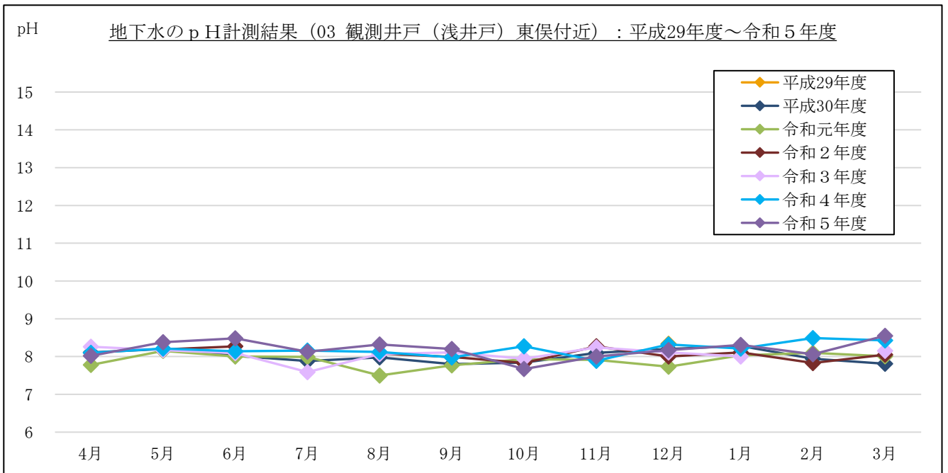
図 3-1-4(4) 地下水のpH計測結果 : 03 観測井戸 (浅井戸) 東俣付近
