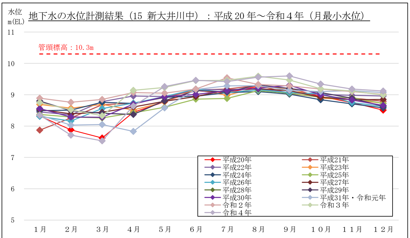
図 3-2-2(30) 地下水の水位計測結果 (月最小水位) : 15 新大井川中 (焼津市下江留)
