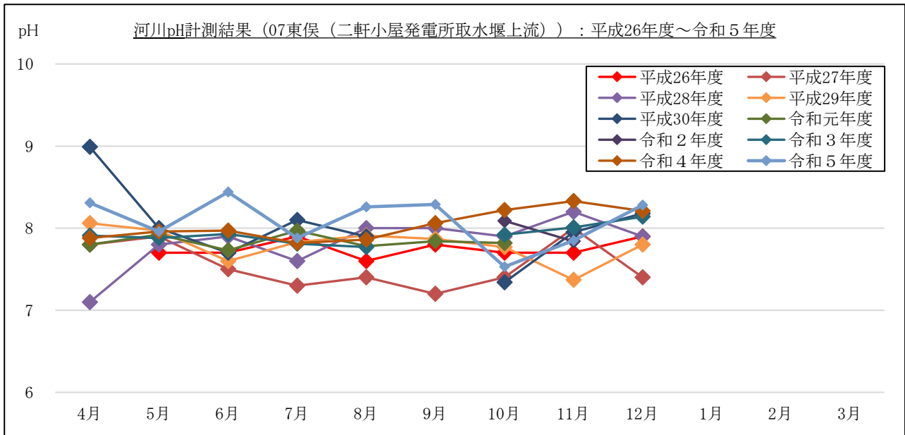
図 2-1-8(3) pH計測結果（流量（月1回計測箇所））：07 東俣（二軒小屋発電所取水堰上流）
