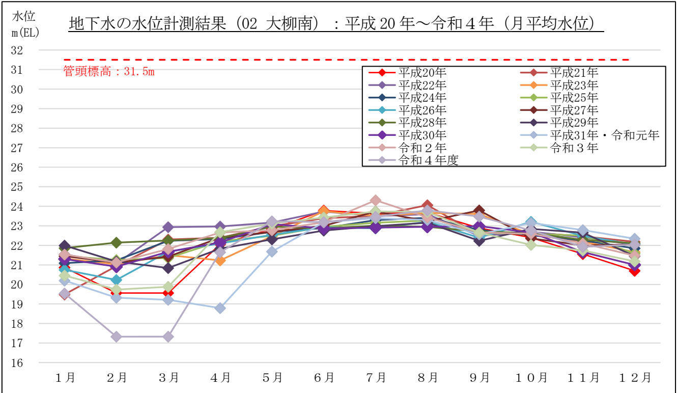
図 3-2-2(3) 地下水の水位計測結果 (月平均水位) : 02 大柳南 (島田市大柳)
