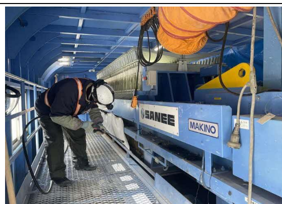
写真4-1-74 濁水処理設備の整備状況
