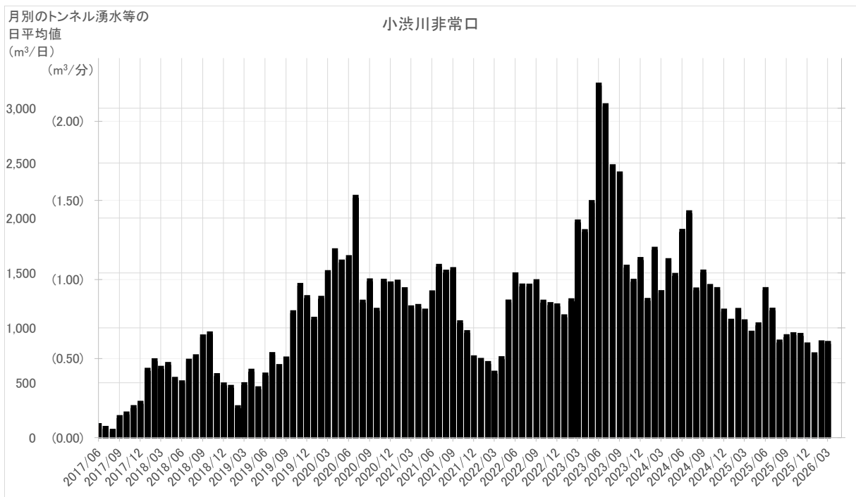
図 参 1-3 小渋川非常口工事施工ヤードのトンネル湧水等の状況
