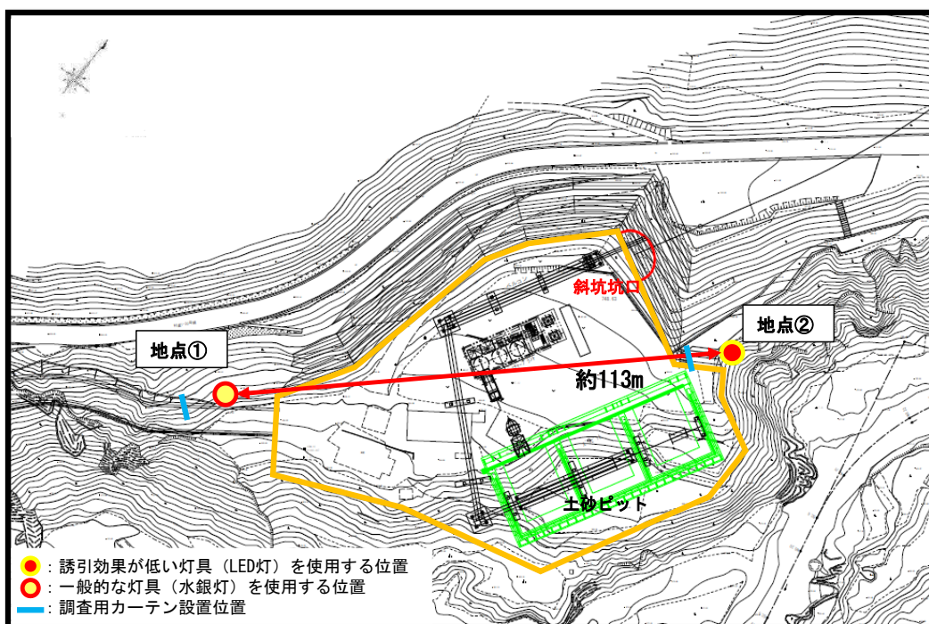
図 2-2-1 灯具配置図
