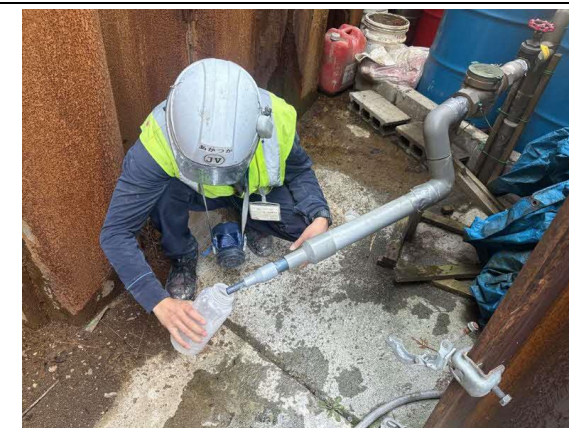
写真4-1-140 地下水等の監視状況
