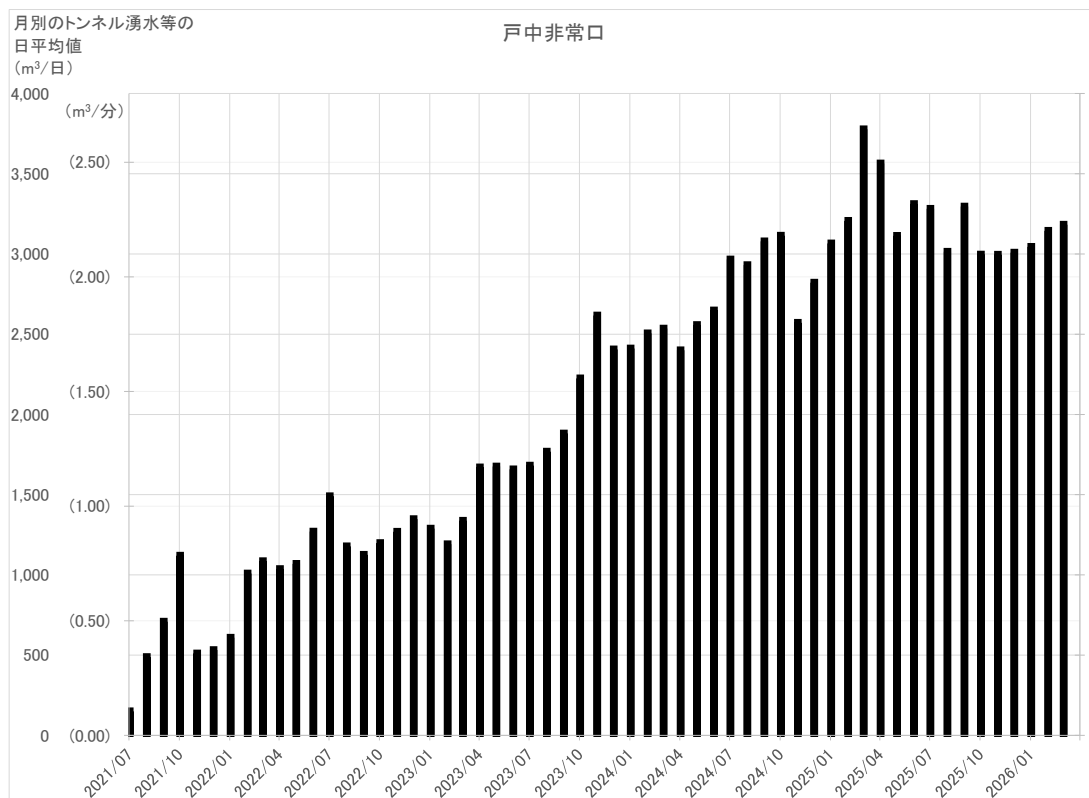
図 参 1-6 戸中非常口工事施工ヤードのトンネル湧水等の状況
