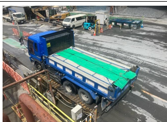
写真4-1-22 荷台への防じんシート敷設
