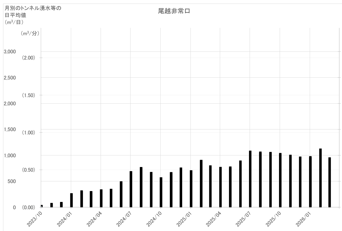
図 参 1-10 尾越非常口工事施工ヤードのトンネル湧水等の状況
