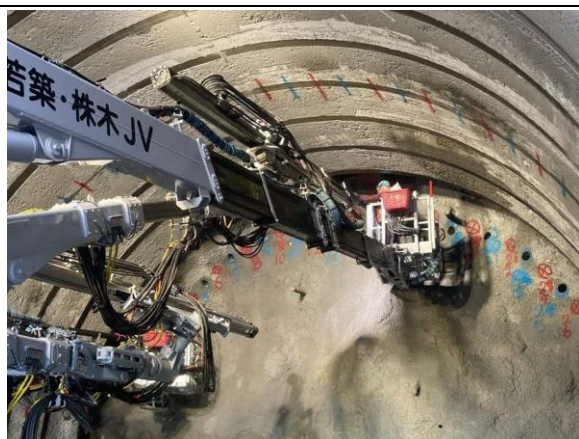
写真4-1-179 補助工法の実施状況
