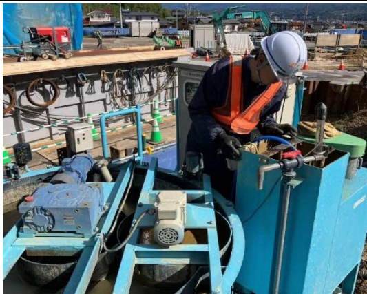
写真4-1-127 工事排水の監視
