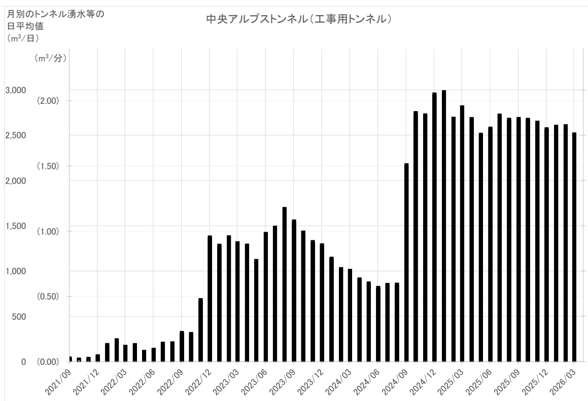
図 参 1-7 黒田非常口工事施工ヤードのトンネル湧水等の状況
