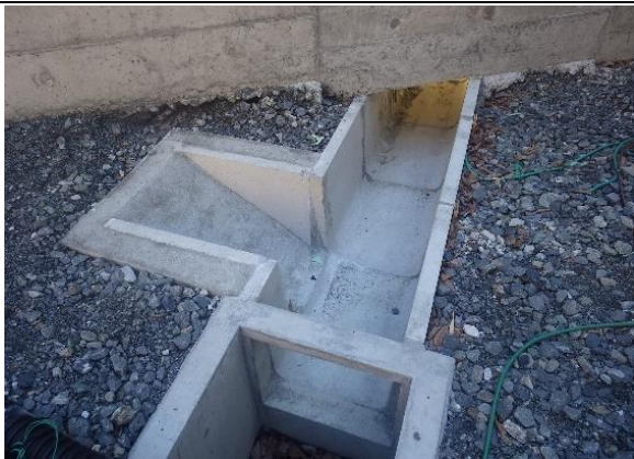
写真4-1-15 小動物等の移動経路の確保 (幅約50cmのスロープを設置)
