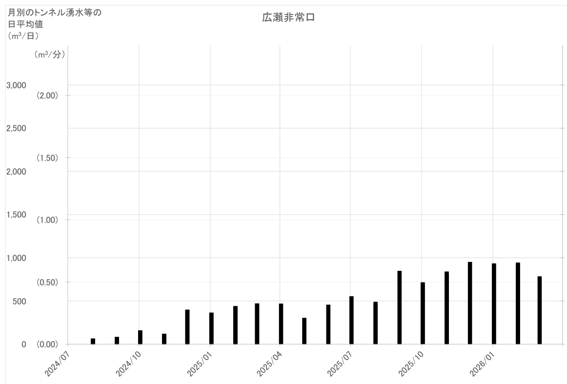
図 参 1-9 広瀬非常口工事施工ヤードのトンネル湧水等の状況
