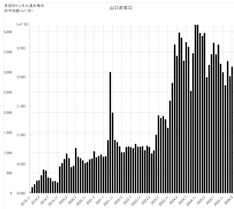
図 参 3-2-1-1 山口非常口工事施工ヤードのトンネル湧水等の状況
