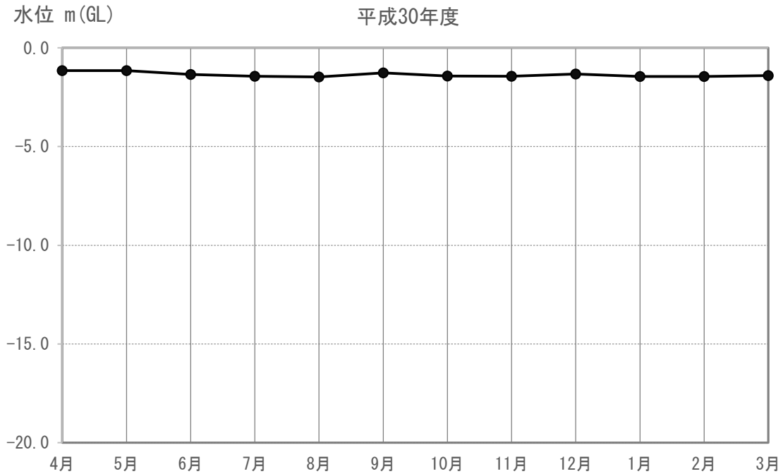
図 4-1-4-1 (32) 地下水の水位 (又は水量) の現地調査結果 (K-01)
