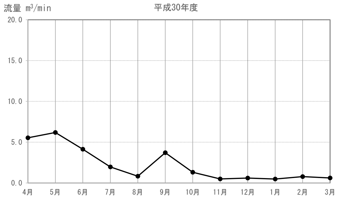
図 4-1-4-2(25) 河川の流量の現地調査結果 (T-05)
