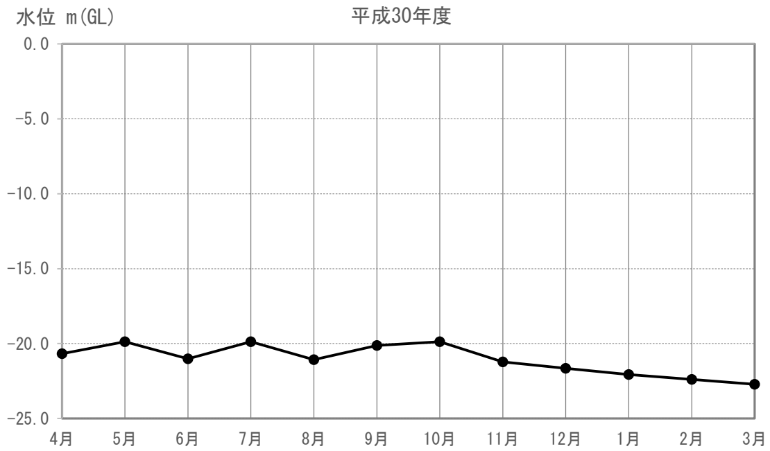
図 4-1-4-1 (35) 地下水の水位 (又は水量) の現地調査結果 (T-01)
