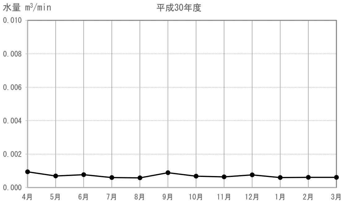
図 4-1-4-1 (26) 地下水の水位 (又は水量) の現地調査結果 (M-04)
