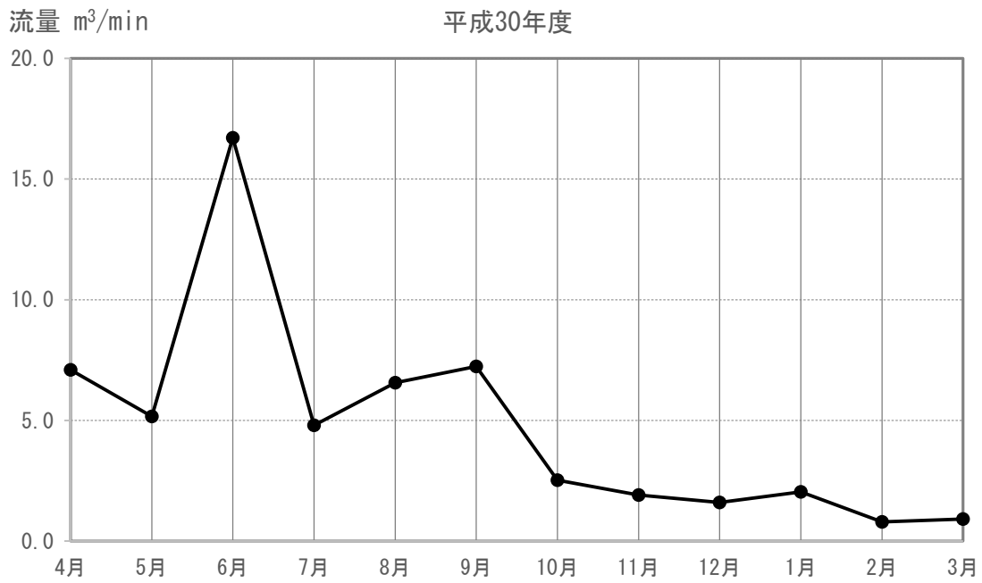
図 4-1-4-2 (23) 河川の流量の現地調査結果 (K-06)
