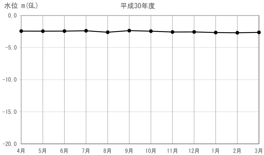
図 4-1-4-1 (25) 地下水の水位 (又は水量) の現地調査結果 (M-03)
