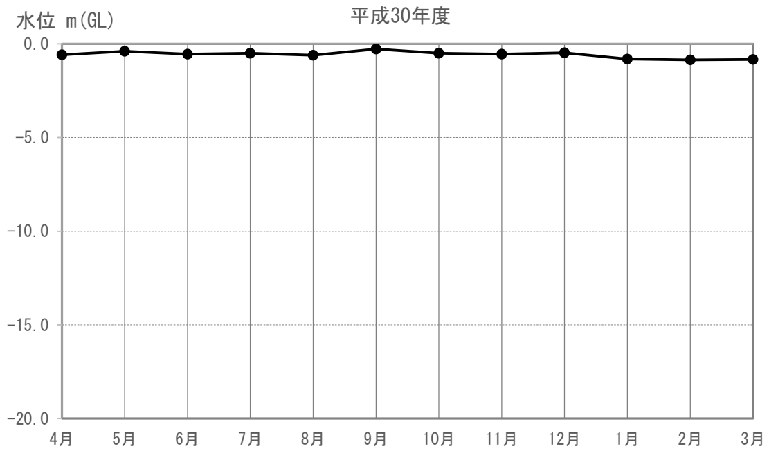
図 4-1-4-1 (31) 地下水の水位 (又は水量) の現地調査結果 (M-09)
