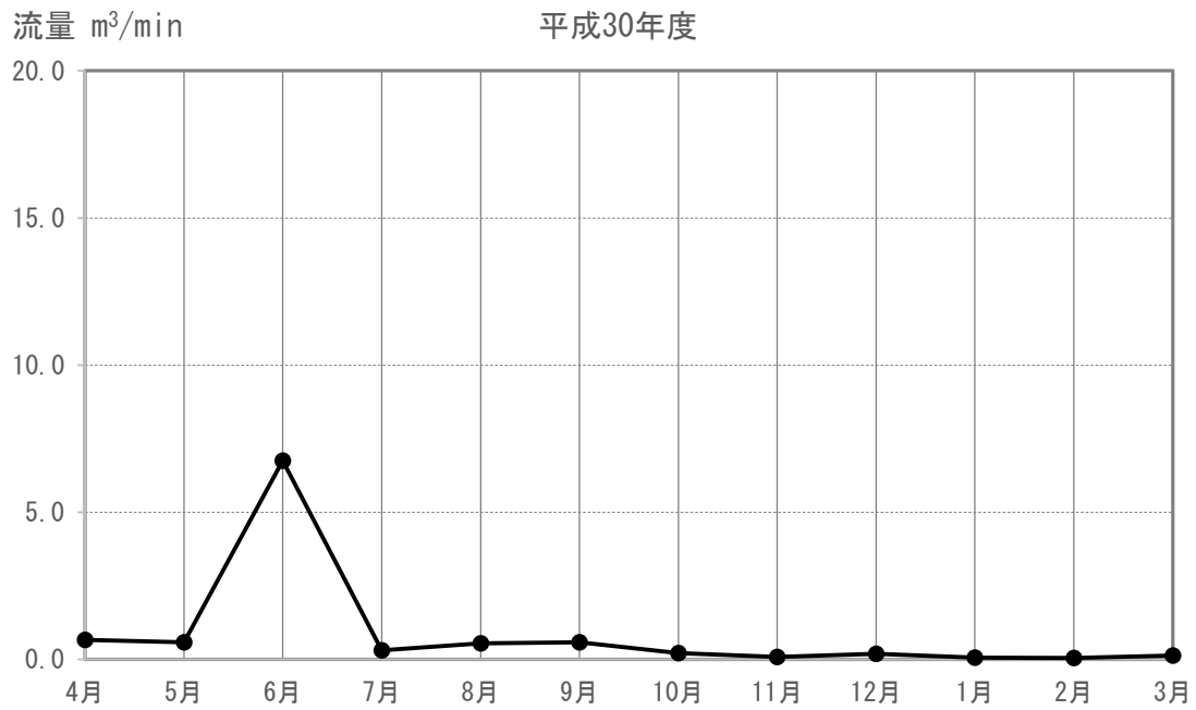
図 4-1-4-2(14) 河川の流量の現地調査結果 (M-12)
