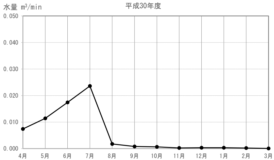
図 4-1-4-1(28) 地下水の水位（又は水量）の現地調査結果（M-06）
