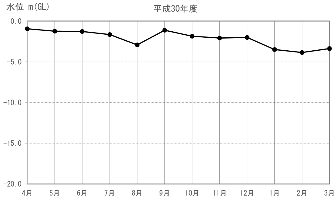
図 4-1-4-1 (36) 地下水の水位 (又は水量) の現地調査結果 (T-02)
