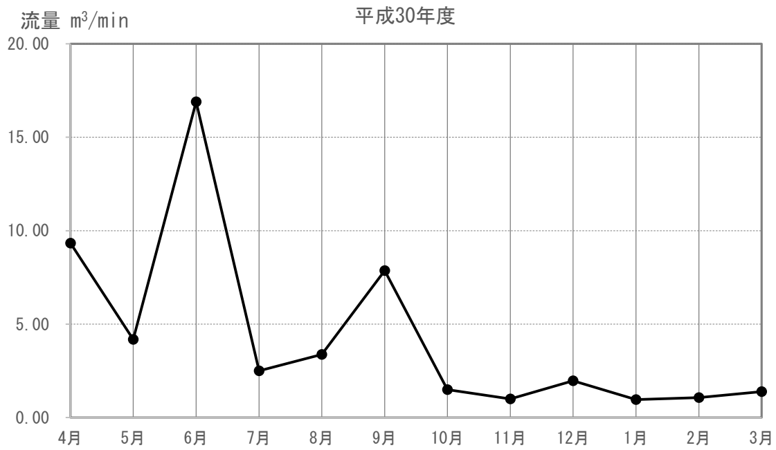
図 4-1-4-2(15) 河川の流量の現地調査結果 (M-13)
