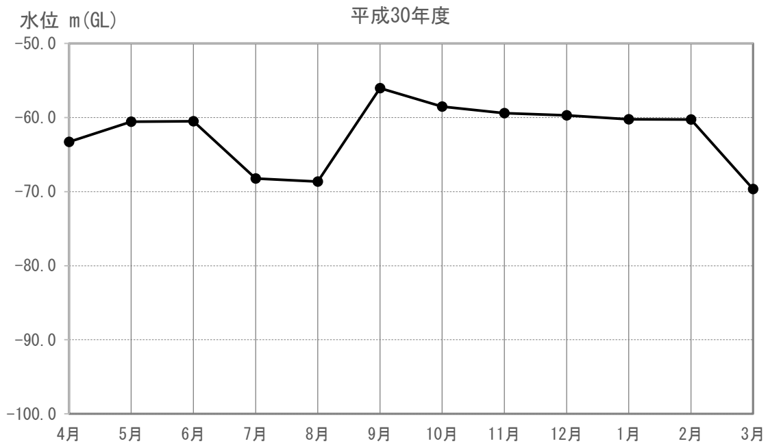
図 4-1-4-1(29) 地下水の水位（又は水量）の現地調査結果（M-07）
