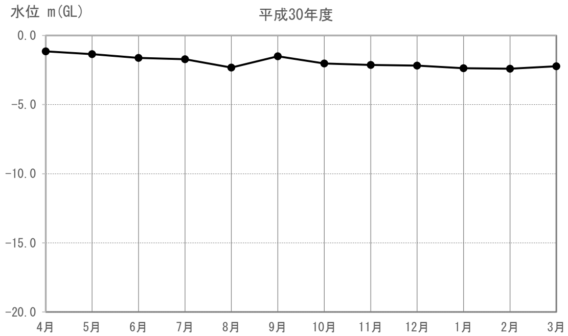
図 4-1-4-1 (33) 地下水の水位 (又は水量) の現地調査結果 (K-02)
