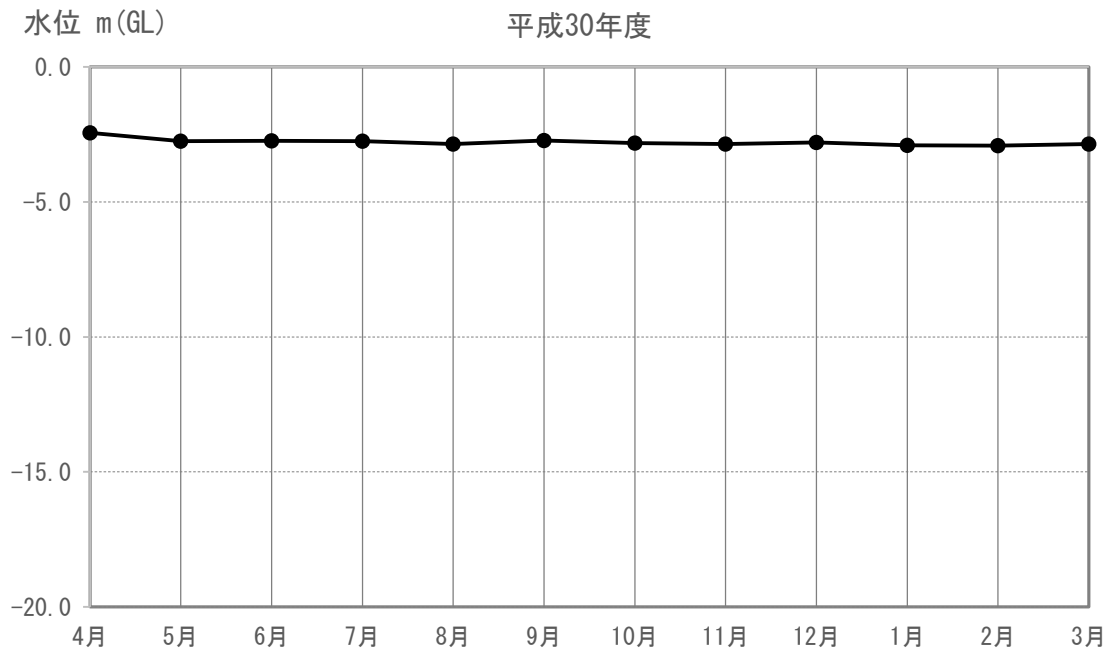
図 4-1-4-1 (34) 地下水の水位 (又は水量) の現地調査結果 (K-03)
