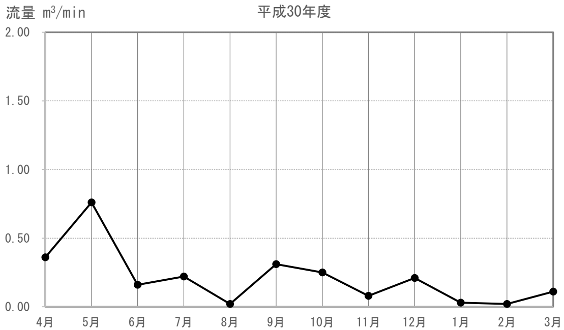
図 4-1-4-2(12) 河川の流量の現地調査結果 (M-10)
