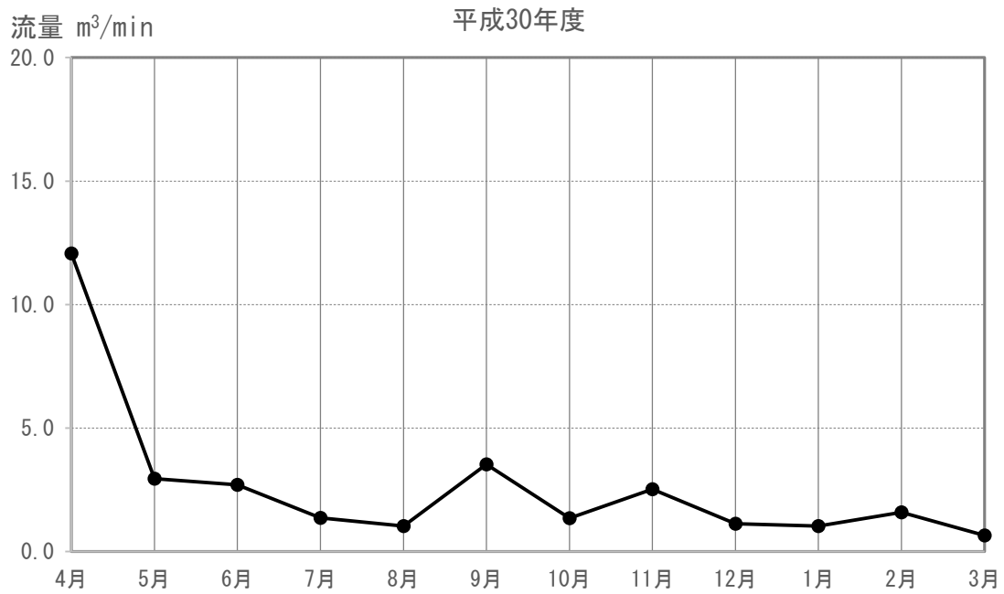
図 4-1-4-2(18) 河川の流量の現地調査結果 (M-16)
