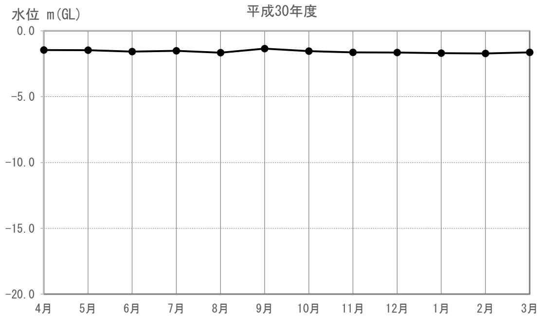
図 4-1-4-1(27) 地下水の水位（又は水量）の現地調査結果（M-05）
