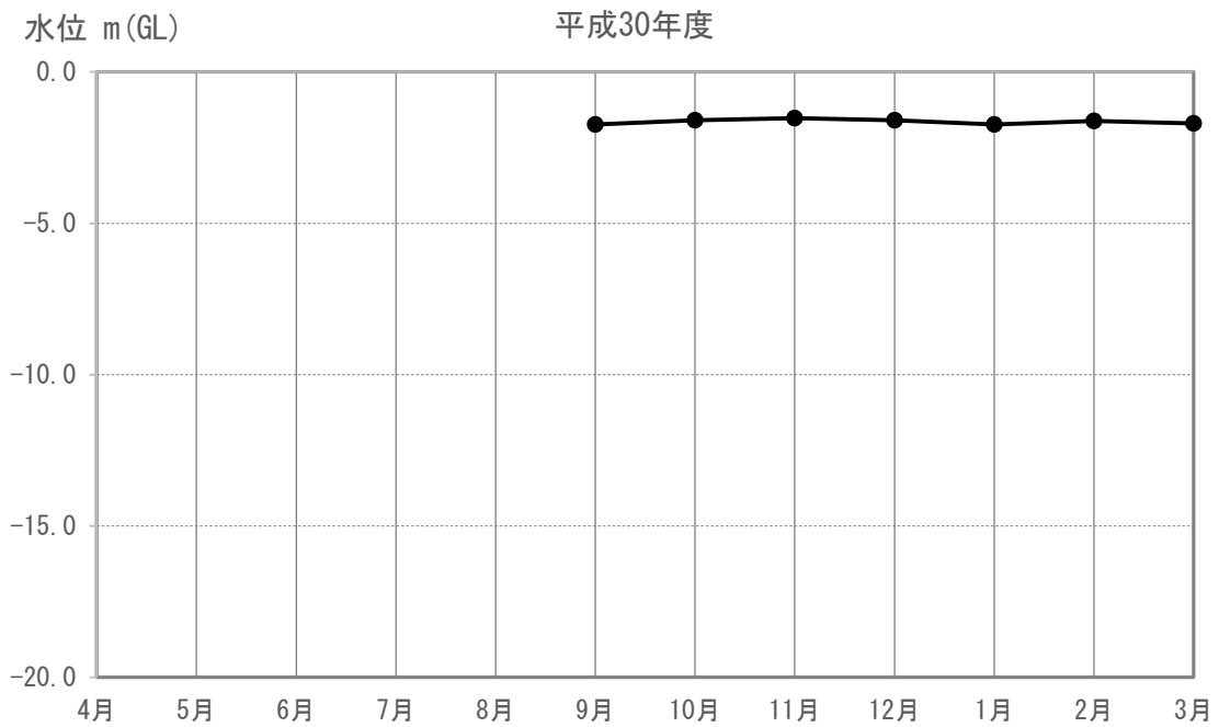
図 4-1-4-1 (20) 地下水の水位 (又は水量) の現地調査結果 (E-07)
