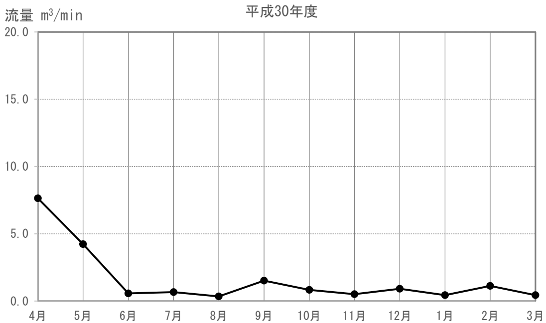
図 4-1-4-2(6) 河川の流量の現地調査結果 (N-19)
