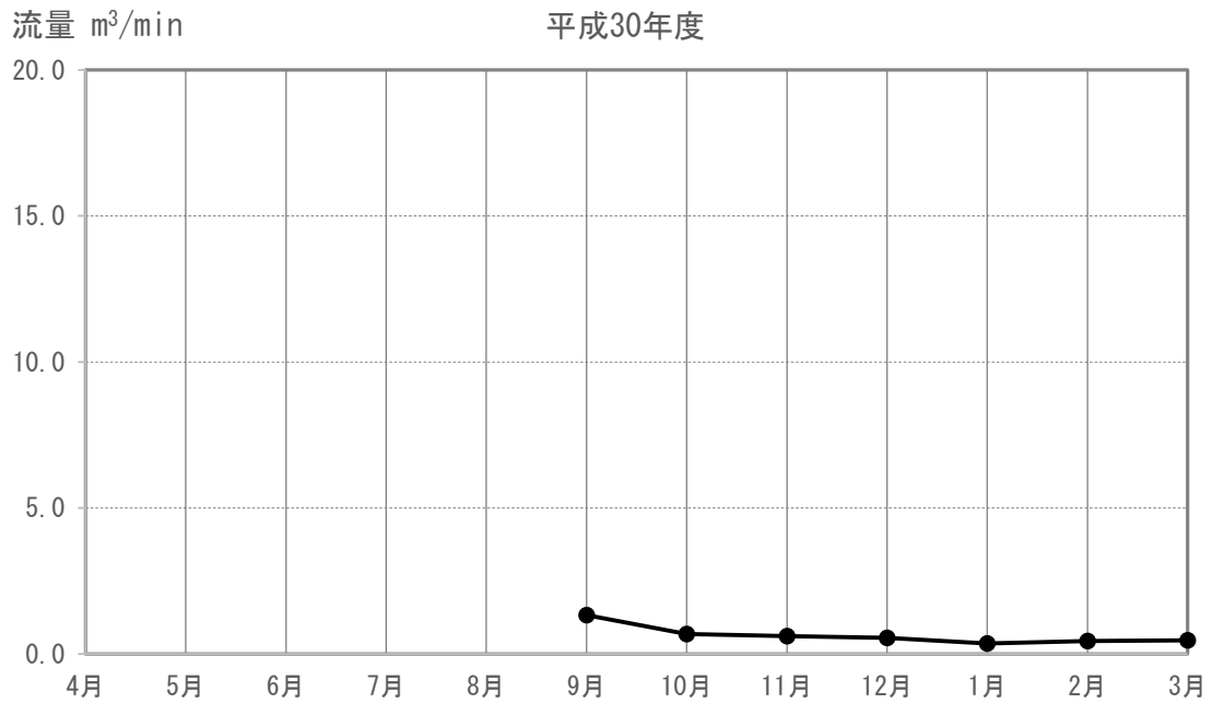
図 4-1-4-2(8) 河川の流量の現地調査結果 (E-09)
