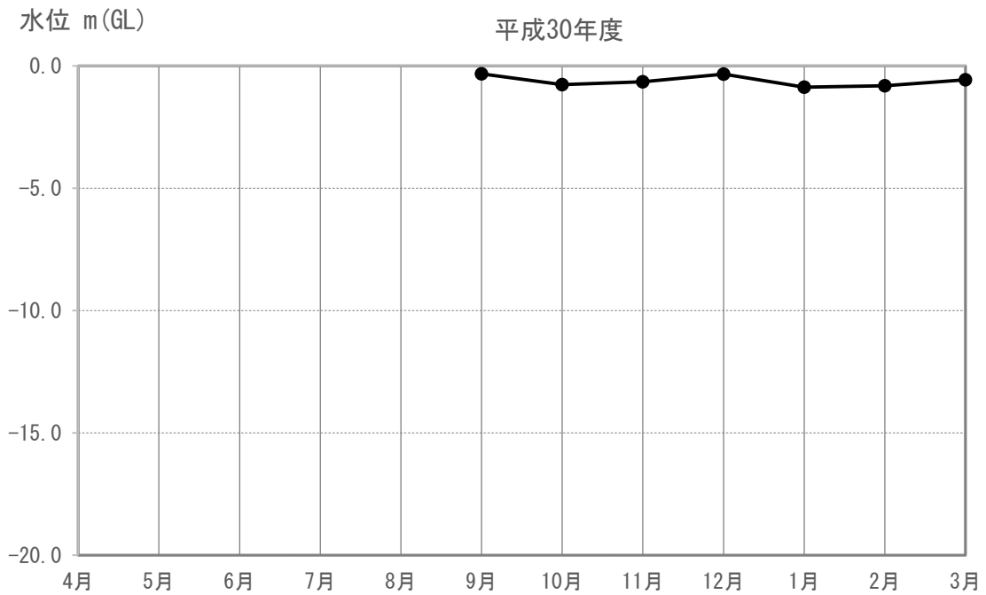
図 4-1-4-1(17) 地下水の水位（又は水量）の現地調査結果（E-04）
