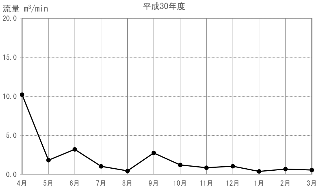
図 4-1-4-2(20) 河川の流量の現地調査結果 (M-18)
