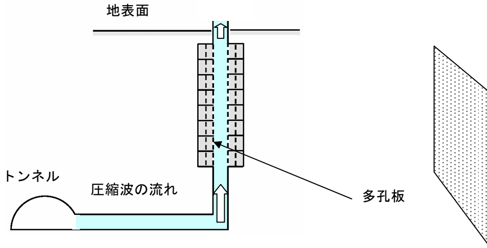
図 4-3-2-1 多孔板の構造
