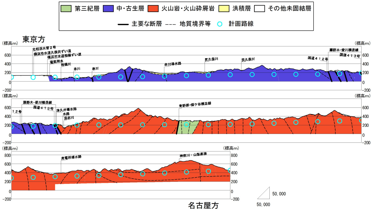
図 8-2-3-5 地質縦断面図
