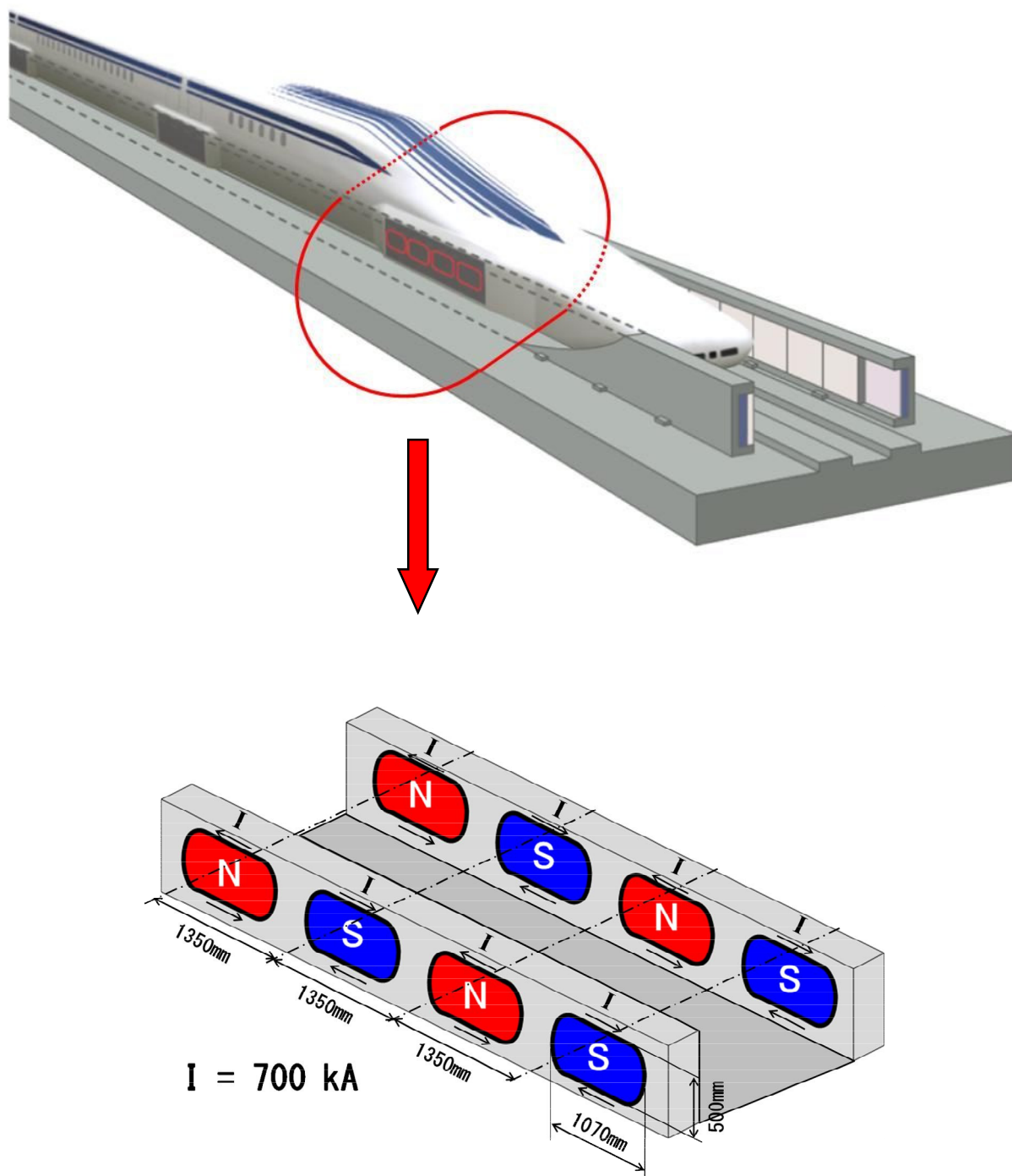
図 9-7-1-2 超電導磁石を拡大した概略図（磁界の算出にあたっての前提条件）
