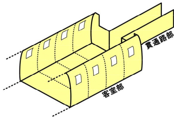
図 9-5-1 車内への磁気シールド設置の概念図
