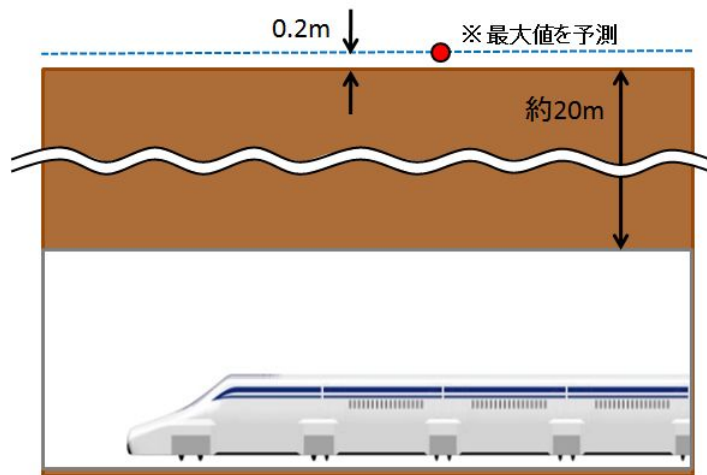
図 9-7-3-1 地上における磁界の算出位置イメージ（ケース 1）
