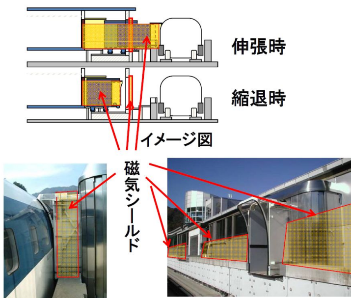
図 9-5-2 ホームへの磁気シールド設置の概念図
