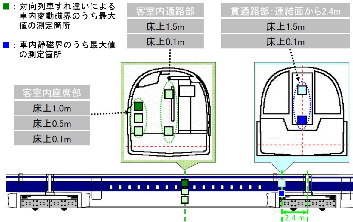
図 9-5-3 車内の磁界の測定箇所
