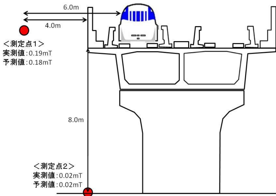
図 9-7-2-1 山梨リニア実験線における実測値と予測値の比較
