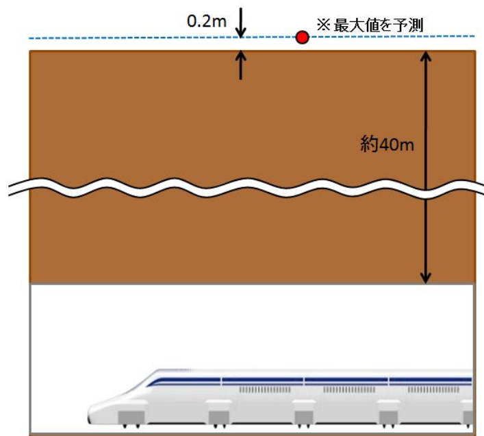
図 9-7-3-2 地上における磁界の算出位置イメージ（ケース 2）
