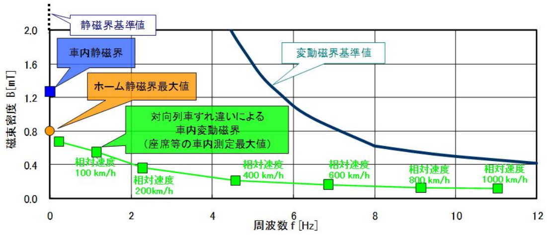
図 9-5-5 車内及びホームの磁界の測定結果
