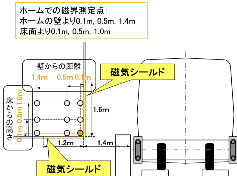
図 9-5-4 ホーム上の磁界の測定箇所
