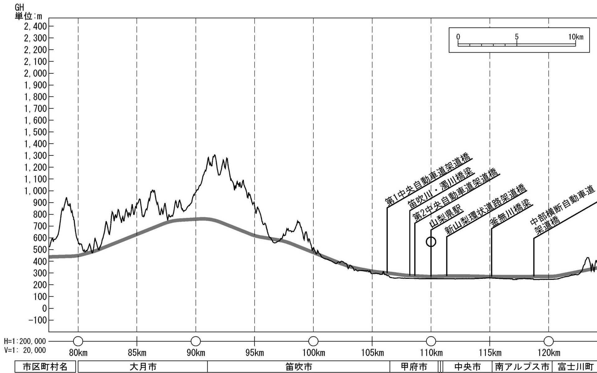
図 2-1(3) 路線概要 (縦断計画)
