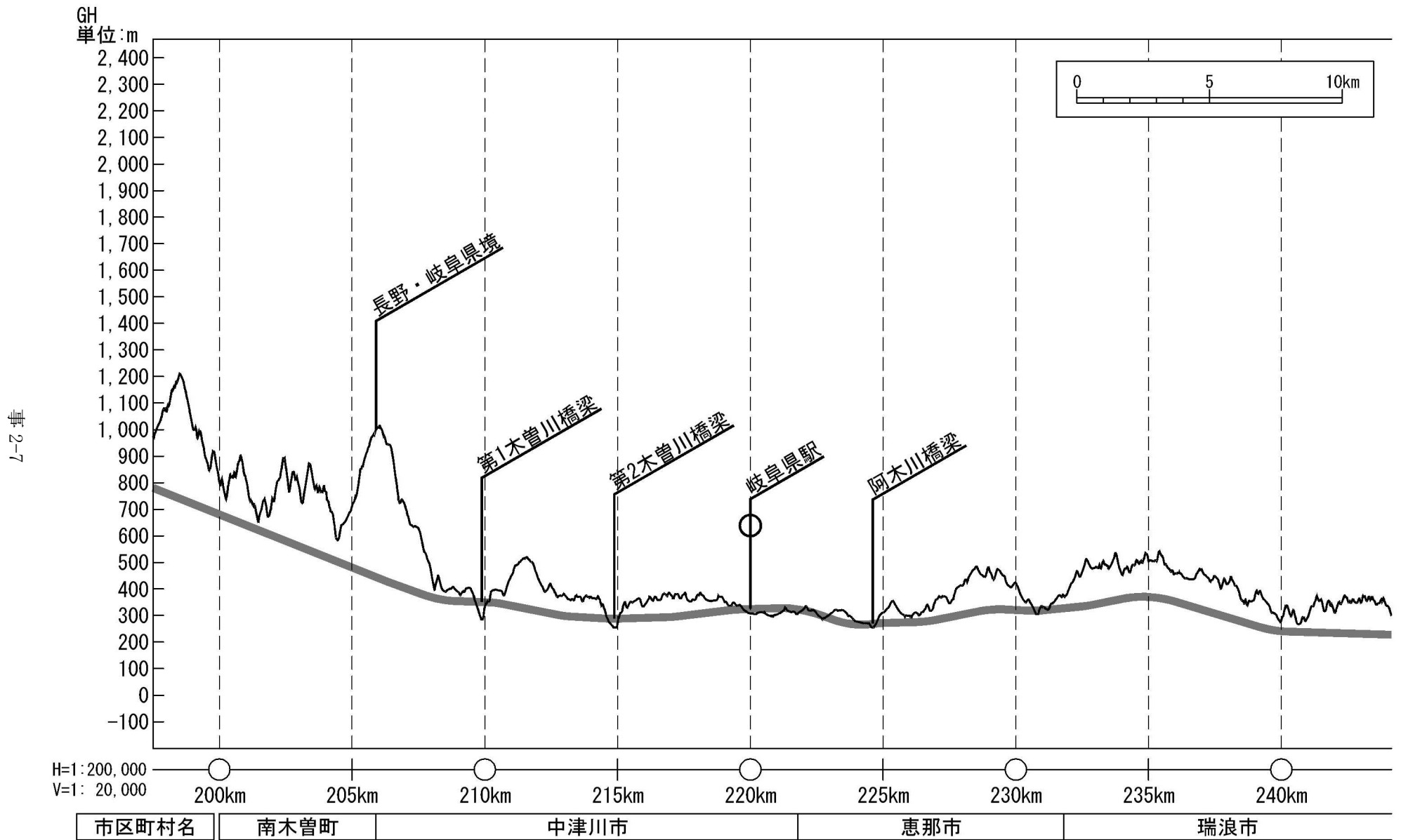
图 2-1(6) 路線概要(縦断計画)
