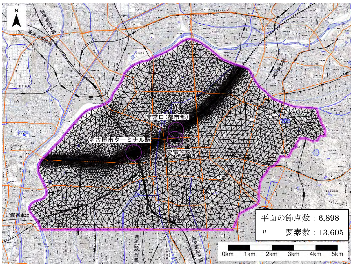
5-3-2-2 要素区分
