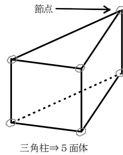
図 5-3-1-1 要素形状
