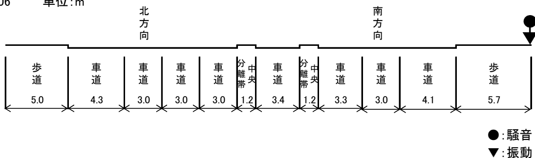
図 2-3-1(6) 調査地点断面図
