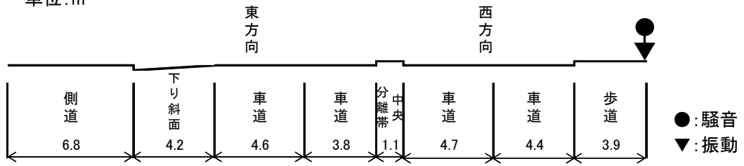
図 2-3-1(1) 調査地点断面図
