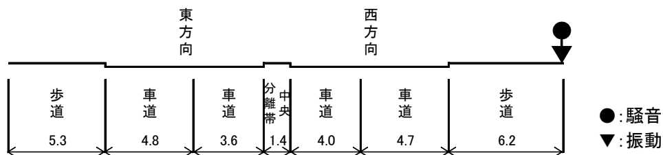
図 2-3-1(7) 調査地点断面図
