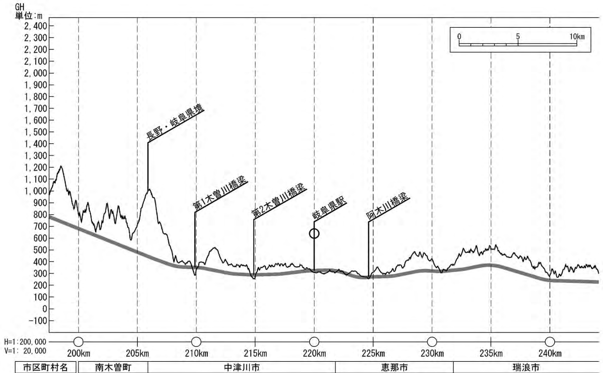
図 2-1(6) 路線概要(縦断計画)
