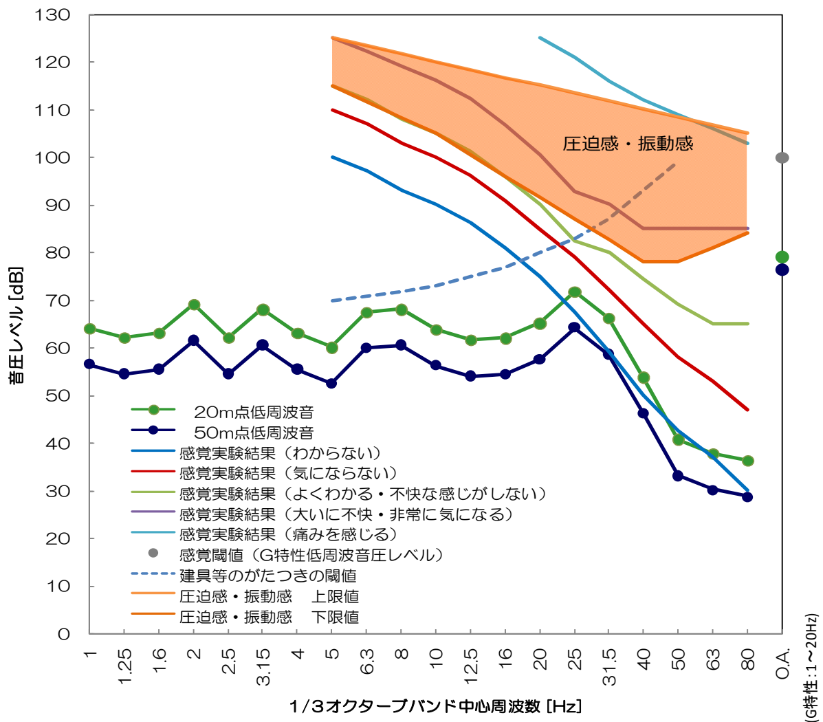
図 8-1-5-6(1) 非常口（都市部）、地下駅における換気施設の評価結果
