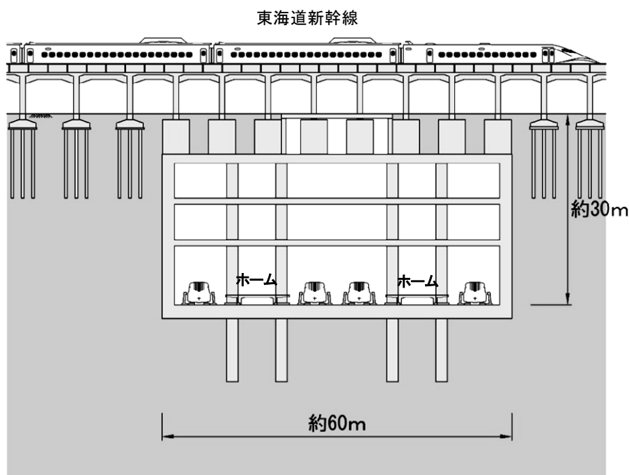
図 3-4-6-1 名古屋市ターミナル駅の概要
