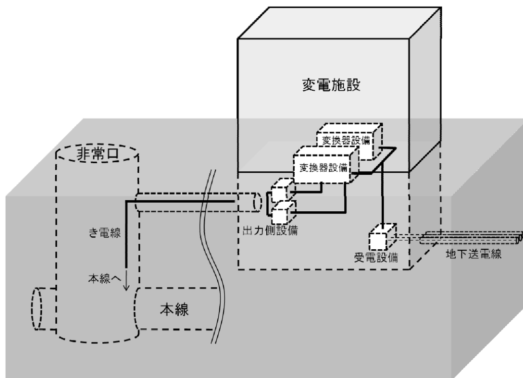
図 3-4-6-7 変電施設の概要
