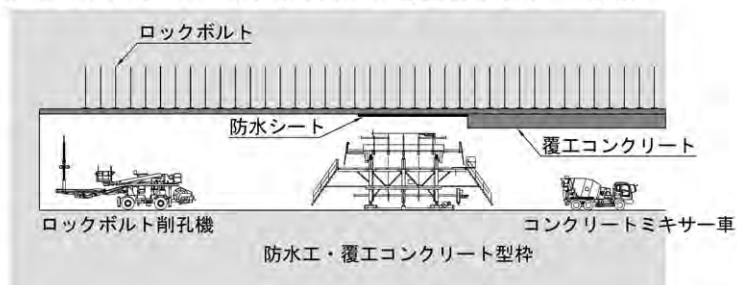
図 3-4-6-10 山岳トンネル部における施工概要
