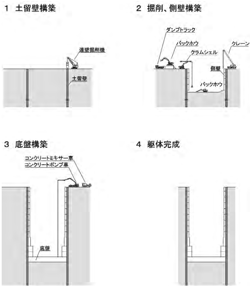
図 3-4-6-17 非常口の施工概要(RC 地中連続壁工法の場合)
