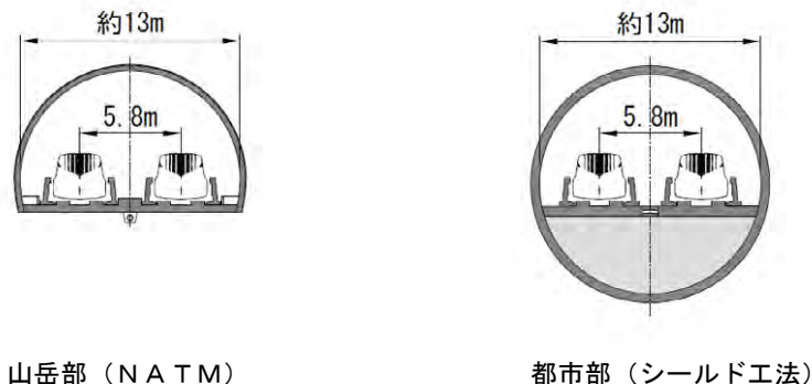
図 3-4-6-2 トンネルの標準的な断面図
