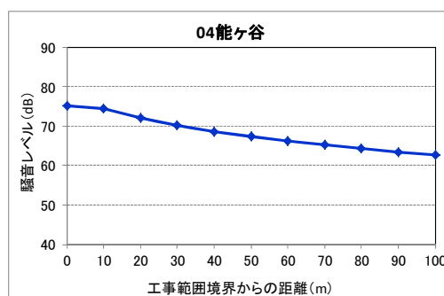
図 2-7-1-1 建設機械の稼働に係る騒音の距離減衰の状況
