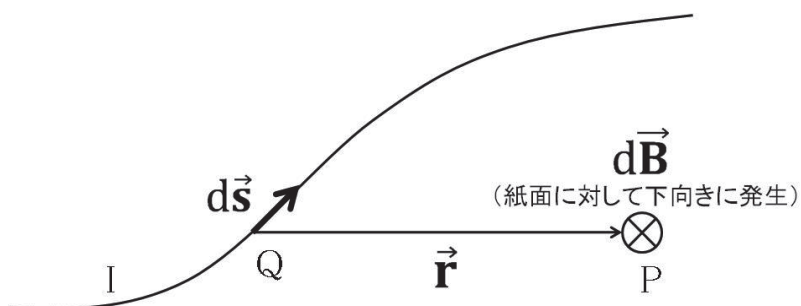
図 13-7-1 ビオ・サバルの法則概念図
