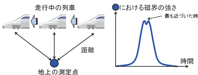
図 13-9-5 走行中の列車から発生する磁界のイメージ(超電導磁石が 1 つ通過する場合)
