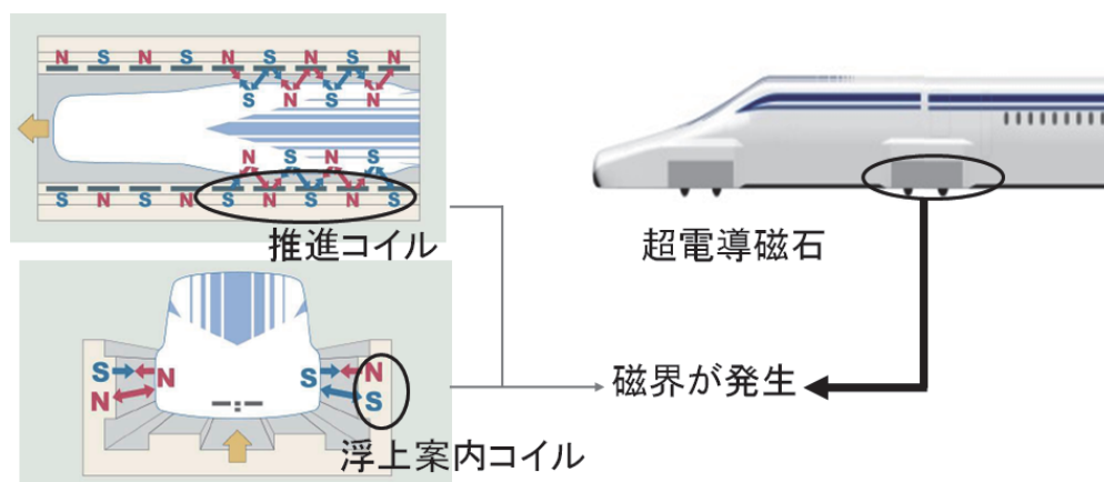
図 13-9-4 超電導リニアによる磁界の発生源
