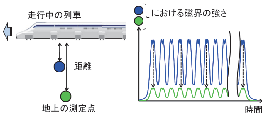
図 13-9-7 走行中の列車から発生する変動磁界のイメージ
