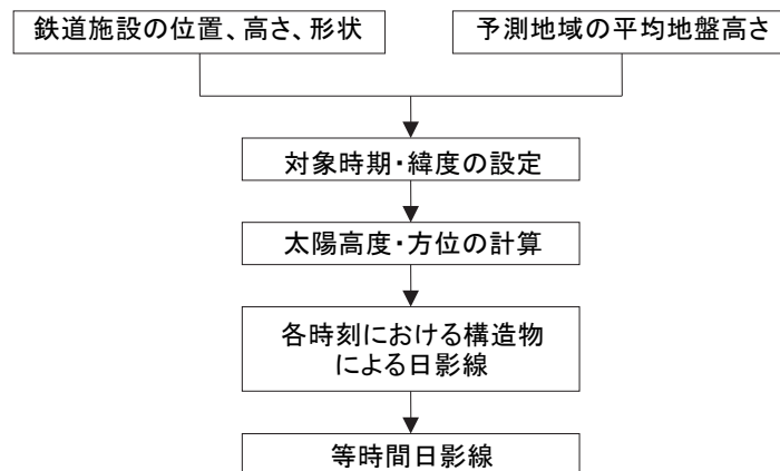
図 8-3-4-1 日照障害の予測手順
