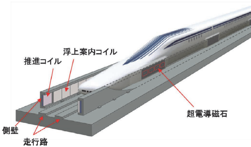
図 3-4-24 車両とガイドウェイの構成
