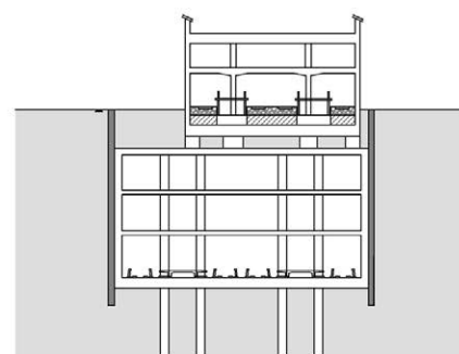
図 3-4-11 駅部における施工概要
