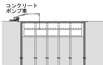
図 3-4-22 変電施設における施工概要
