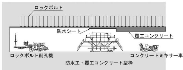
図 3-4-7 山岳トンネル部における施工概要
