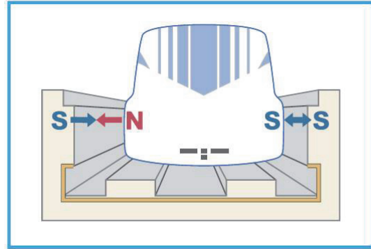
図 3-4-15 案内の原理
