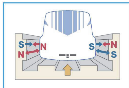
図 3-4-14 浮上の原理
