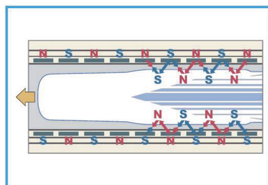
図 3-4-13 推進の原理
