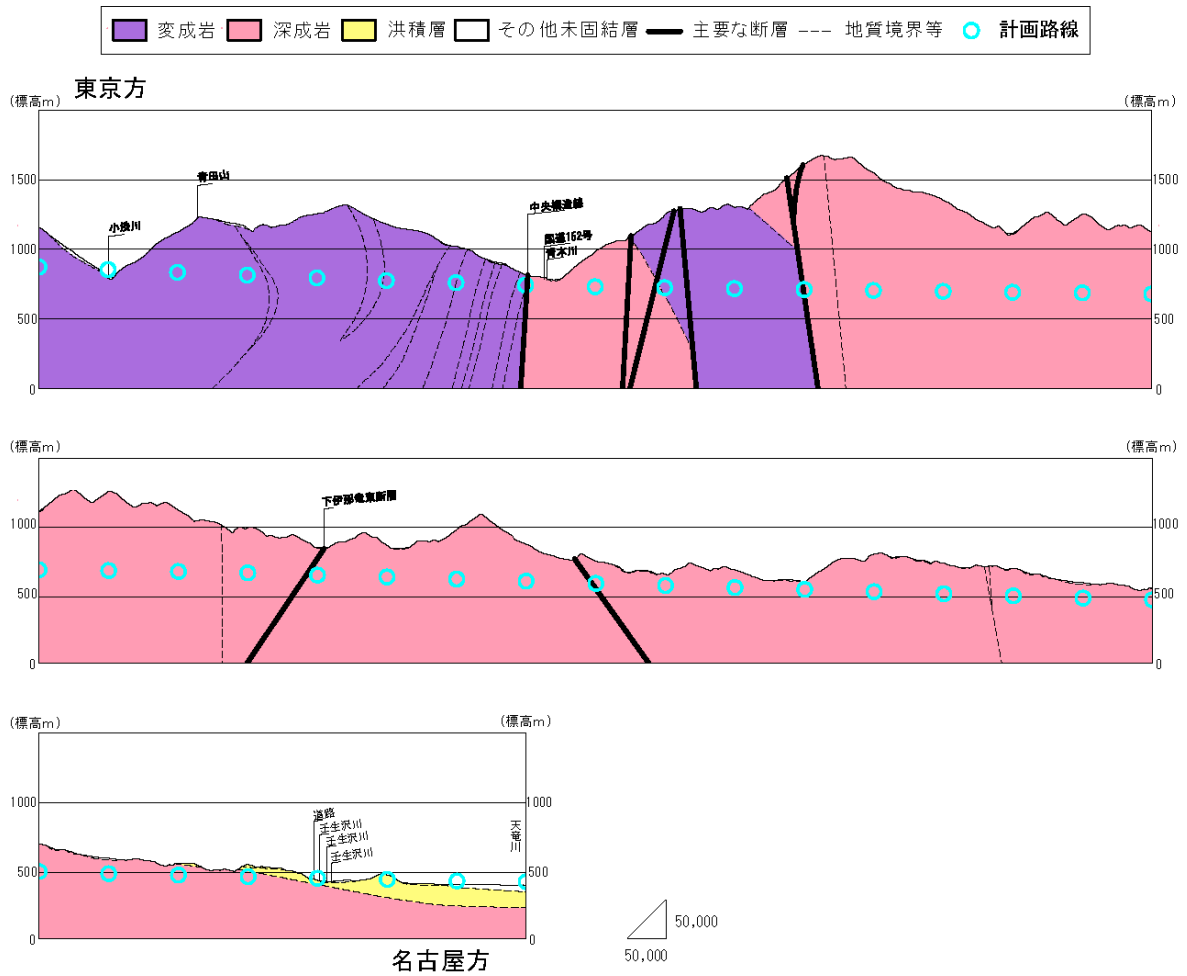
図 8-2-3-4(2) 地質縦断図 (小湊川から天竜川まで)
