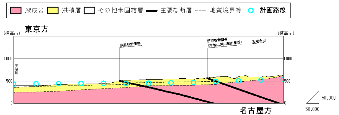
図 8-2-3-4(3) 地質縦断図 (天竜川から王竜寺川まで)
