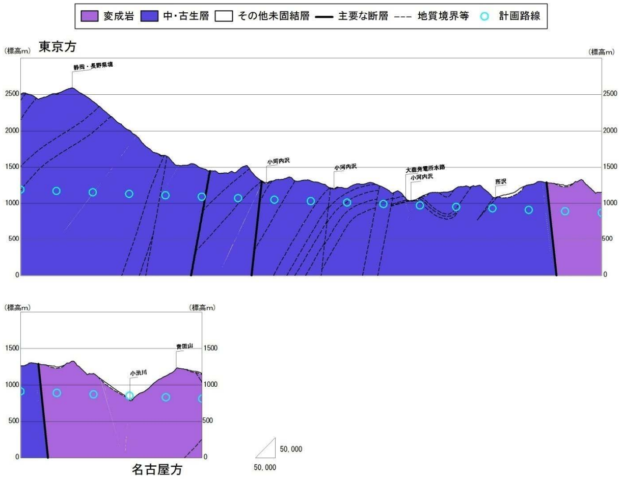
図 8-2-3-4(1) 地質縦断図 (静岡県境から小渋川まで)
