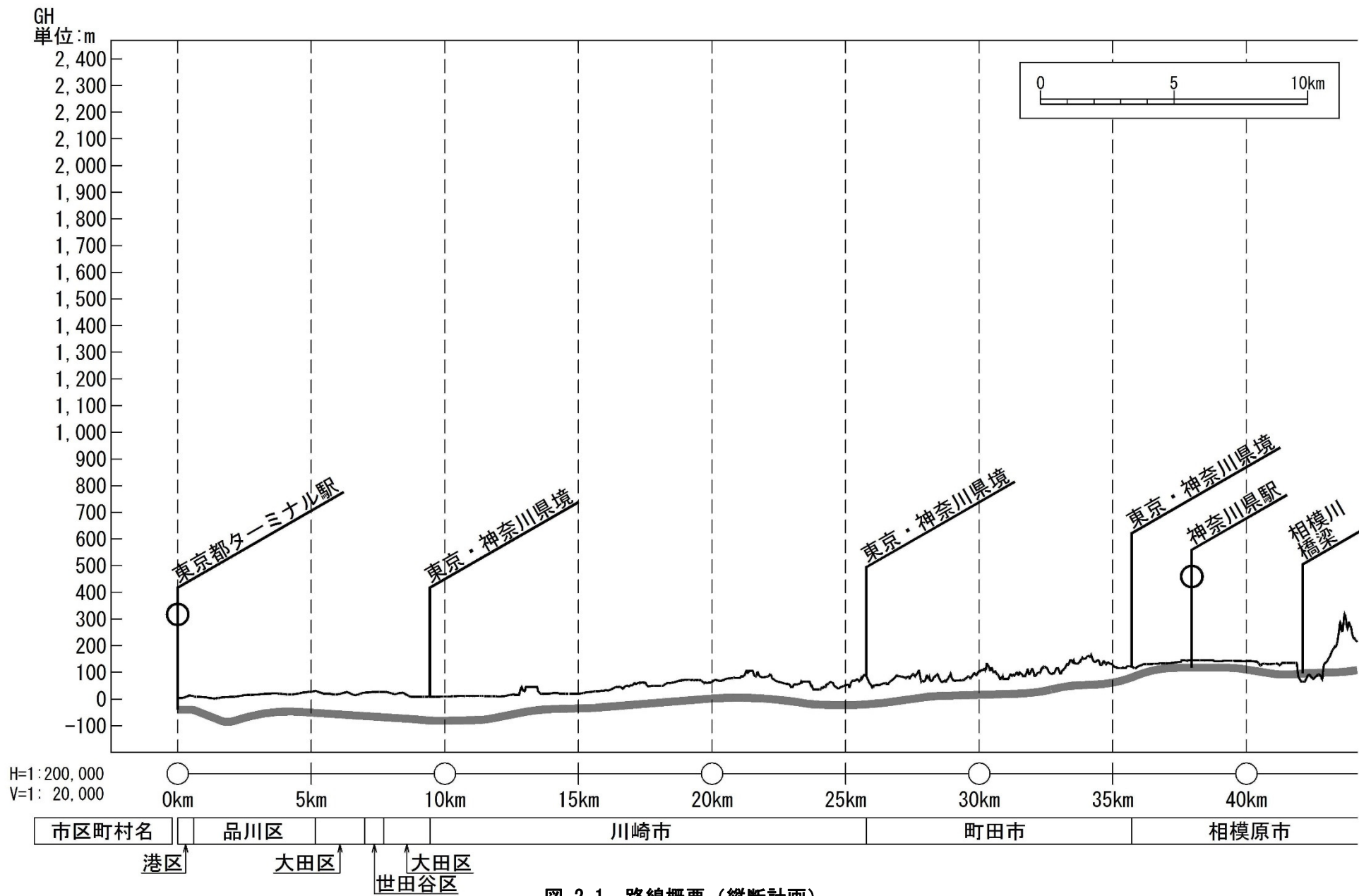
図 2-1 路線概要 (縦断計画)
