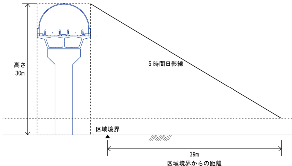
図 8-3-4-1 日影断面予測図(高架橋)
