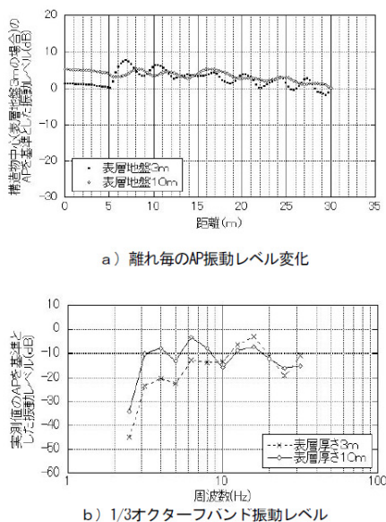
図-32 表層地盤の厚さが異なる場合の予測値の比較
