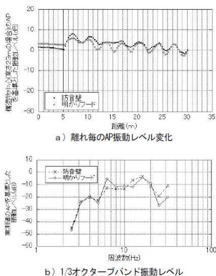
図-31 防音壁と明かりフードの予測値の比較
