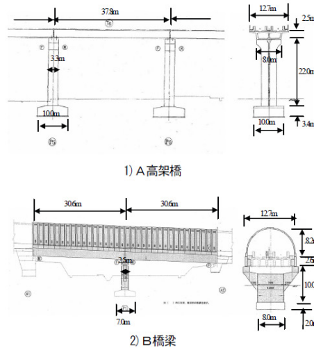
図-2 測定対象構造物の概要
