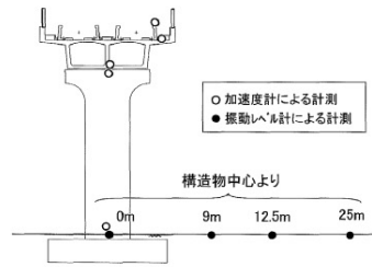
図-3 振動の測定位置
