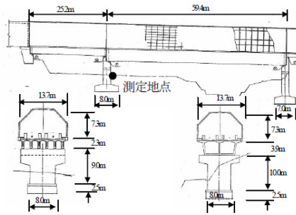
図-18 C橋梁の概要
