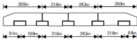
図-4 試験車両の概要
