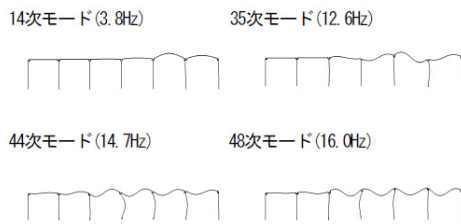
図-21 A高架橋の卓越振動モード(鉛直方向)
