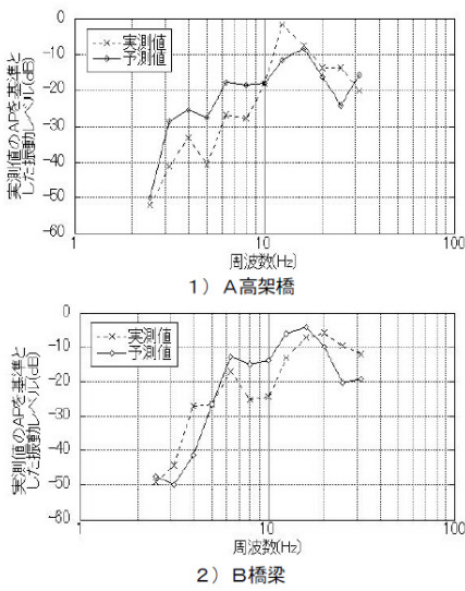
図-27 500km/h走行時の沿線地盤振動(9m離れ)に関する予測値・実測値比較
