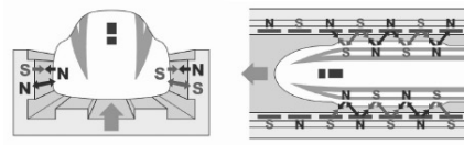
図-1 超高速鉄道の推進・浮上の原理
