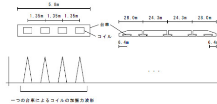
一つの台車によるコイルの加振力波形
