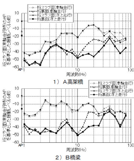
図-12 200km/h走行時の桁スラブ面、桁裏面における1/3オクターブバンド振動レベル(車輪走行時と浮上走行時の比較)
