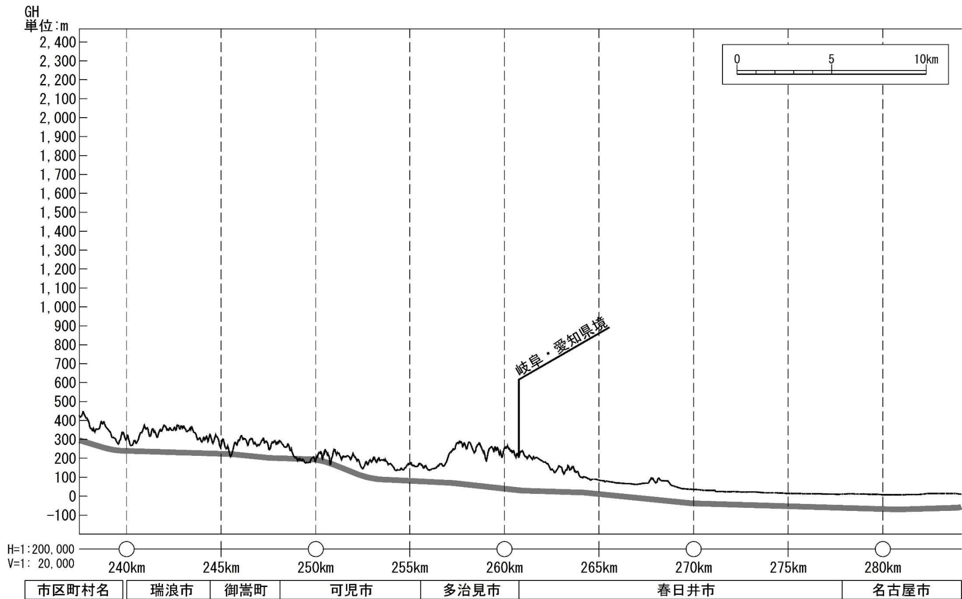
図 2-1(7) 路線概要 (縦断計画)
