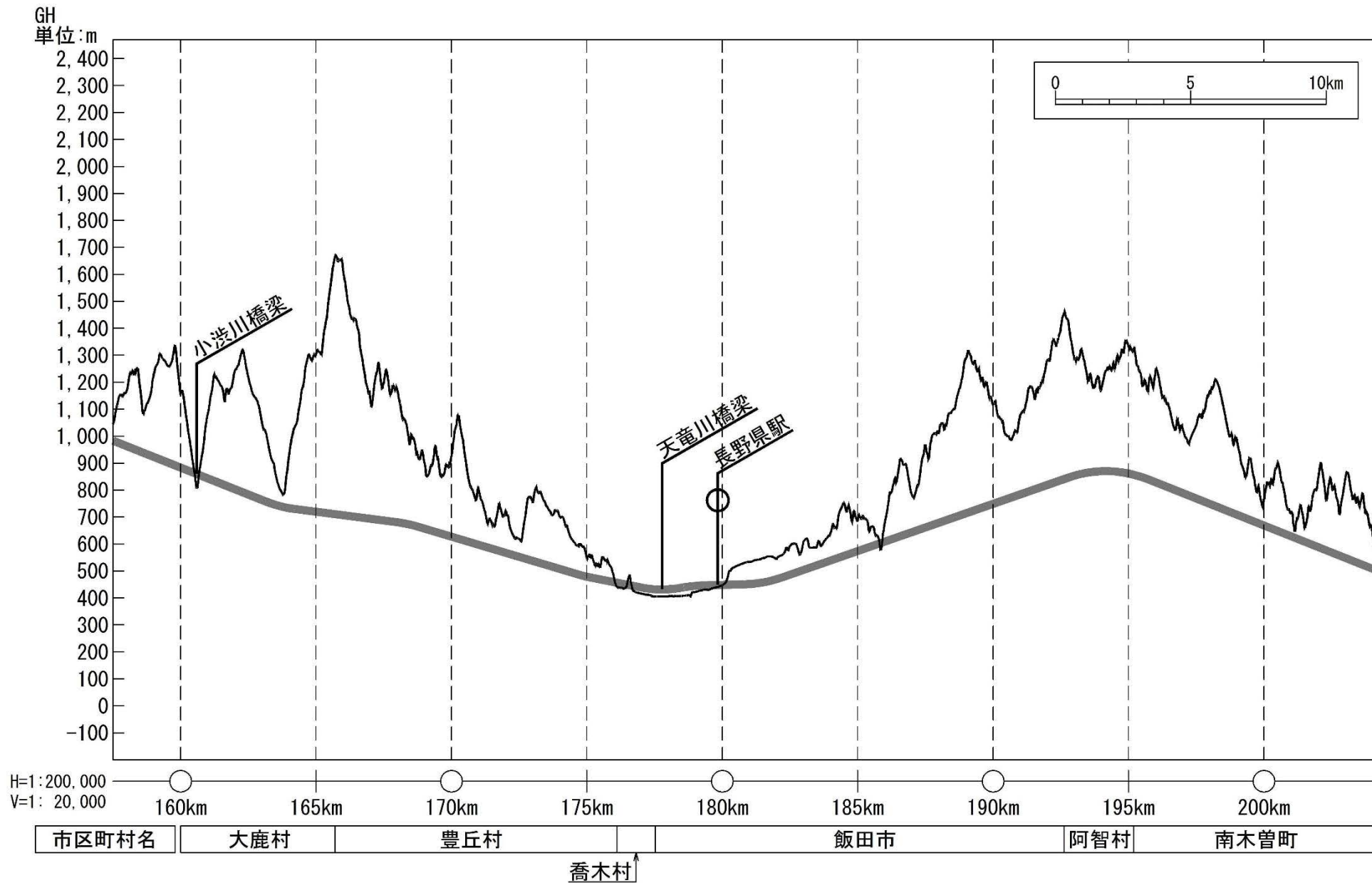
图 2-1(5) 路線概要 (縦断計画)
