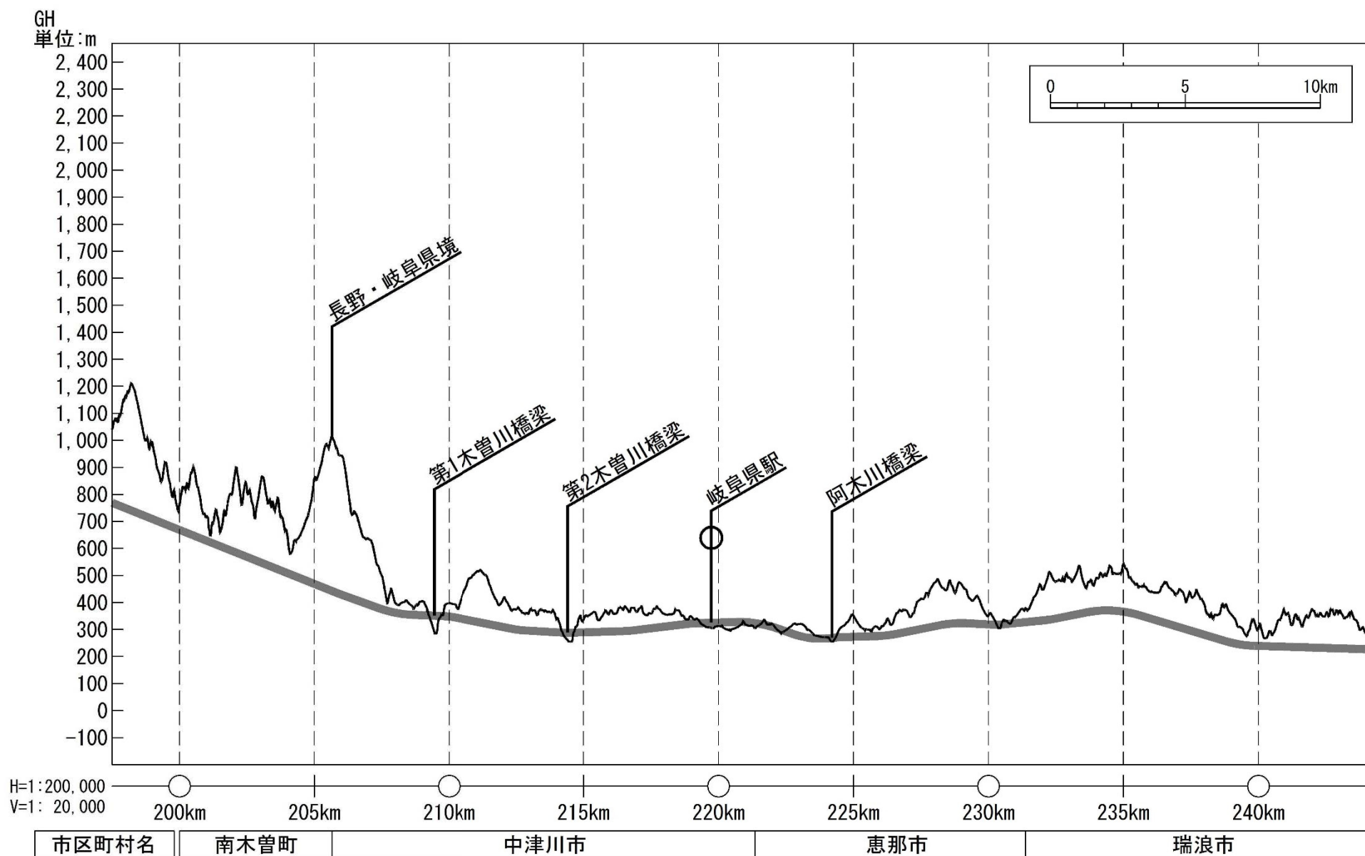
図 2-1(6) 路線概要(縦断計画)
