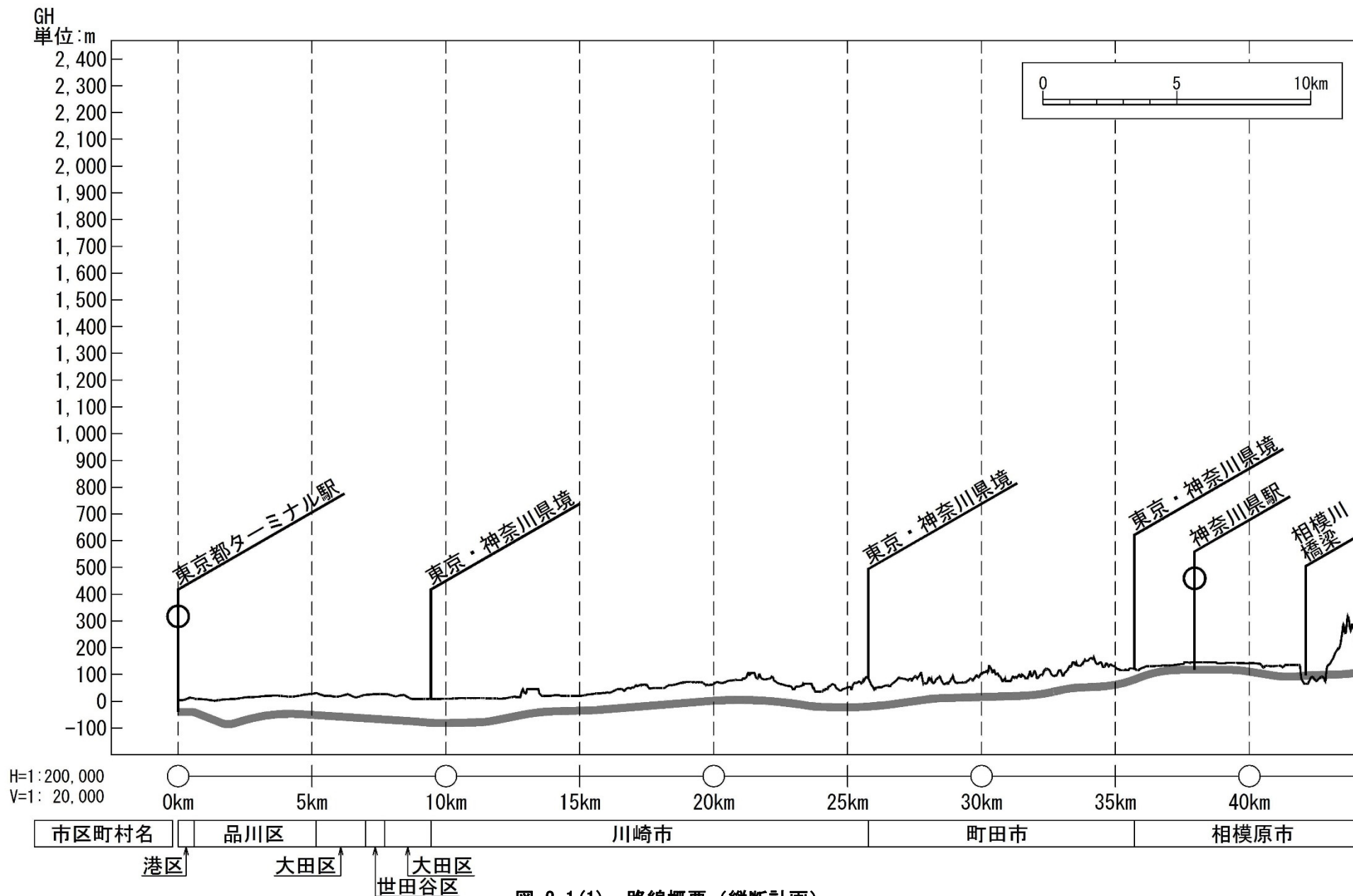
図 2-1(1) 路線概要 (縦断計画)
