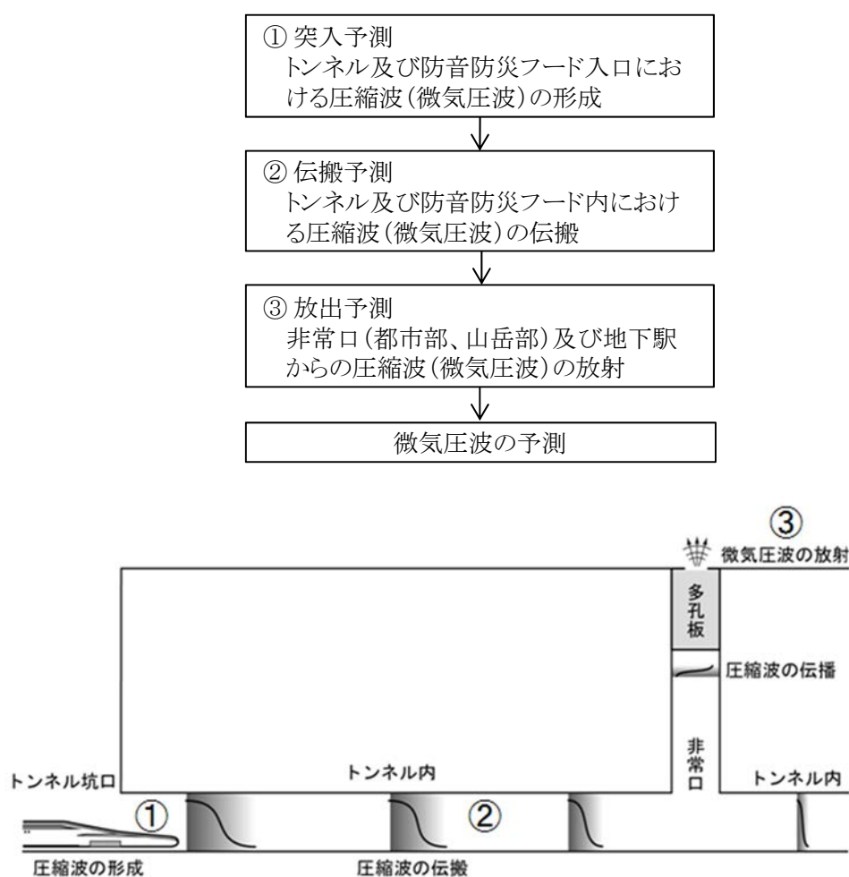
図 8-1-4-2 非常口（都市部、山岳部）及び地下駅から発生する微気圧波の予測フロー
