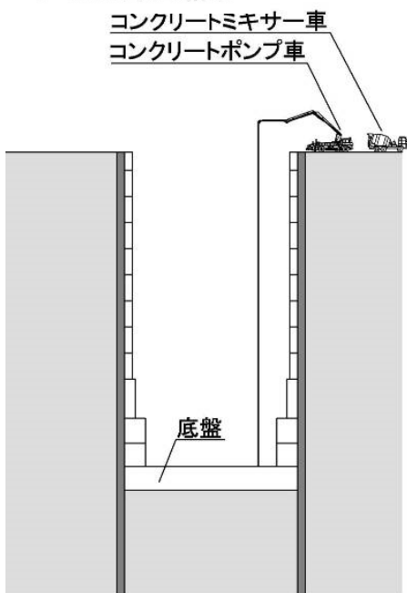
図 3-4-6-21 非常口の施工概要（RC 地中連続壁工法の場合）
