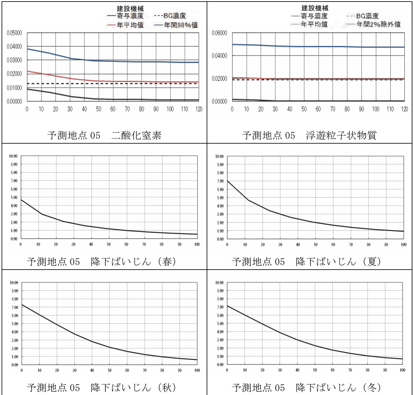
図 1-4-2(5) 建設機械の稼働による大気質の距離減衰の状況
