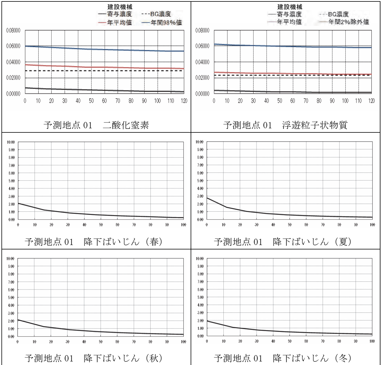
図 1-4-2(1) 建設機械の稼働による大気質の距離減衰の状況
