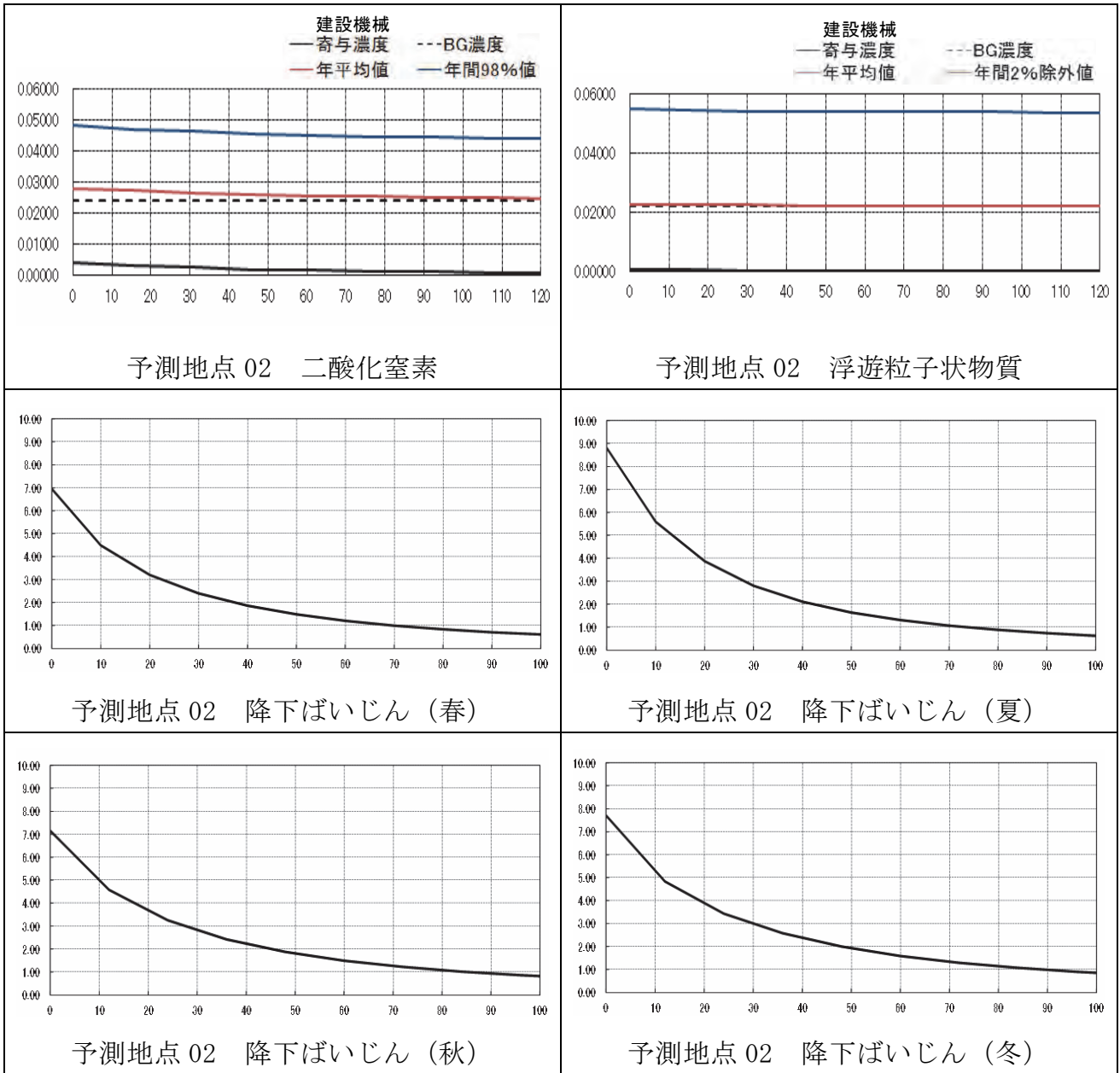
図 1-4-2(2) 建設機械の稼働による大気質の距離減衰の状況
