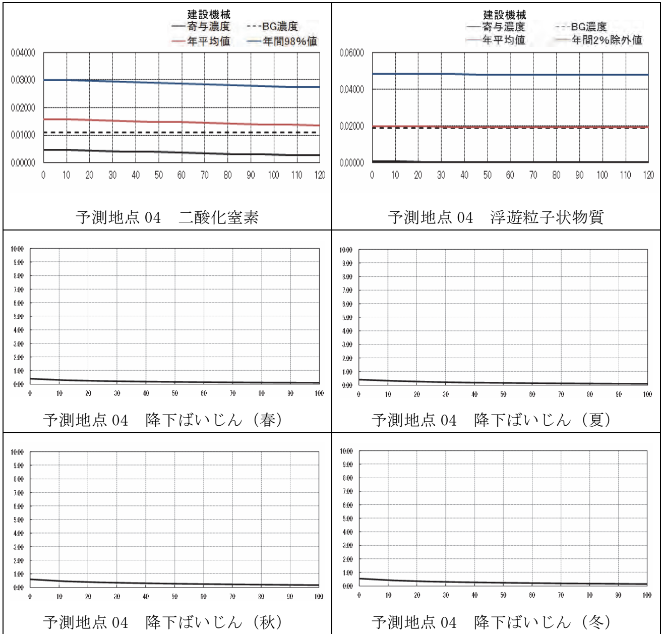
図 1-4-2(4) 建設機械の稼働による大気質の距離減衰の状況
