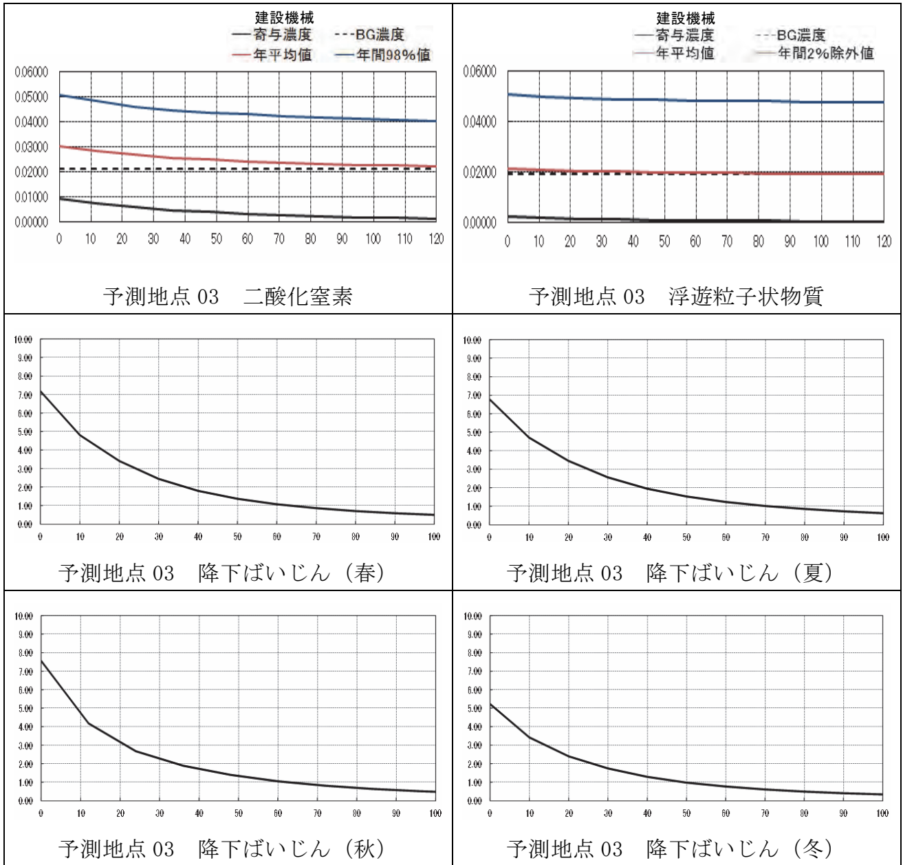
図 1-4-2(3) 建設機械の稼働による大気質の距離減衰の状況
