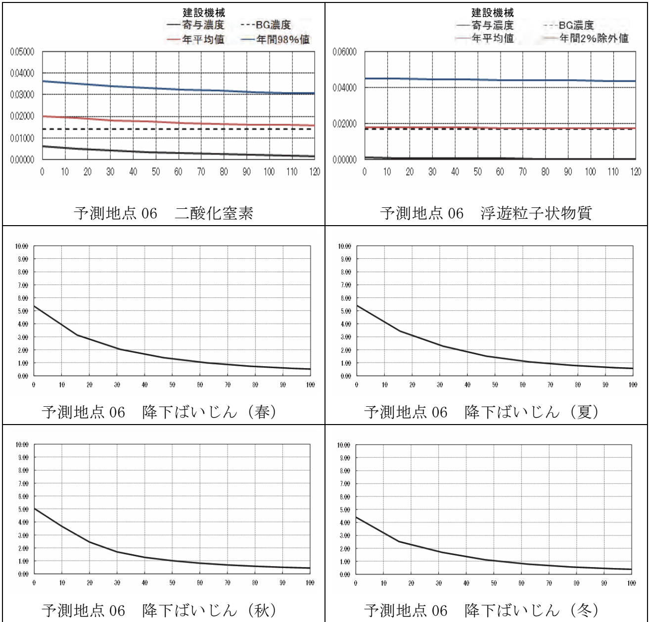
図 1-4-2(6) 建設機械の稼働による大気質の距離減衰の状況
