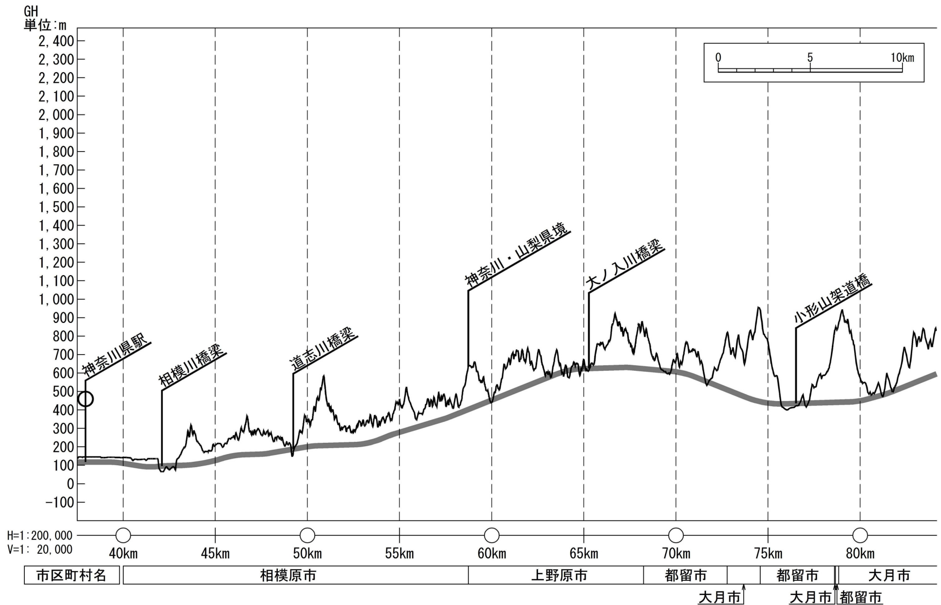
図 2-1 (2) 路線概要 (縦断計画)
