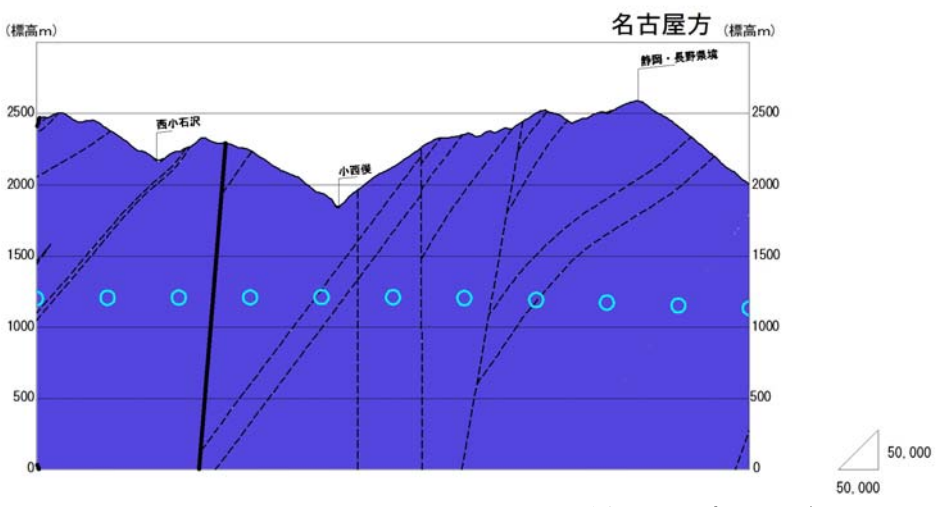
図 8-2-3-3 地質縦断図 (赤石山脈)
