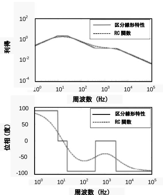
図 A1 誘導電界の重み付けに対する振幅応答と位相応答
