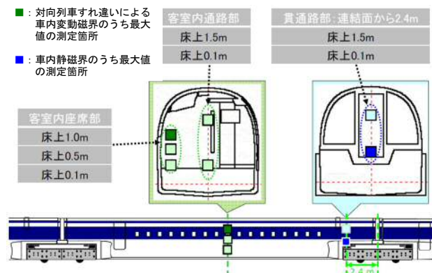
図 13-5-6 車内の磁界の測定箇所
