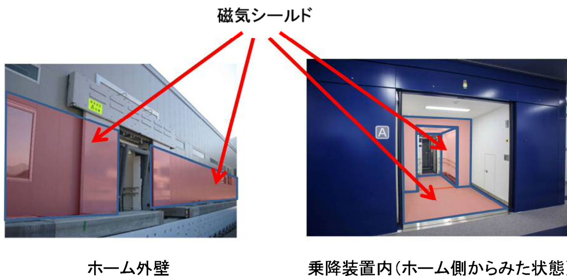
図 13-5-2 ホームへの磁気シールド設置の概念図
