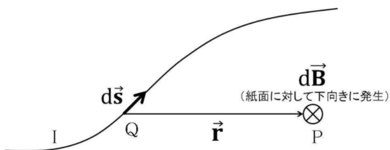
図 13-7-1 ビオ・サバールの法則概念図
