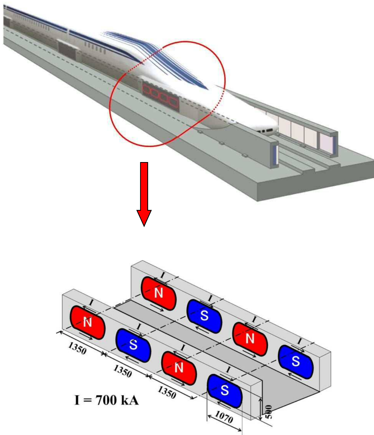
図 13-7-2 超電導磁石を拡大した概略図（磁界の算出にあたっての前提条件）
