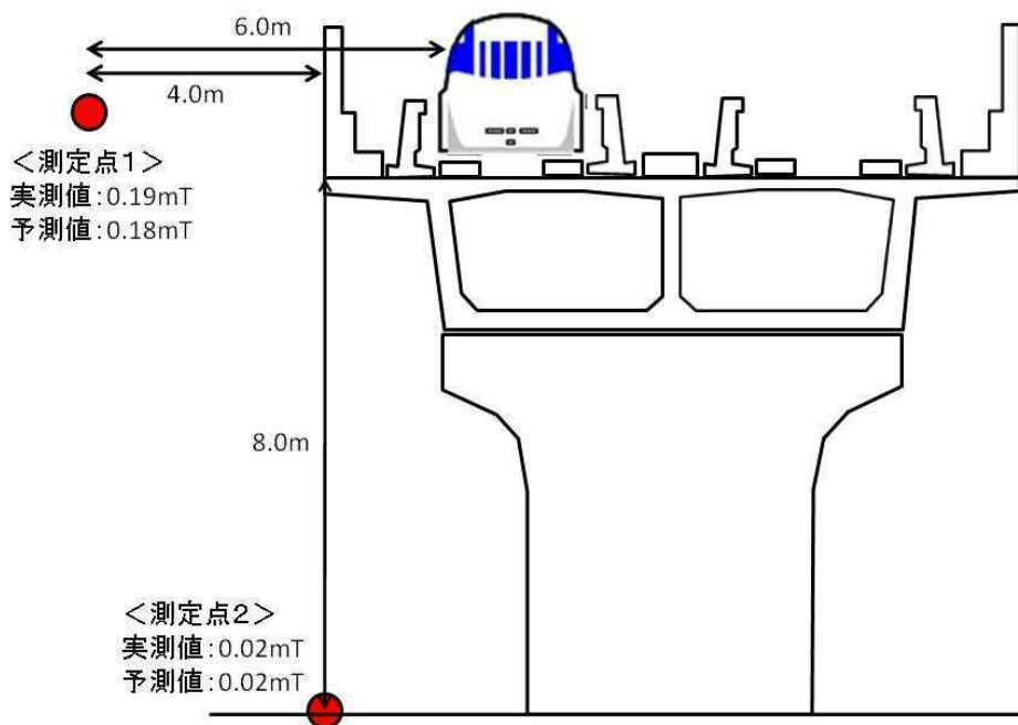
図 13-7-3 山梨リニア実験線における実測値と予測値の比較
