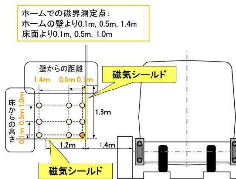
図 13-5-7 ホーム上の磁界の測定箇所
