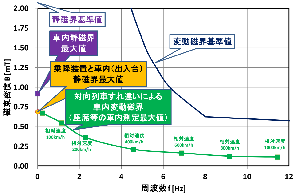
図 13-5-5 車内及び乗降装置と車内（出入台）の磁界の測定結果
