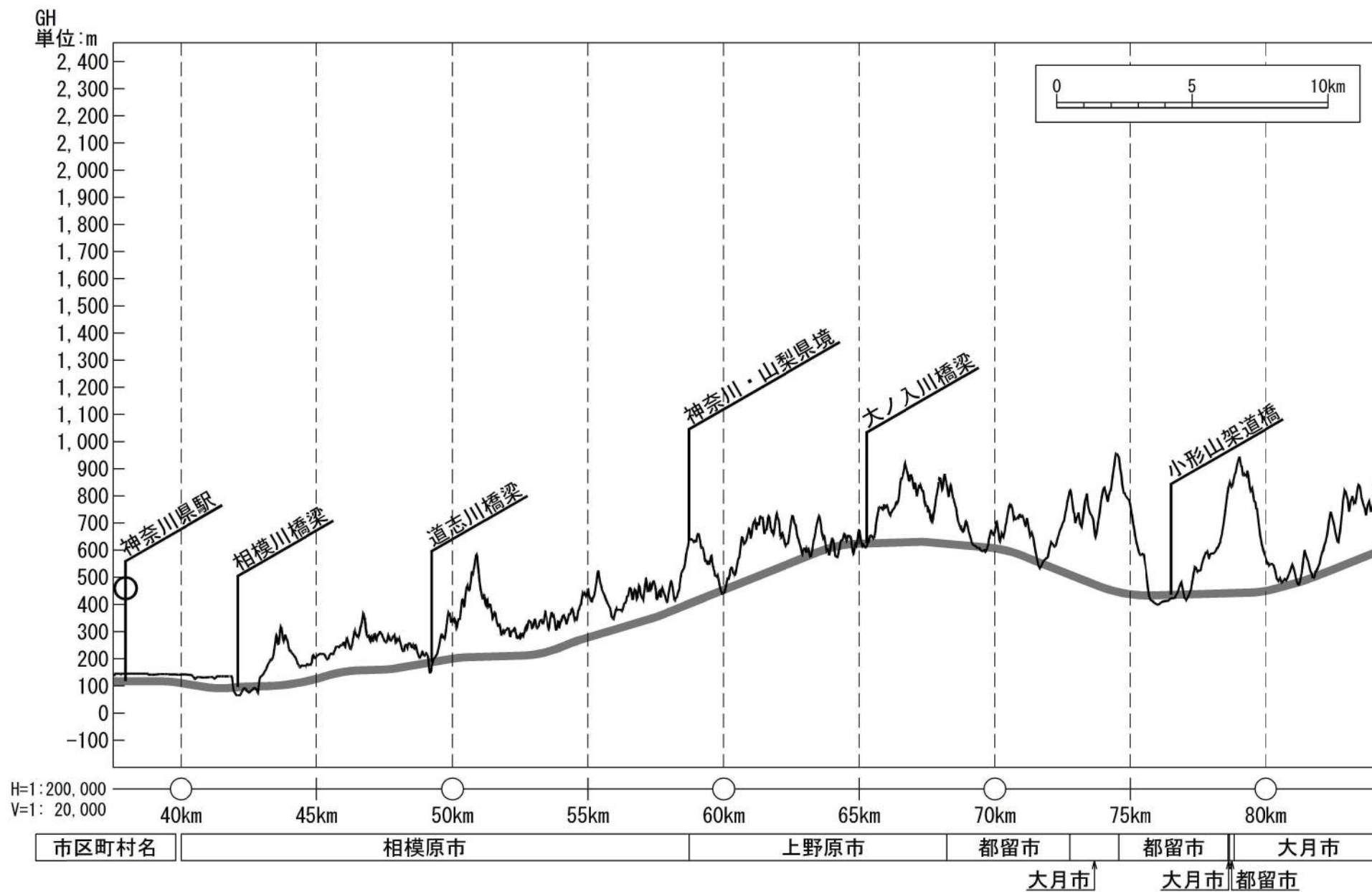
図 2-1(2) 路線概要 (縦断計画)
