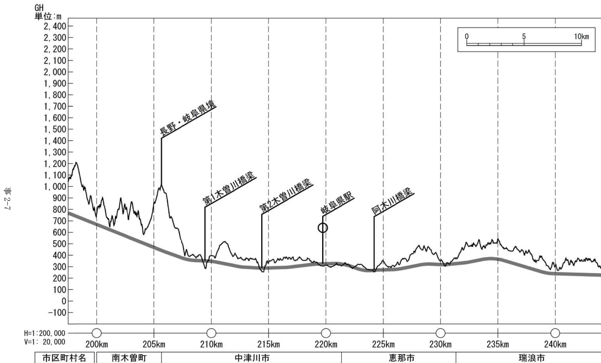
図 2-1(6) 路線概要(縦断計画)
