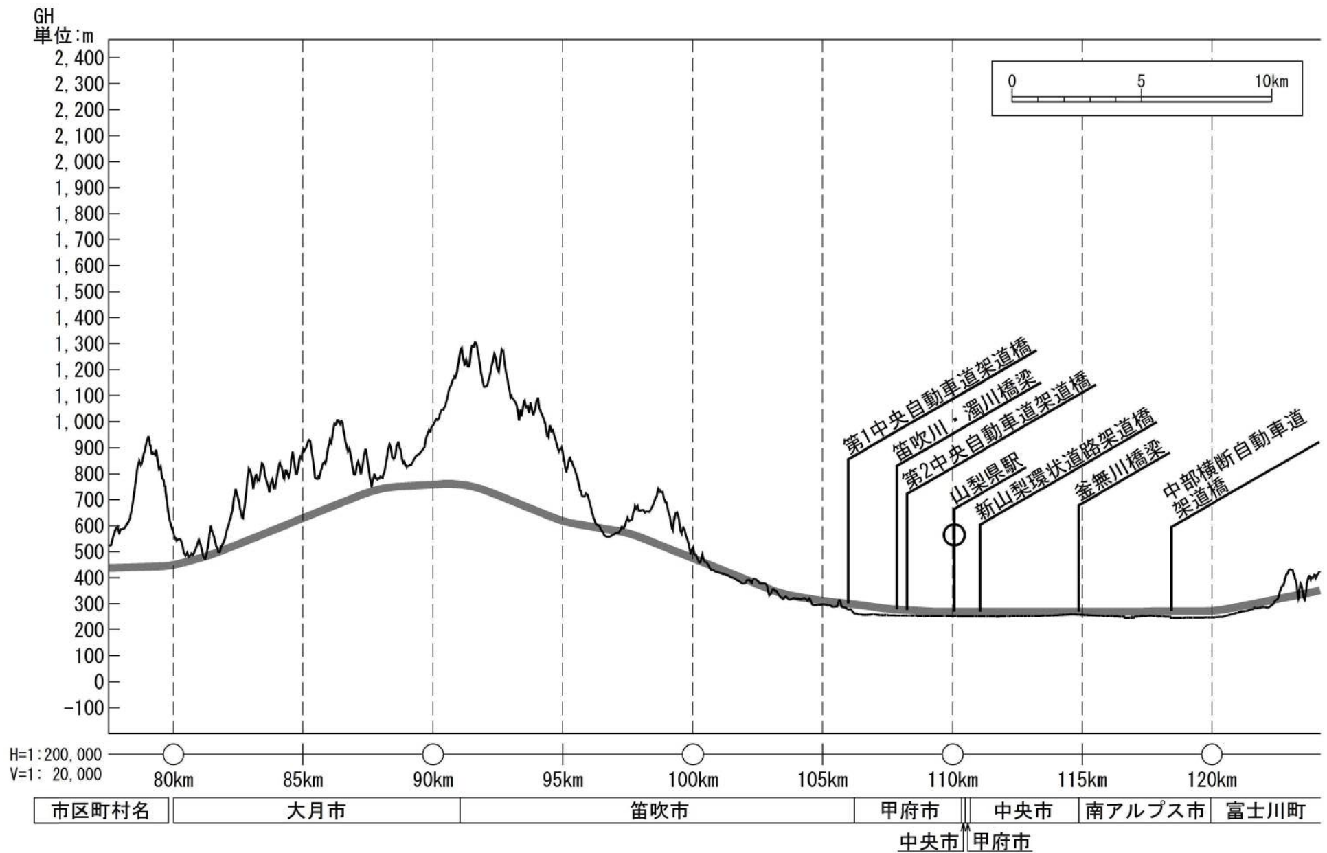
図 2-1(3) 路線概要 (縦断計画)
