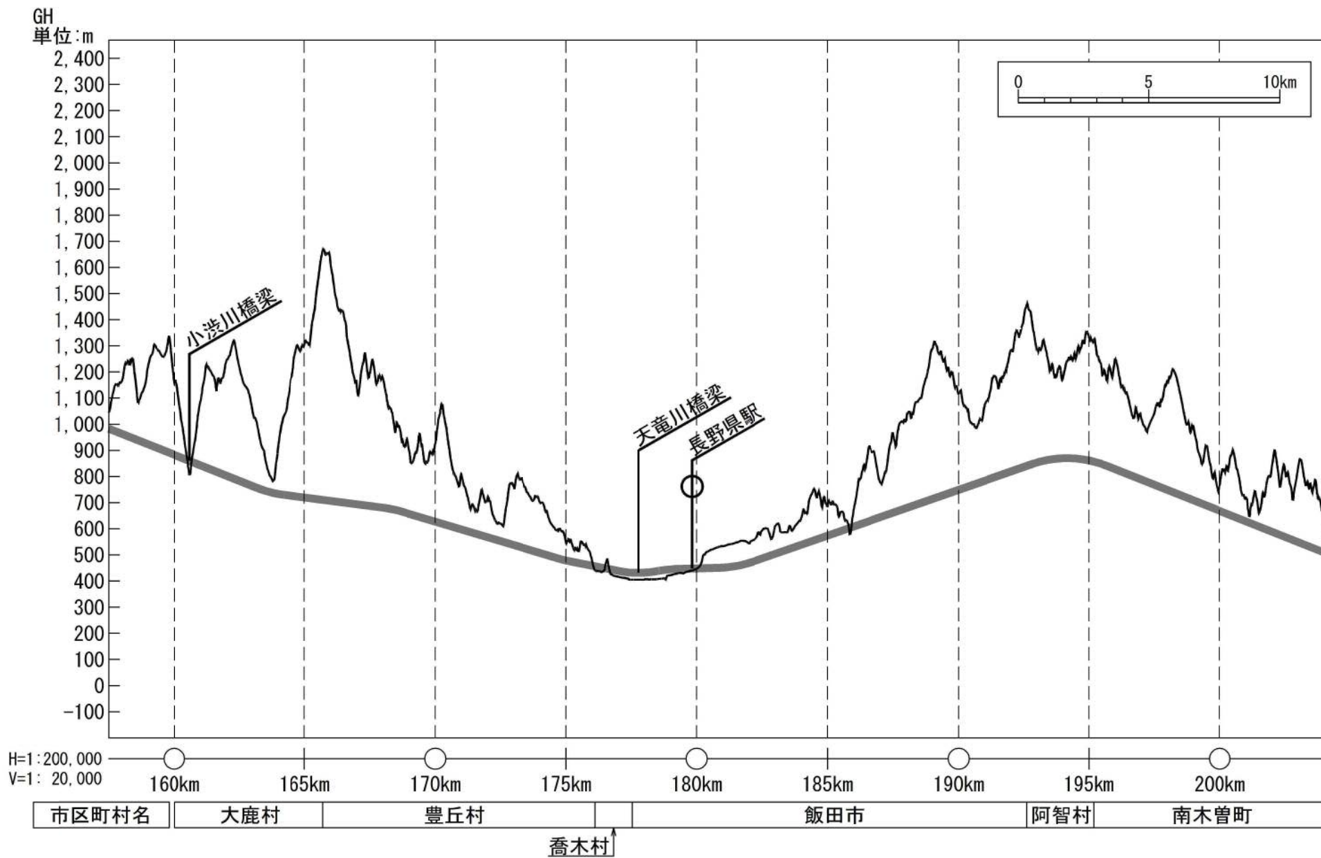
図 2-1 (5) 路線概要 (縦断計画)
