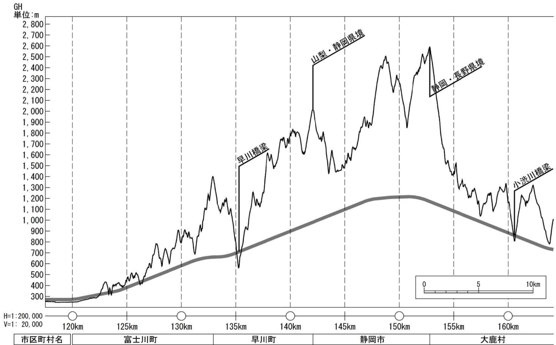
図 2-1(4) 路線概要 (縦断計画)
