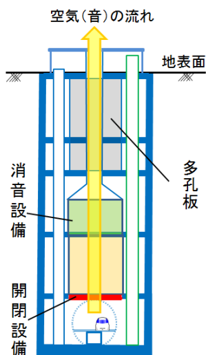
図 2-12-1-1 開閉設備の配置
