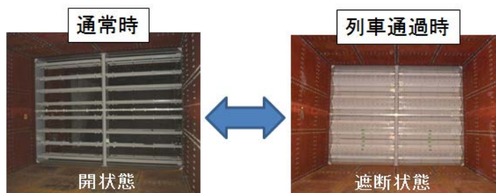
図 2-12-1-2 開閉設備の開閉状況のイメージ
